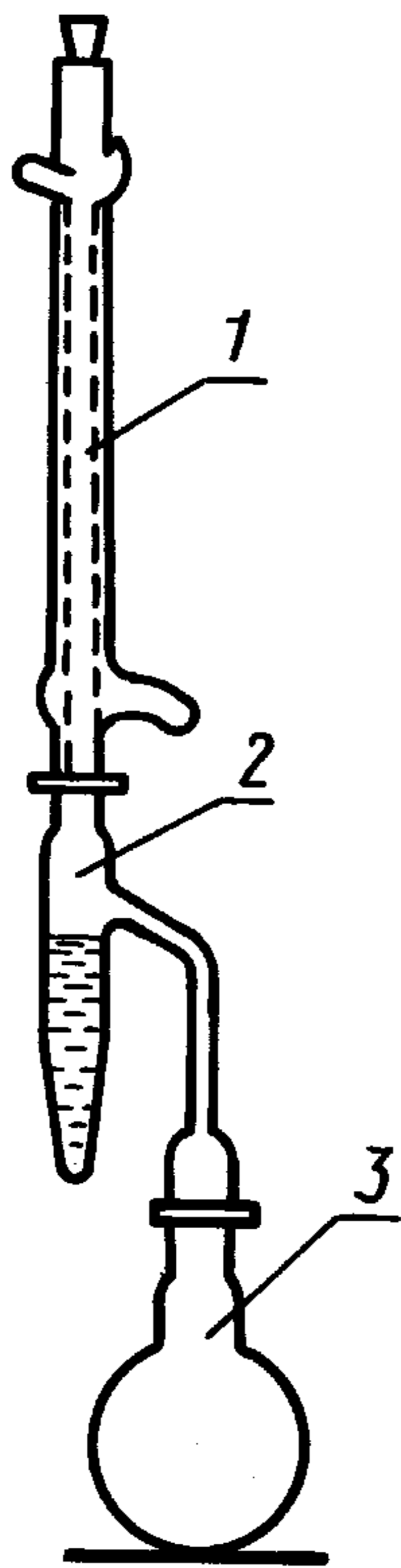
1 — холодильник с прямой трубкой; 2 — приемник-ловушка; 3 — круглодонная колба
