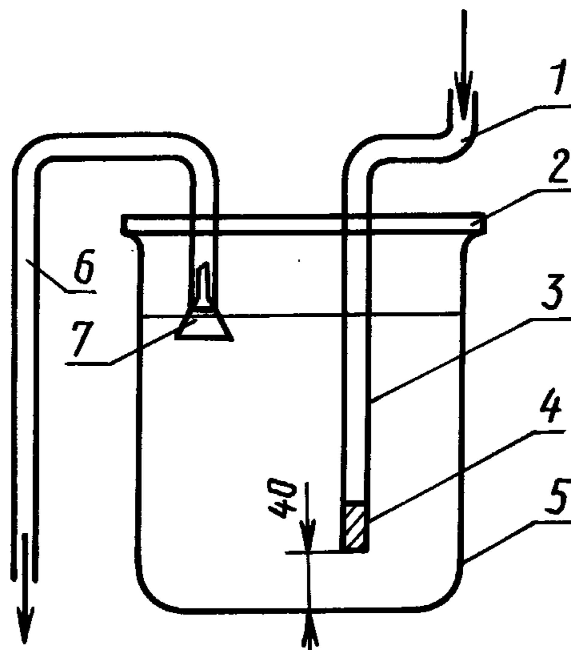
Установка для определения посторонних минеральных примесей
