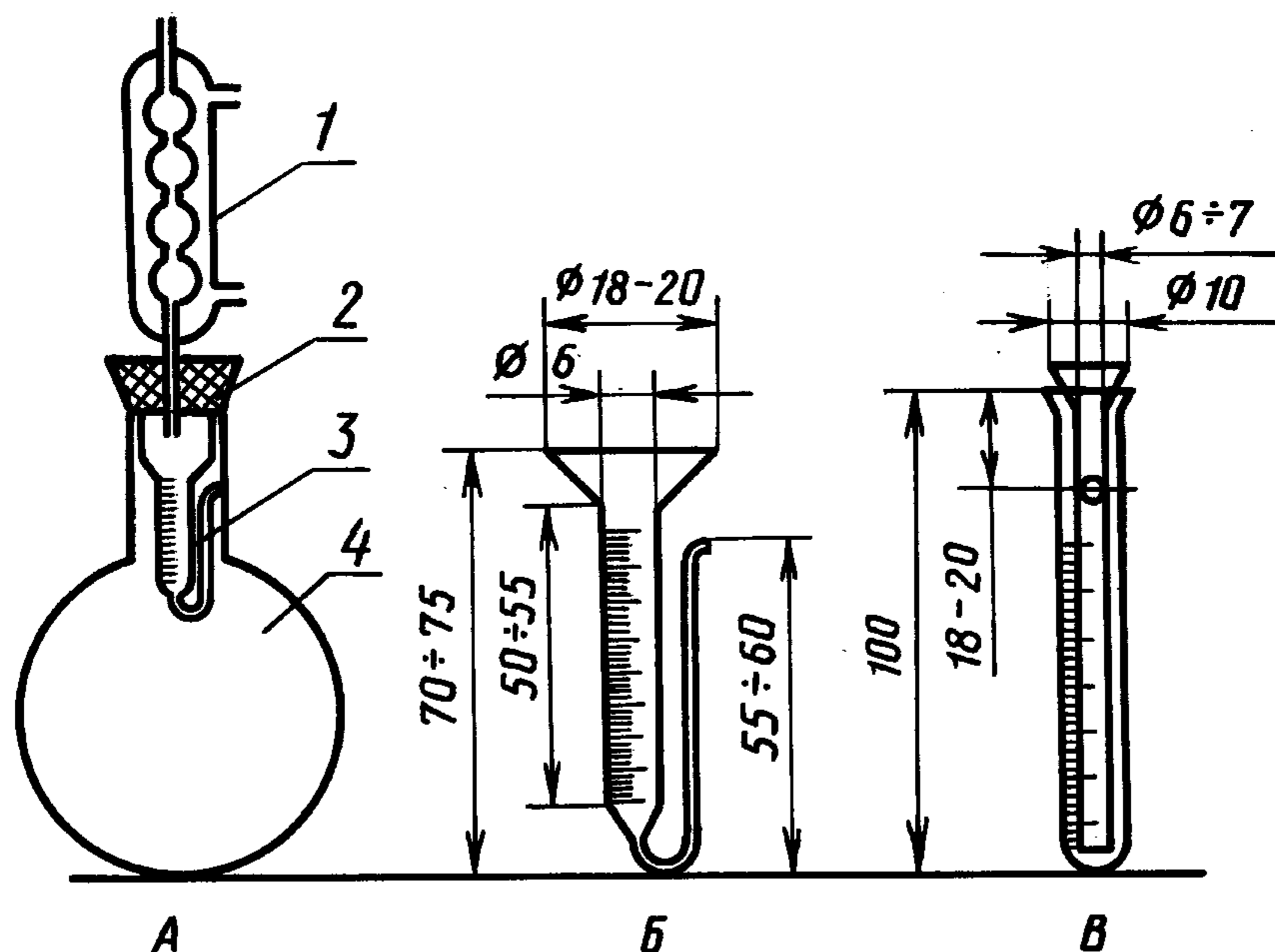
A — прибор для определения эфирных масел; B — приемник Гинзберга для эфирных масел плотностью менее 1 г/см 3 ; B' — приемник для эфирных масел плотностью более 1 г/см 3 1 — обратный холодильник; 2 — резиновая пробка; 3 — градуированный приемник; 4 — круглодонная колба
