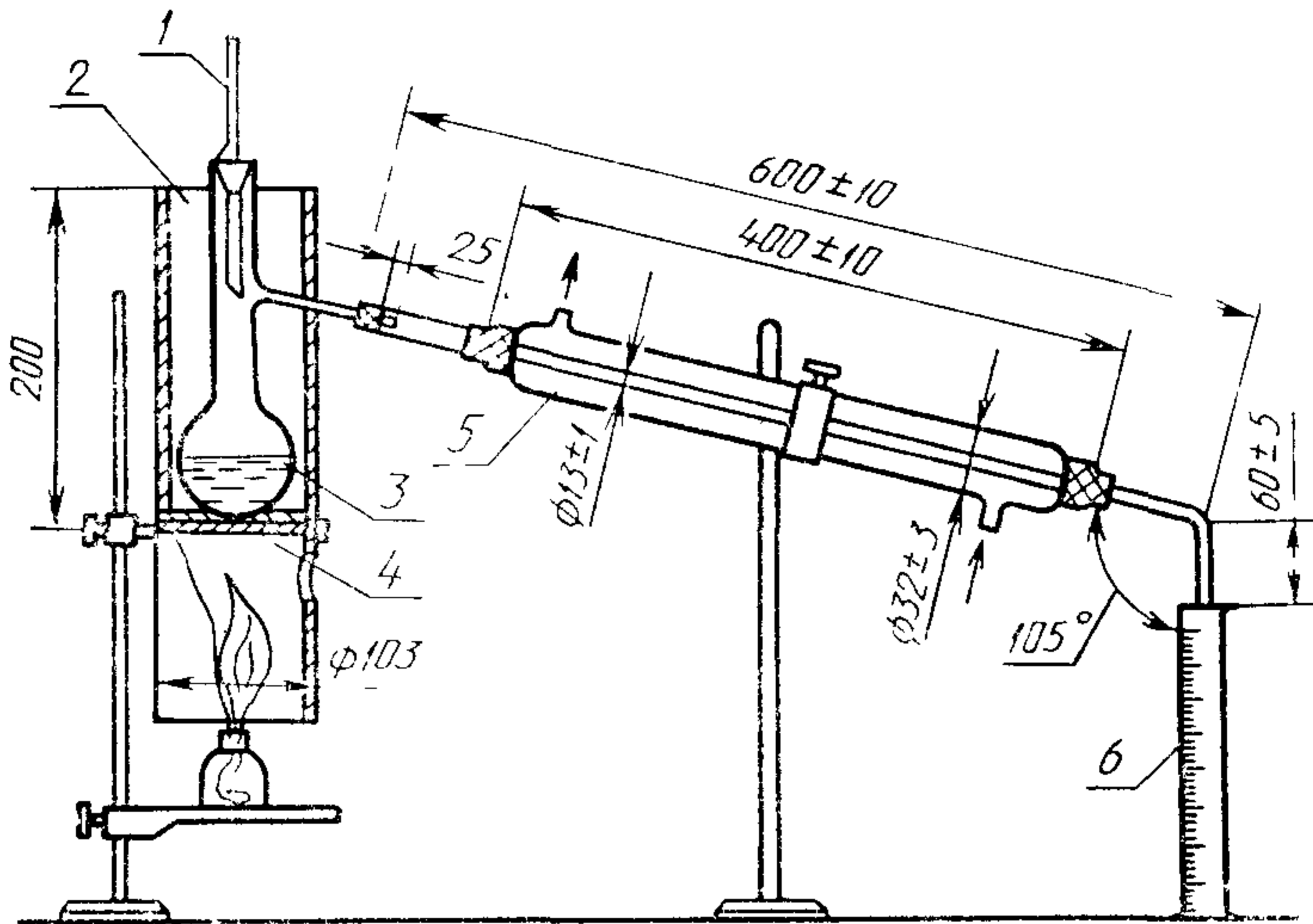
1—термометр; 2, 4—металлические кожухи; 3—колба; 5—холодильник; 6—цилиндр
