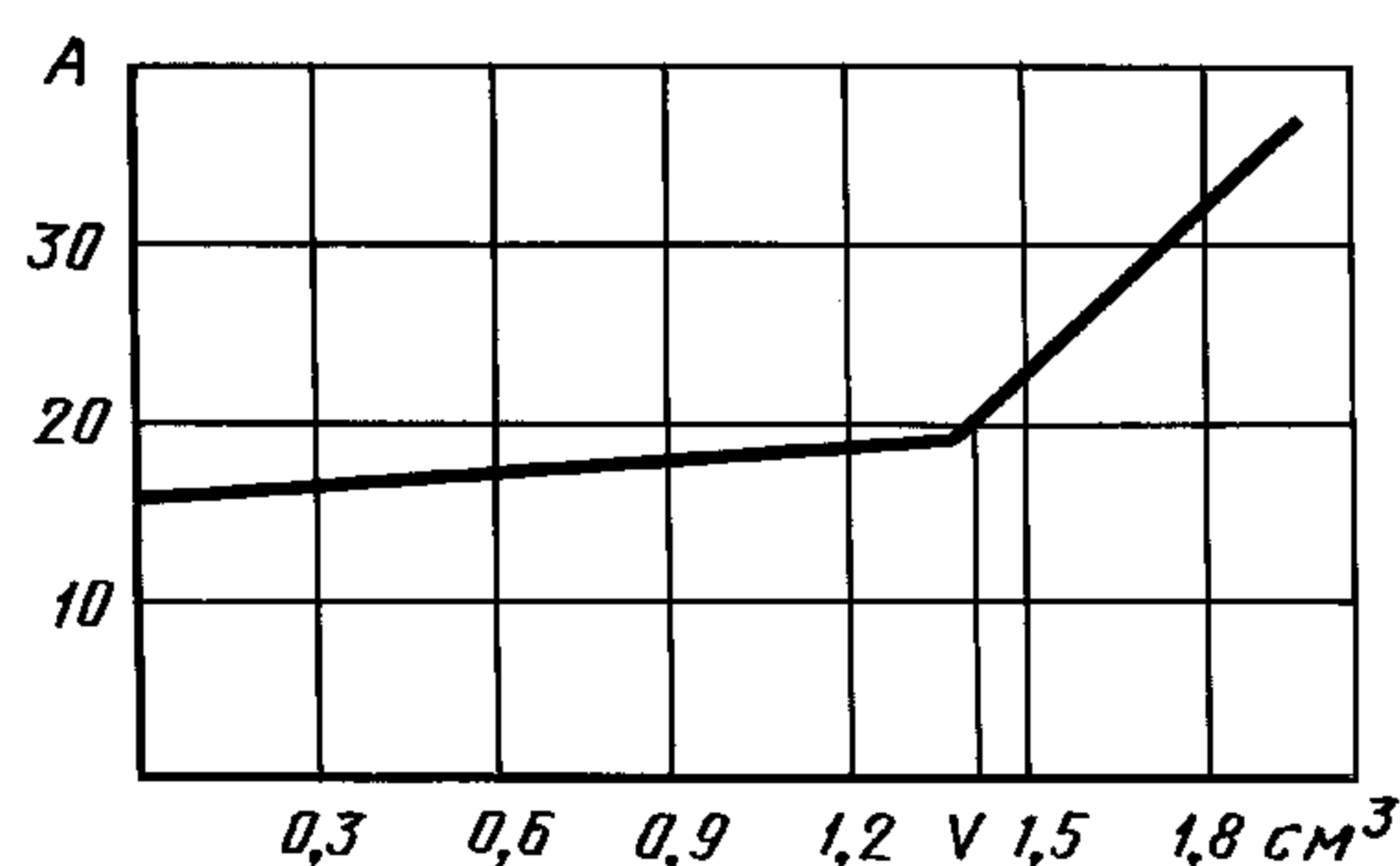
График титрования
