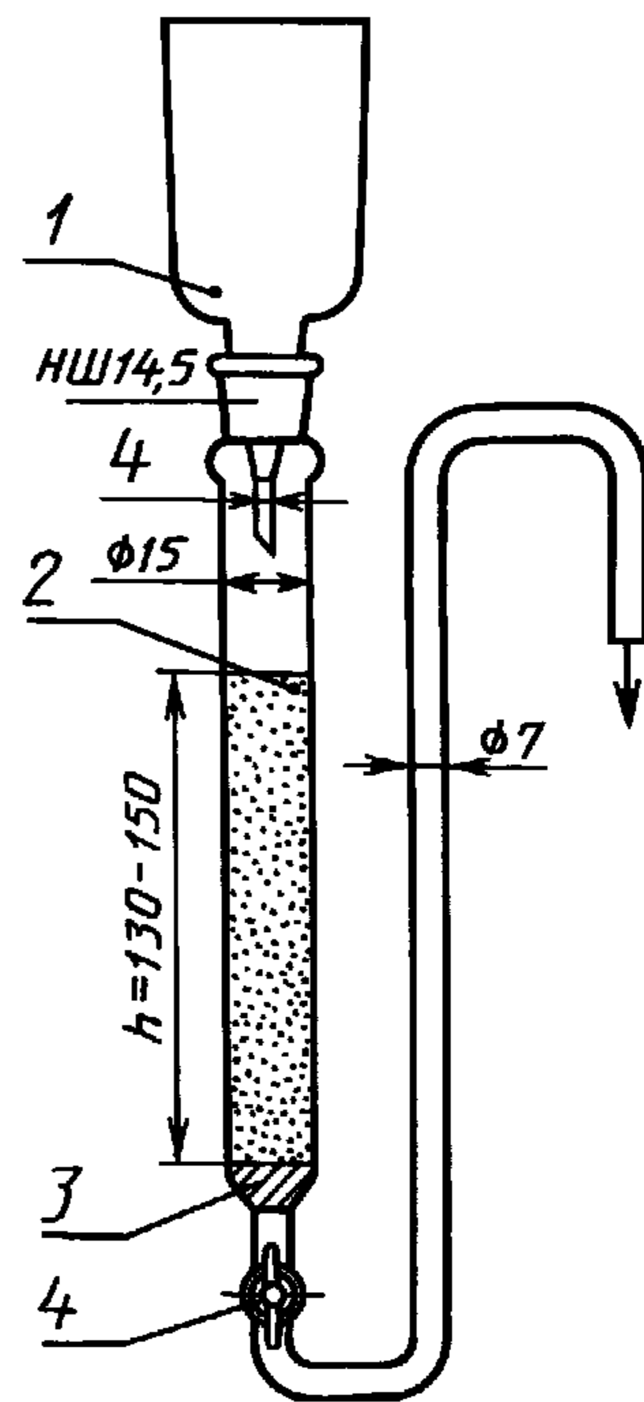
1 — резервуар вместимостью 50 см 3 ; 2 — колонка с кадмием; 3 — стекло-вата; 4 — кран
