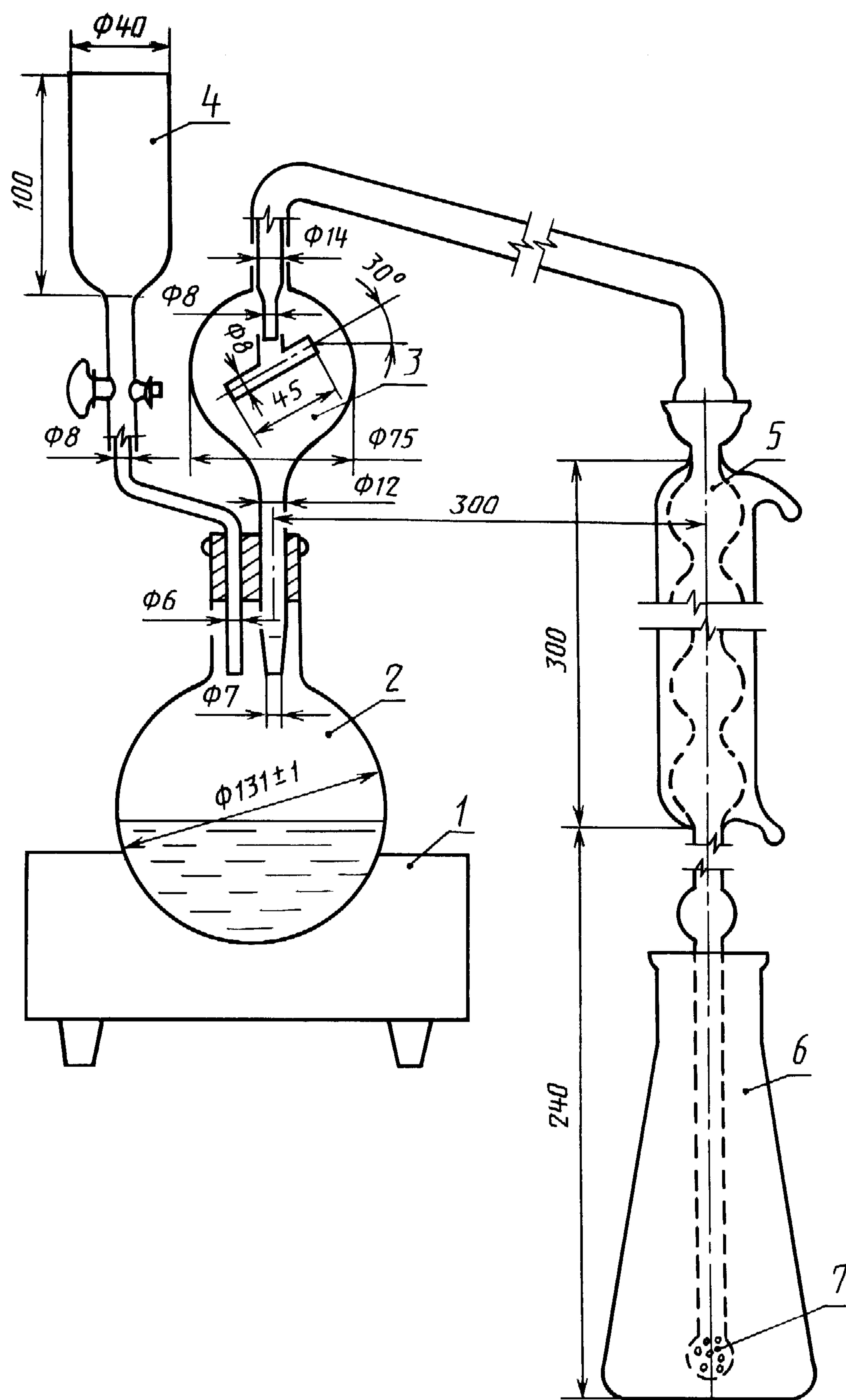
1 — колбонагреватель; 2 — реакционная колба вместимостью 0,5—1,0 дм 3 ; 3 — каплеуловитель; 4 — капельная воронка с краном; 5 — холодильник; 6 — приемник; 7 — барбатор
