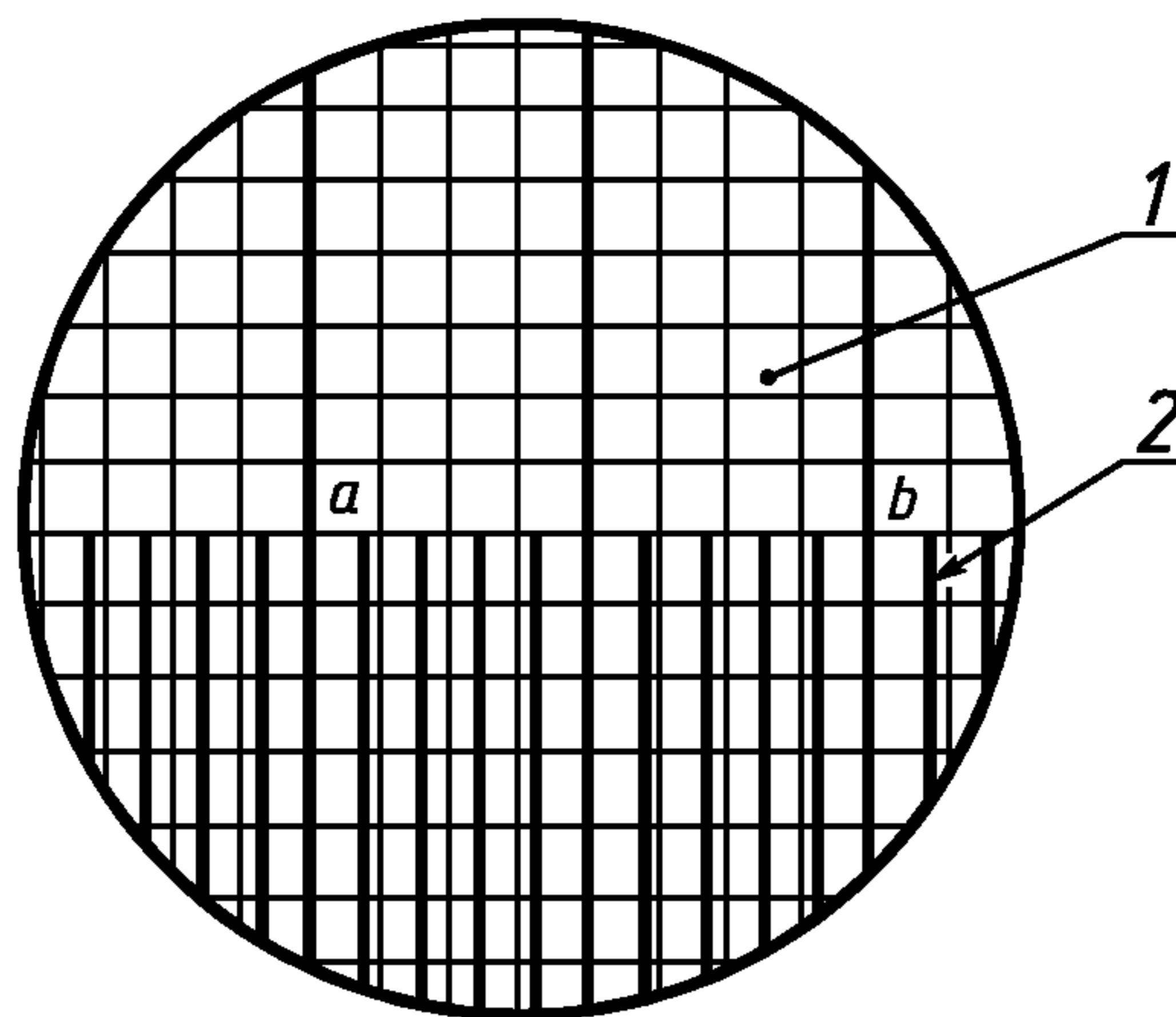
1 — сетка окулярного микрометра; 2 — шкала объекта-микрометра
