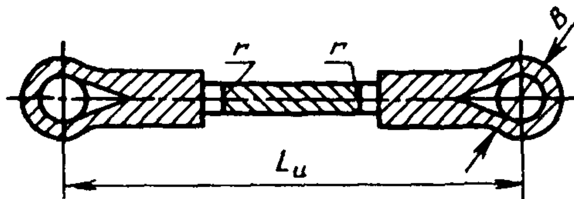
Машина для испытаний с кнехтами для нарощенных петель (отметка r расположена на расстоянии 150 мм от последнего витка сращивания)
