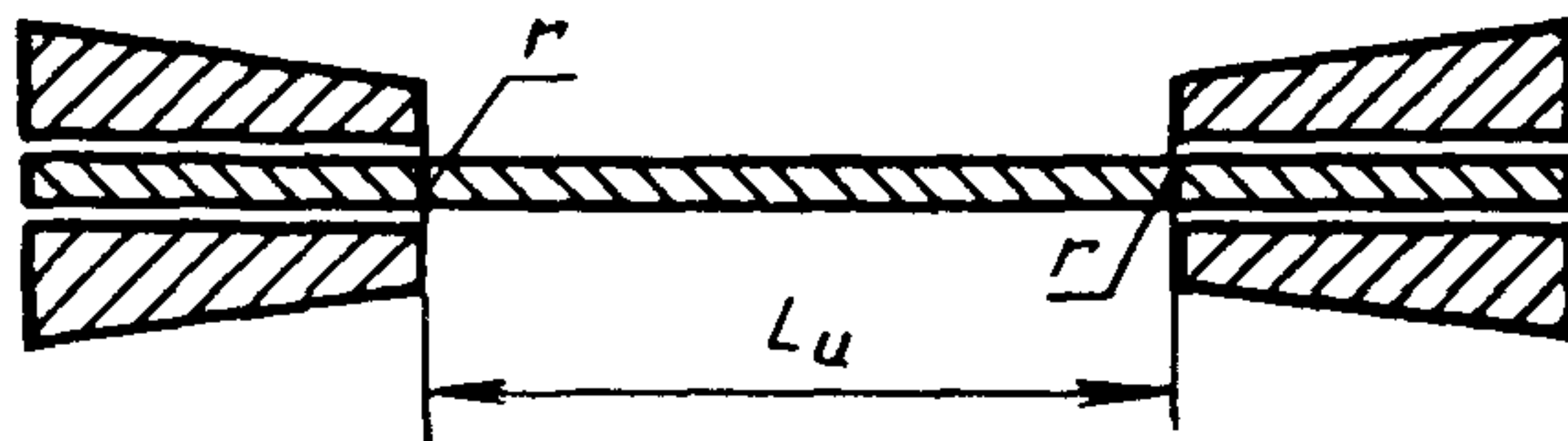
Машина для испытаний с кнехтами для нарощенных петель (отметка r расположена на расстоянии 150 мм от последнего витка сращивания)
