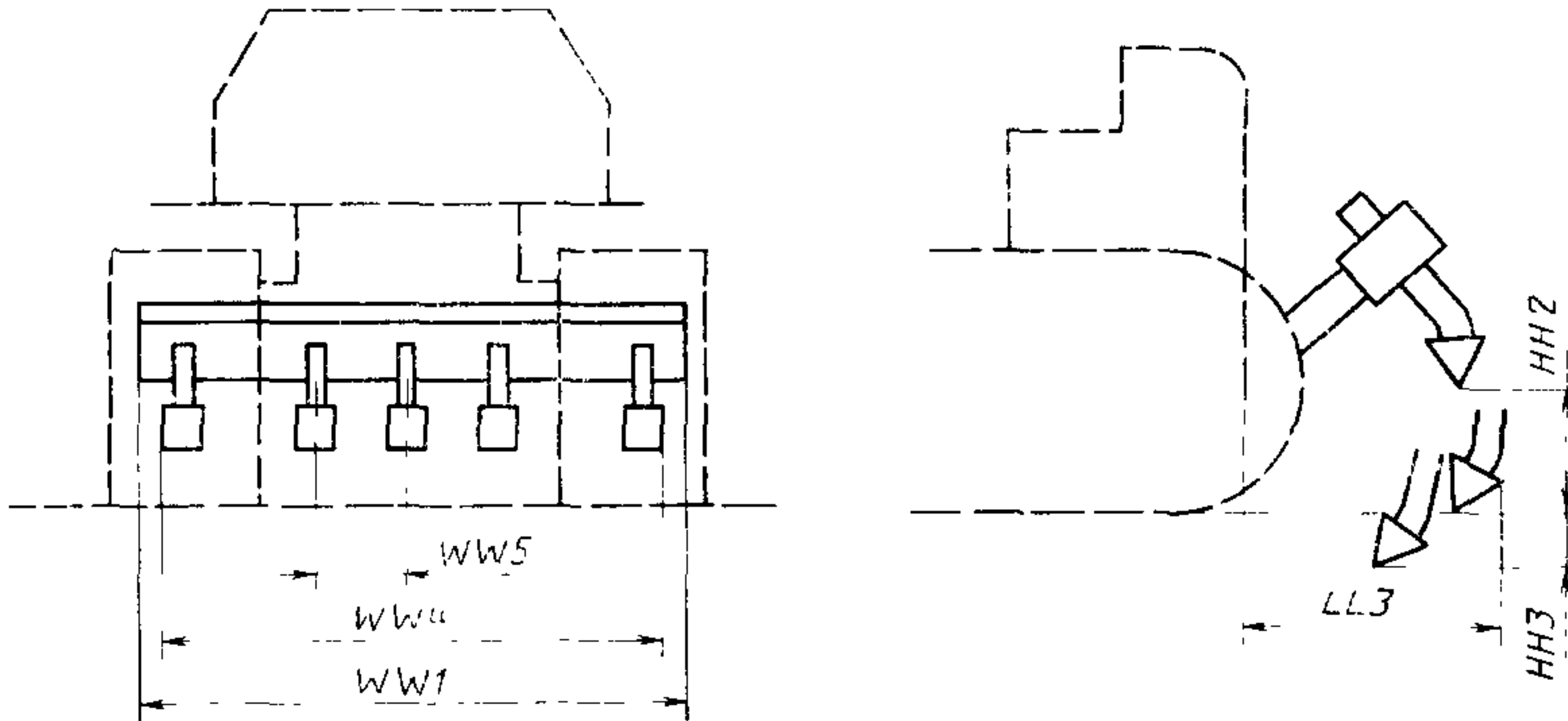
Черт. 18. Размеры рыхлителя
