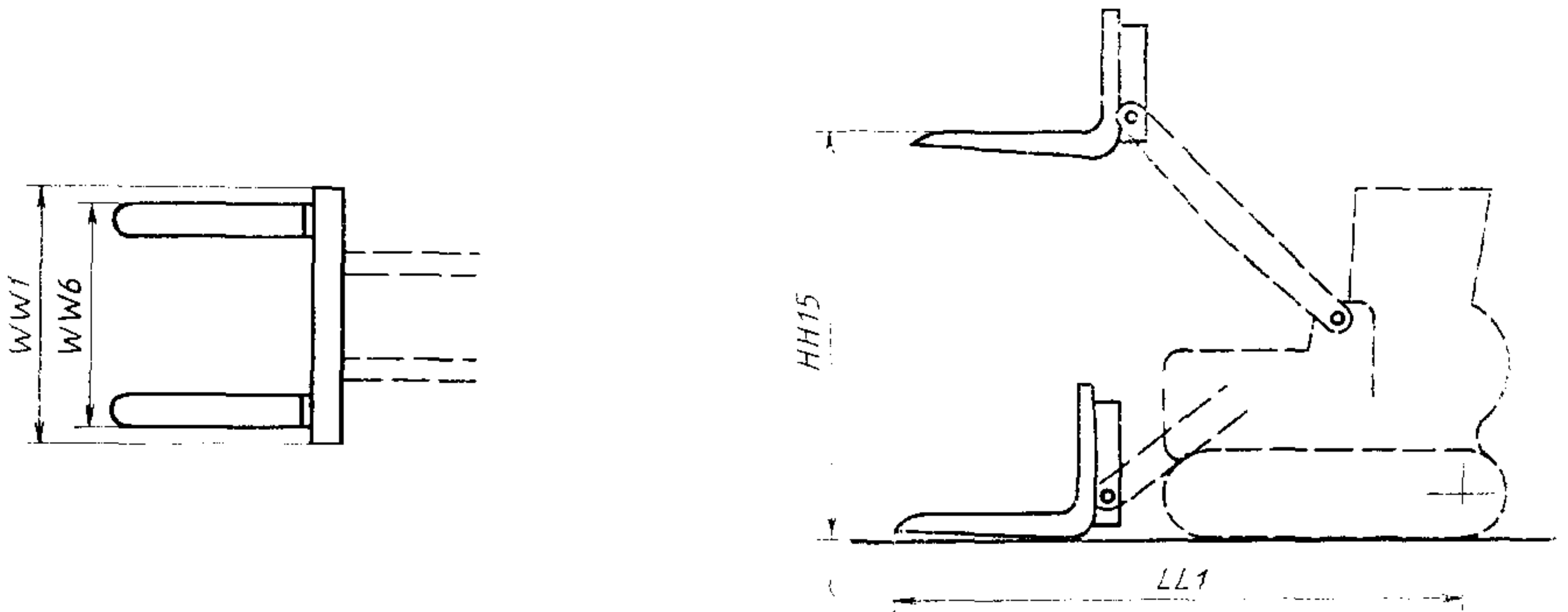
Черт. 21 Размеры грузовых вилок
