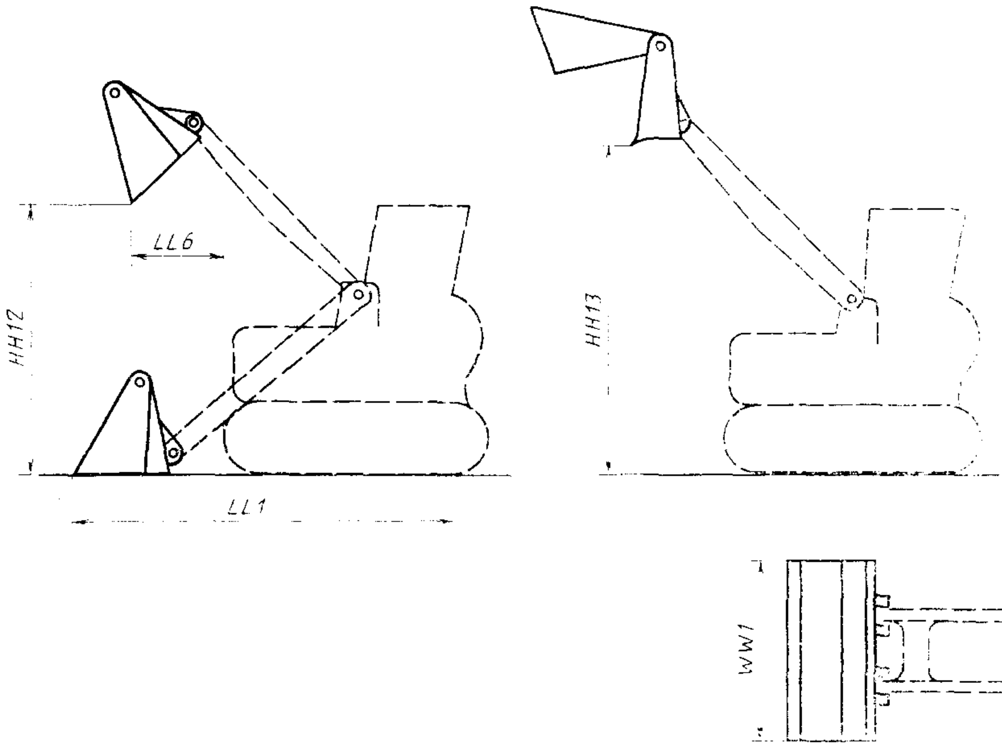
Черт. 20. Размеры двухчелюстного ковша
