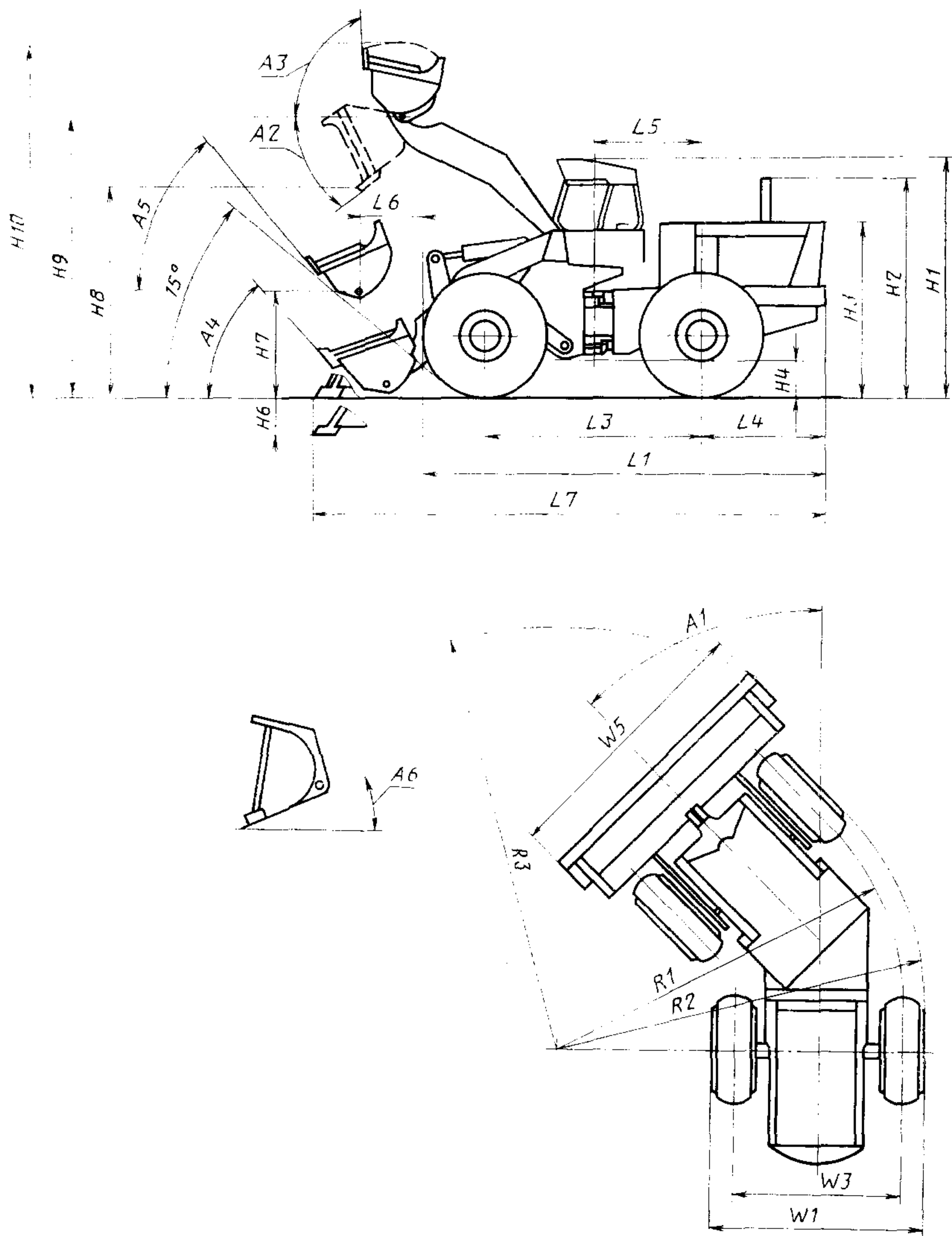
Черт. 16. Размеры базовой машины (колесного погрузчика)
