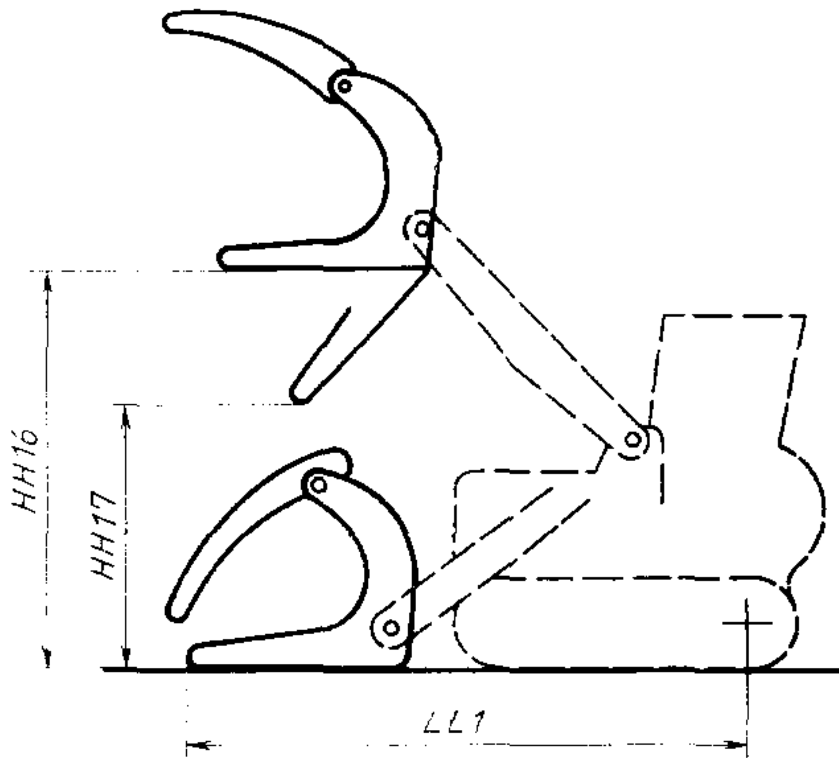
Черт. 22. Размеры челюстного захвата
