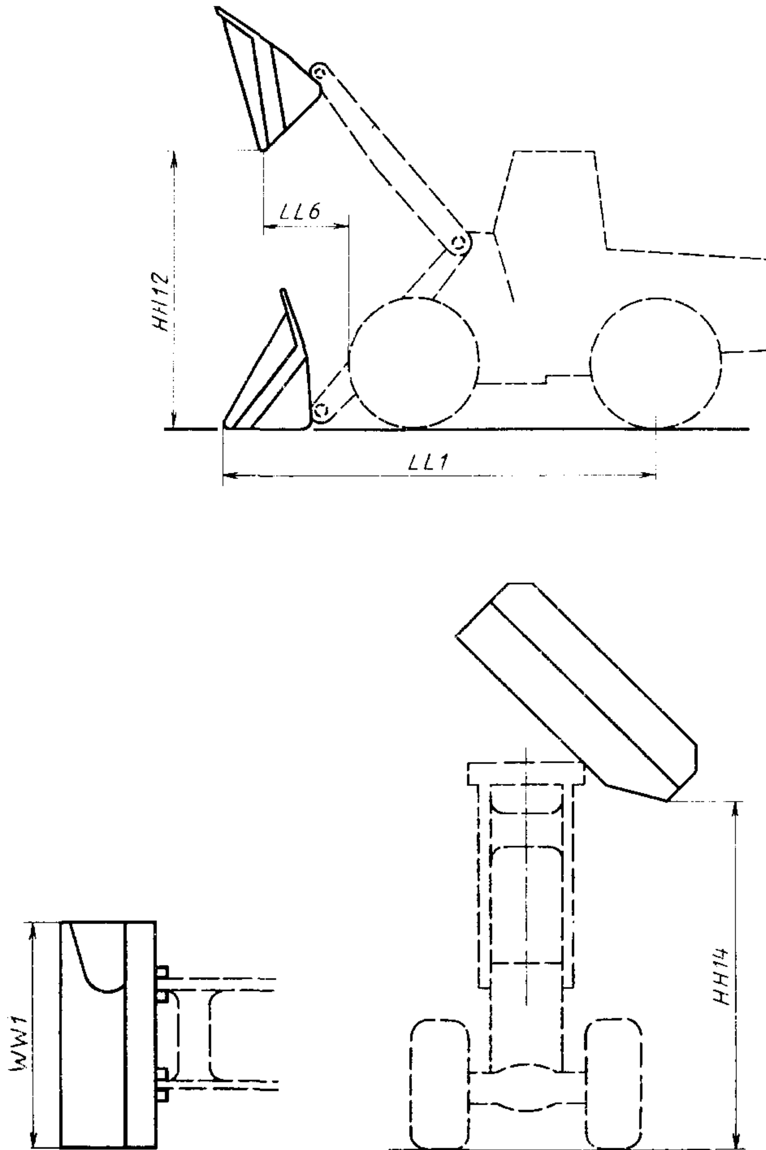
Черт. 19 Размеры ковша с боковой разгрузкой
