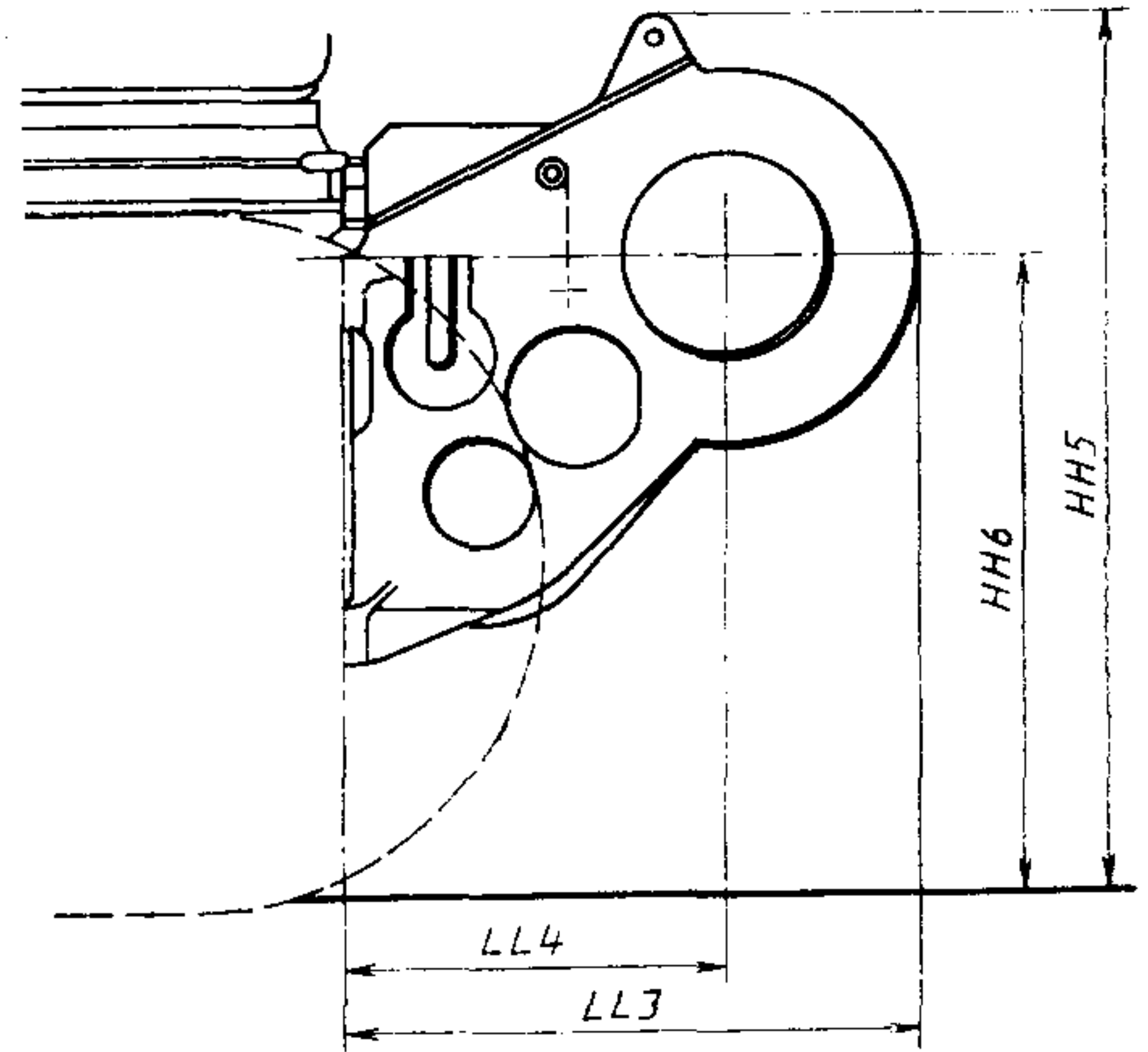
Черт. 23 Размеры лебедки
