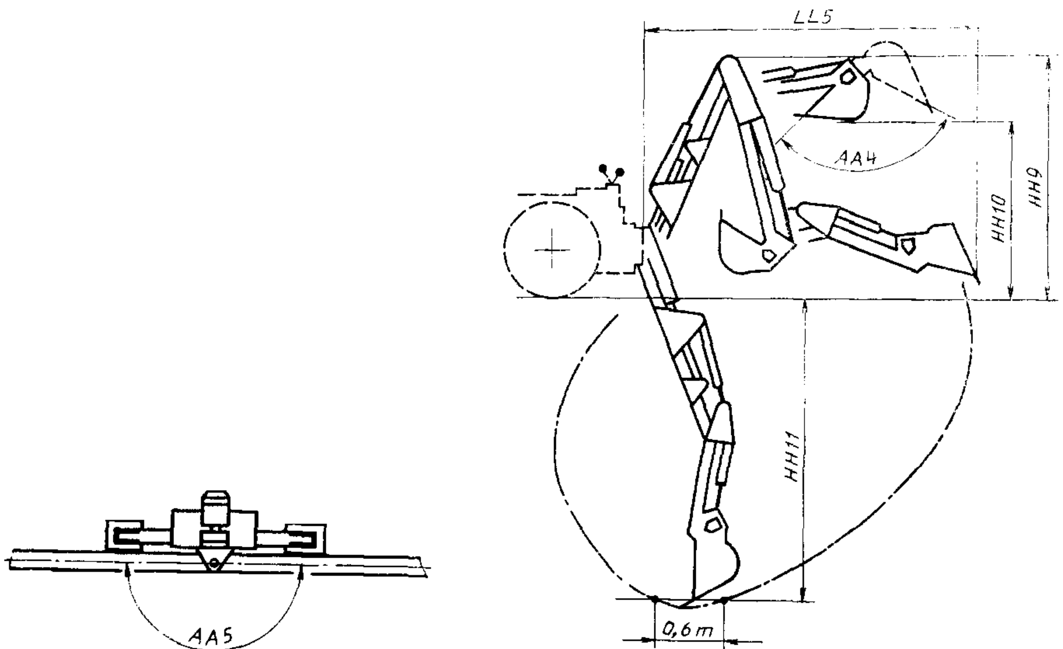
Черт. 17. Размеры обратной лопаты
