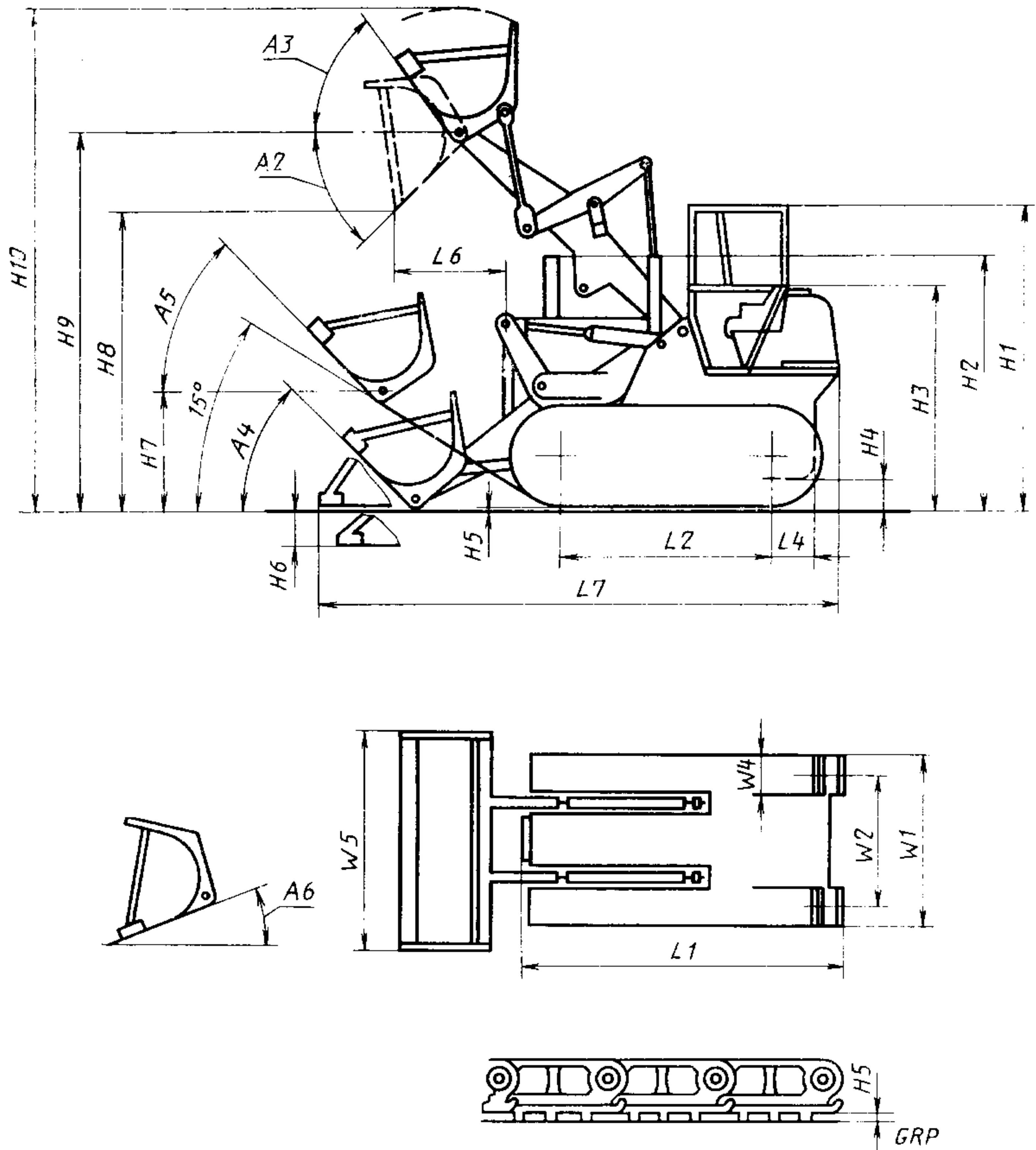
Черт. 15. Размеры базовой машины (гусеничный погрузчик)
