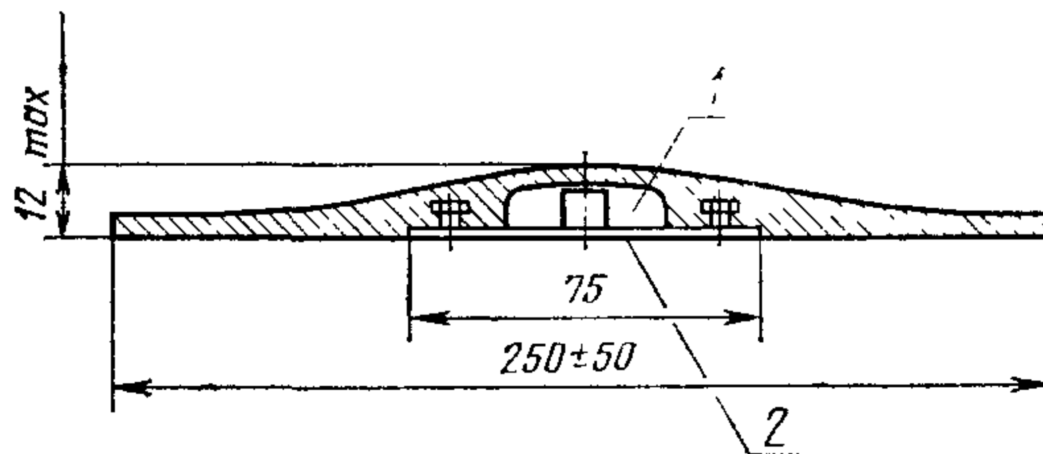
1 — углубление для акселерометра; 2 — тонкий металлический диск для установки акселерометра и увеличения жесткости средней части
