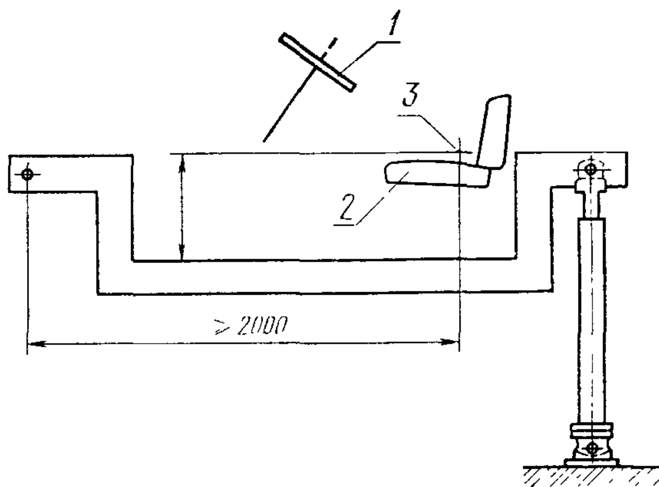
Схема вибростенда для испытаний сиденья оператора
