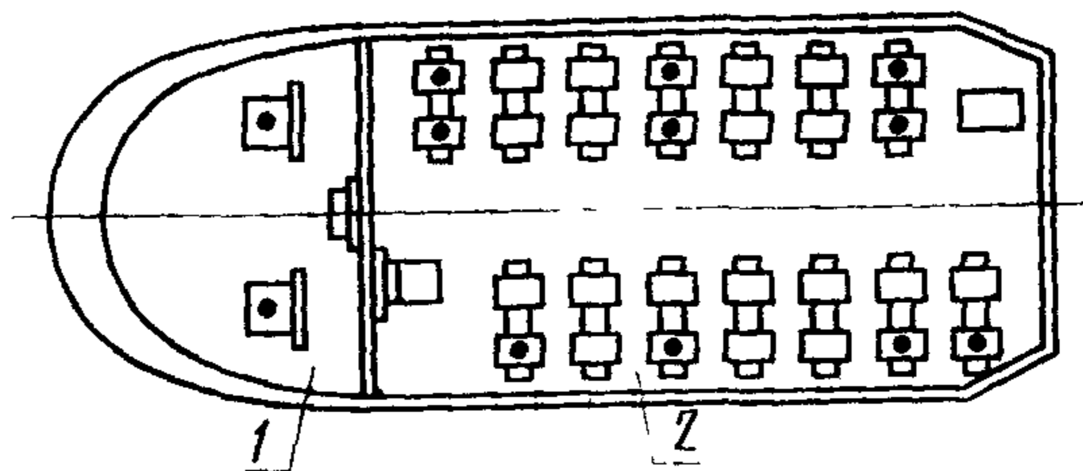
1—кабина экипажа; 2—салон Черт. 5
