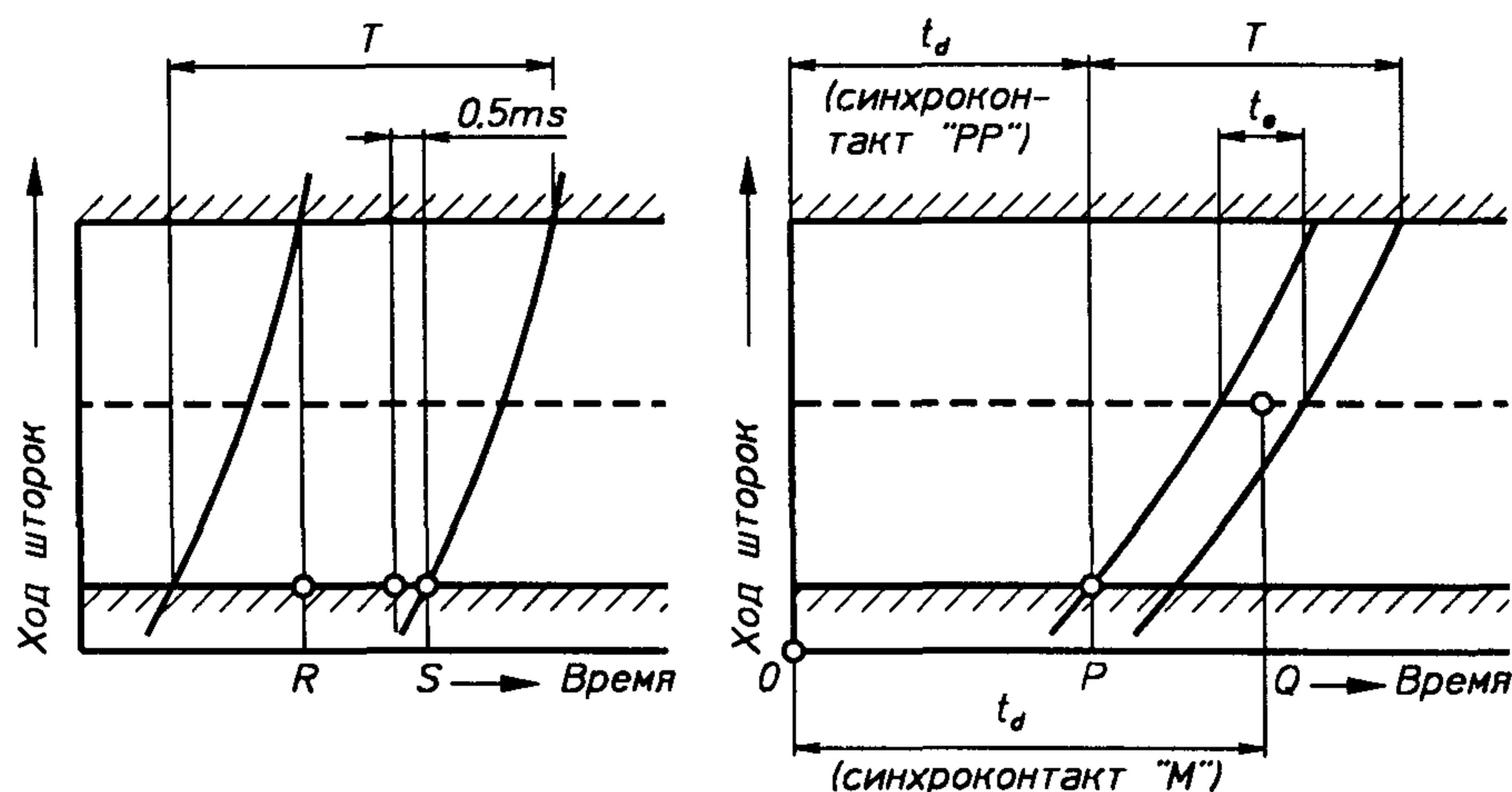
а) Для синхроконтакта типа X
