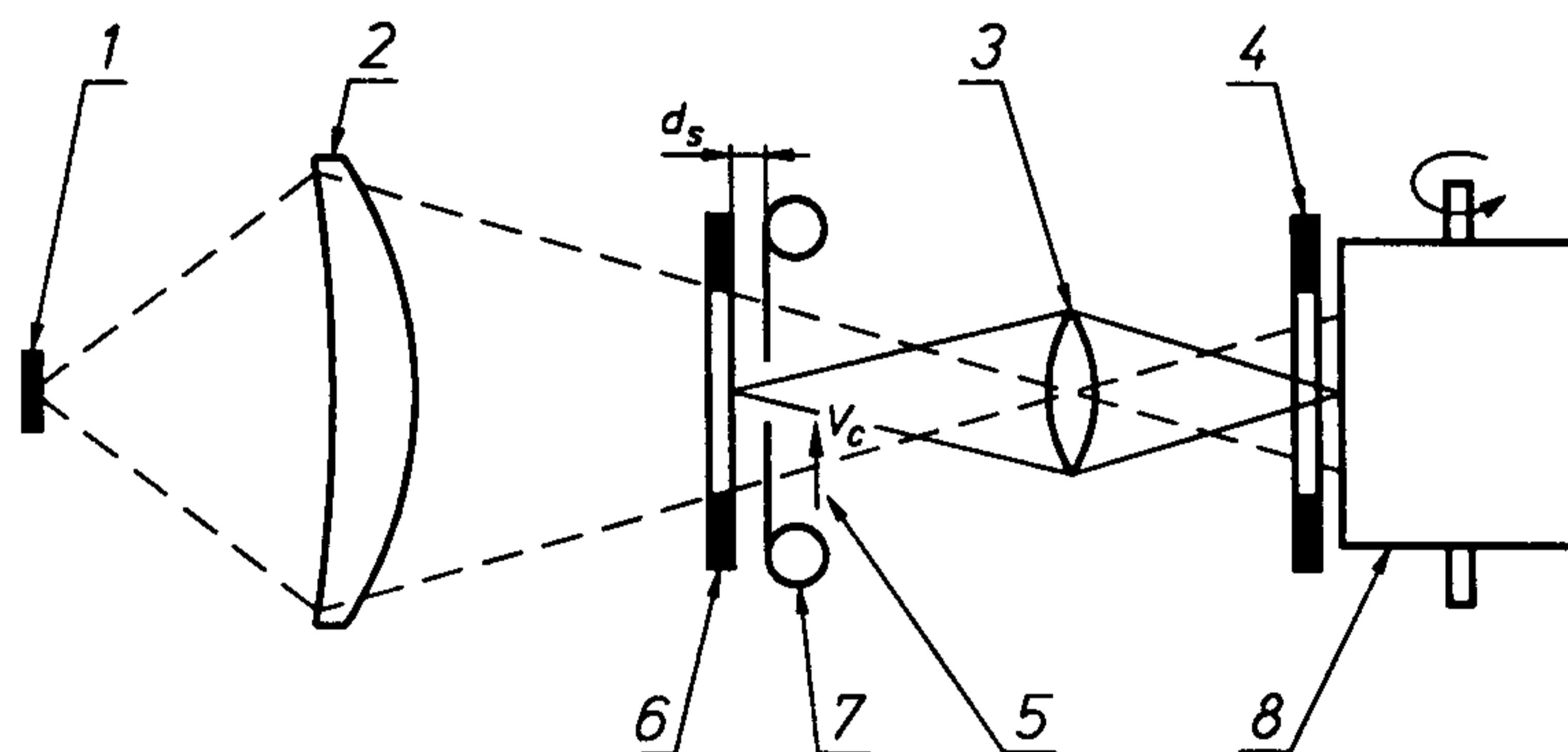
Графический метод для фокальных затворов
