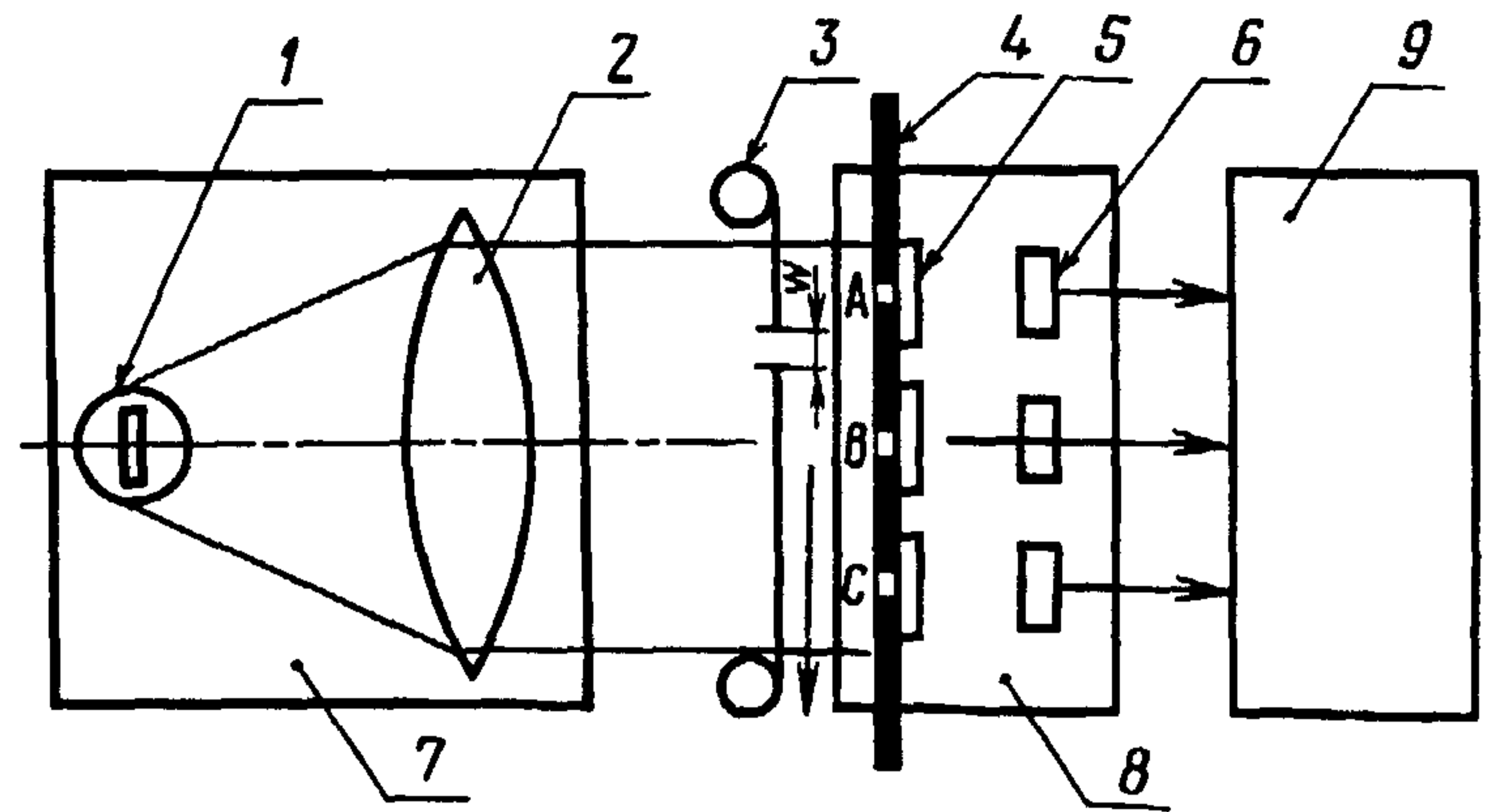
1 — лампа; 2 — линза; 3 — исполнительный элемент; 4 — маска с входными щелями A, B, C (см. табл. 6); 5 — рассеиватели; 6 — светоприемники; 7 — источник света; 8 — светоприемное устройство; 9 — регистратор временных параметров
