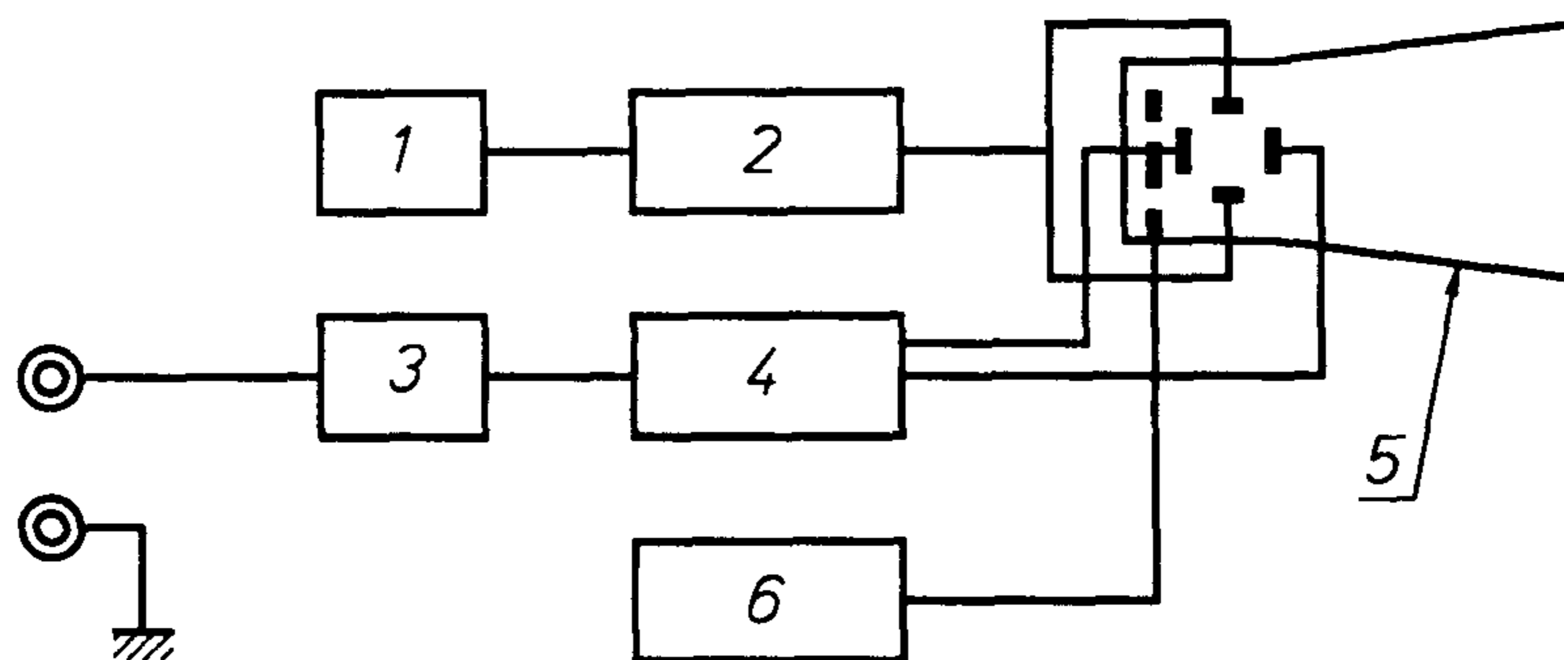
Испытательная схема для апертурных затворов
