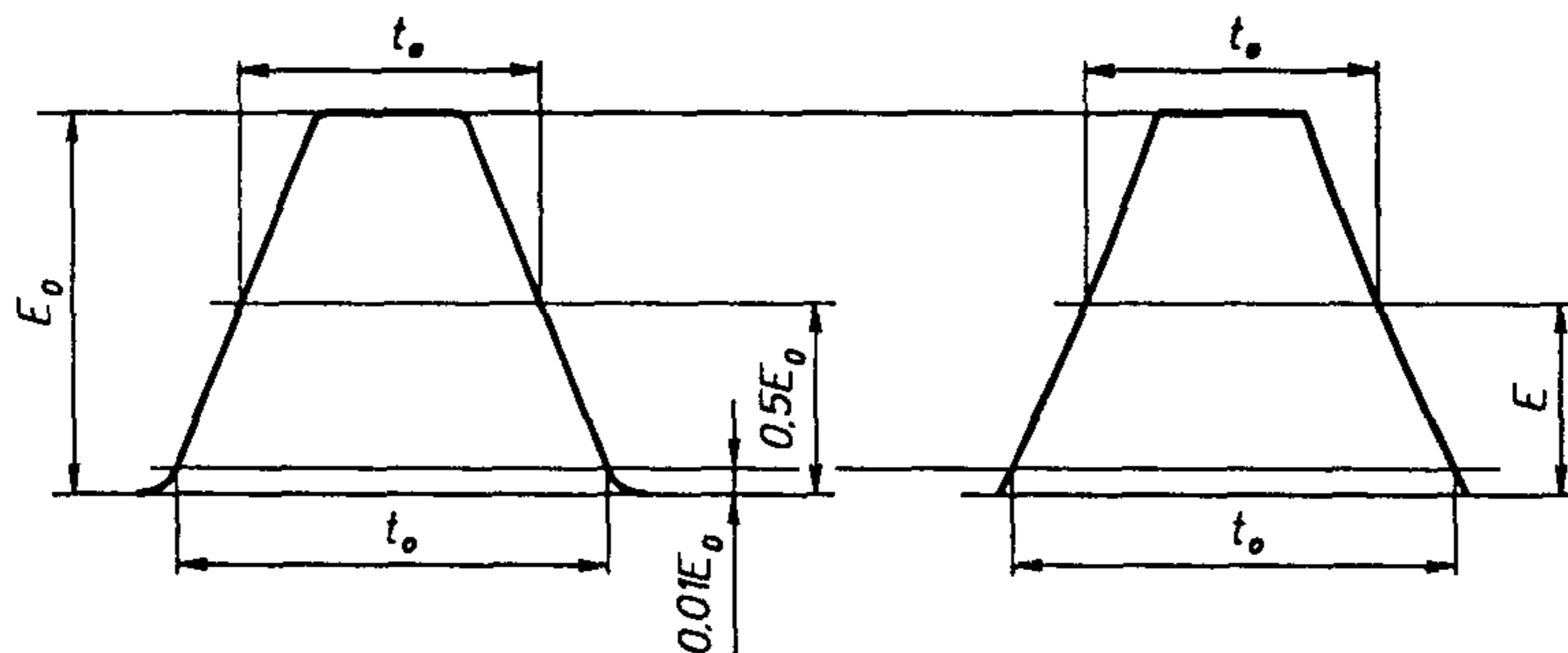
Типичные осциллографические следы
