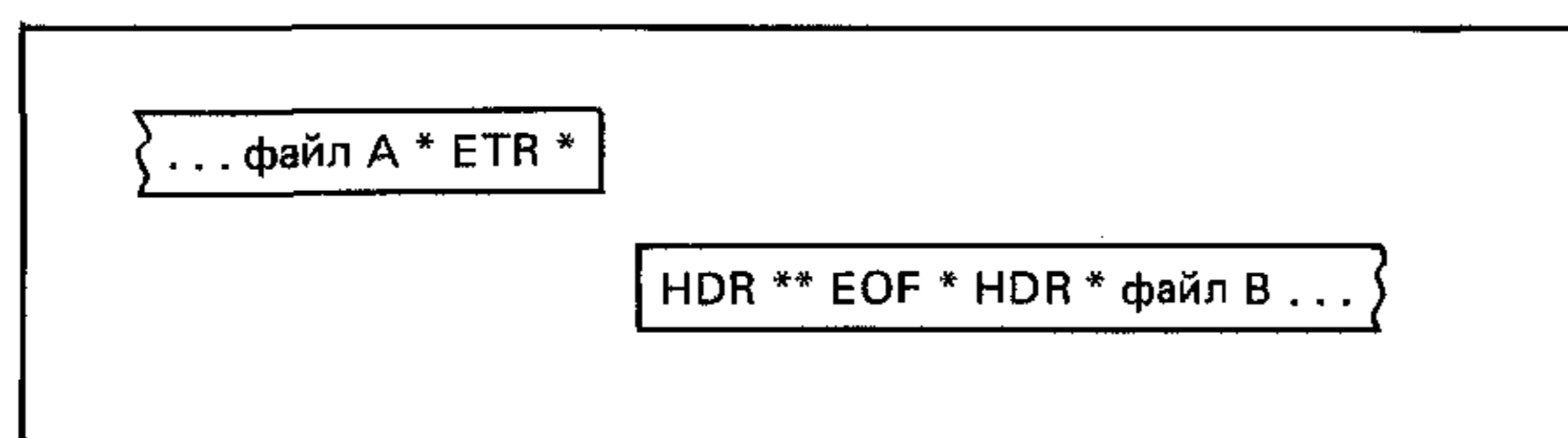
Пустая секция файла в промежуточном начале дорожки
