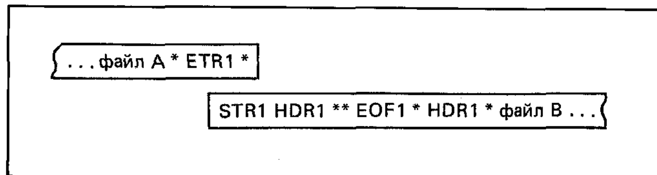
Пустая секция файла в промежуточном начале дорожки
