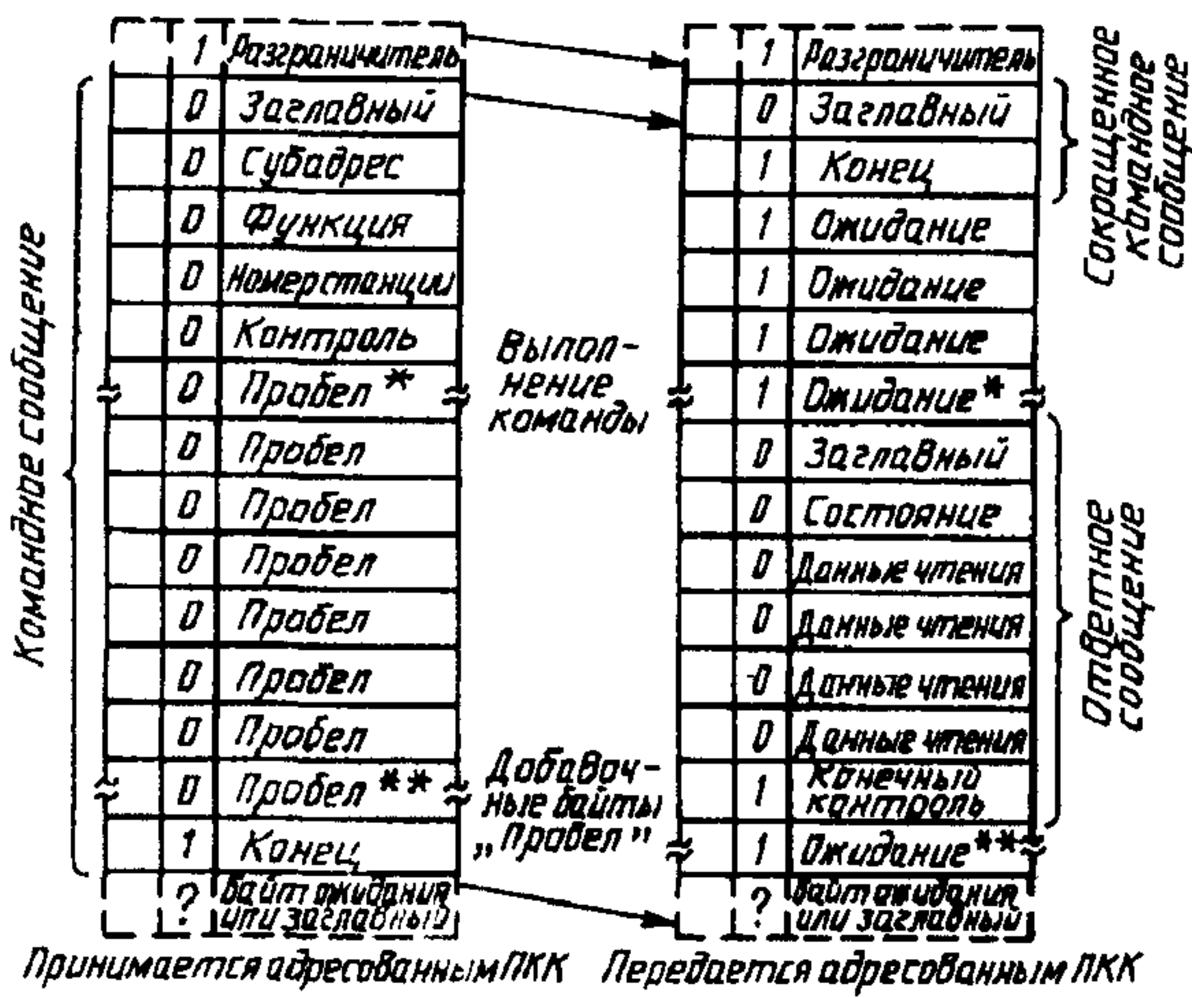
Последовательность обмена команда/ответ: операция чтения, поразрядно-последовательный режим
