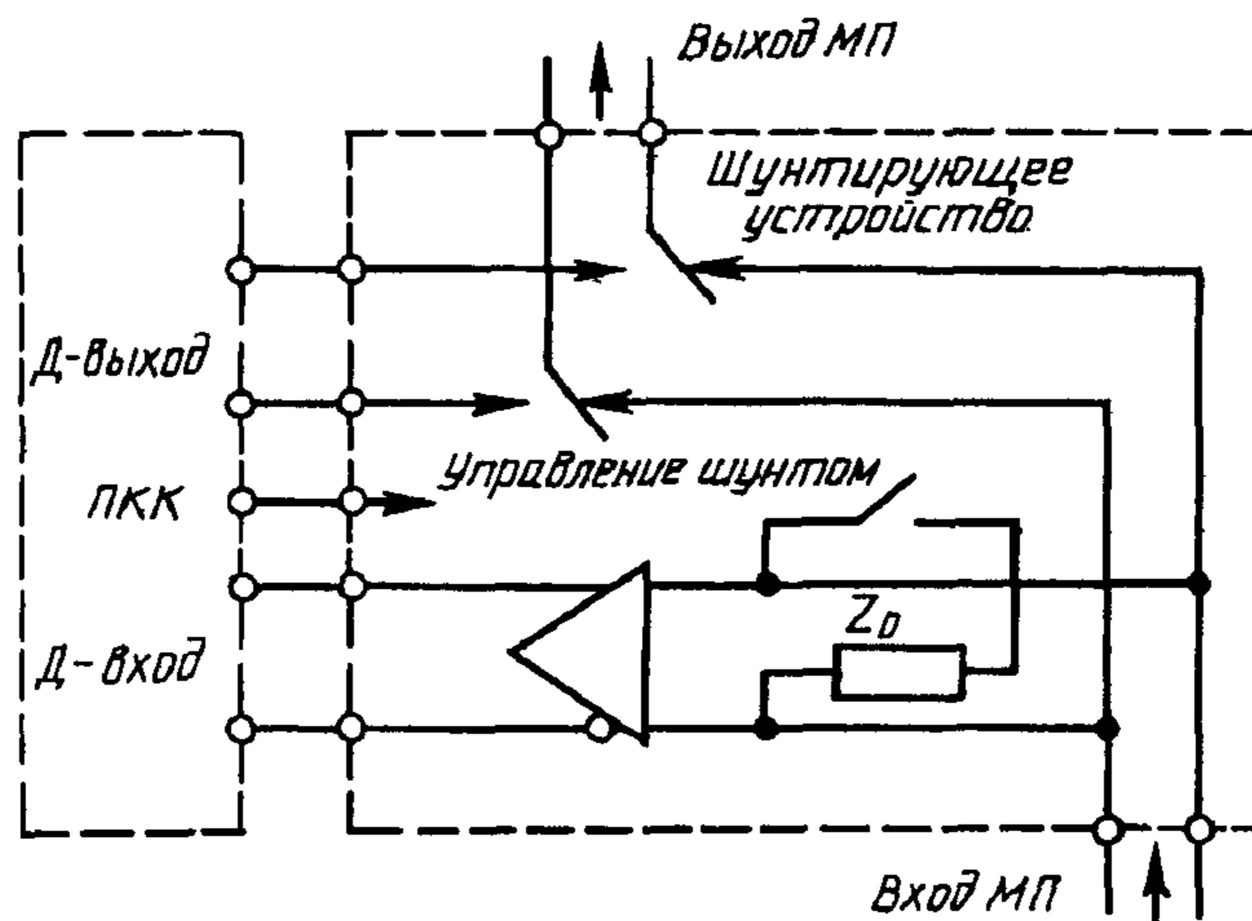
Пример переключения шунта для одного сигнала D-порта
