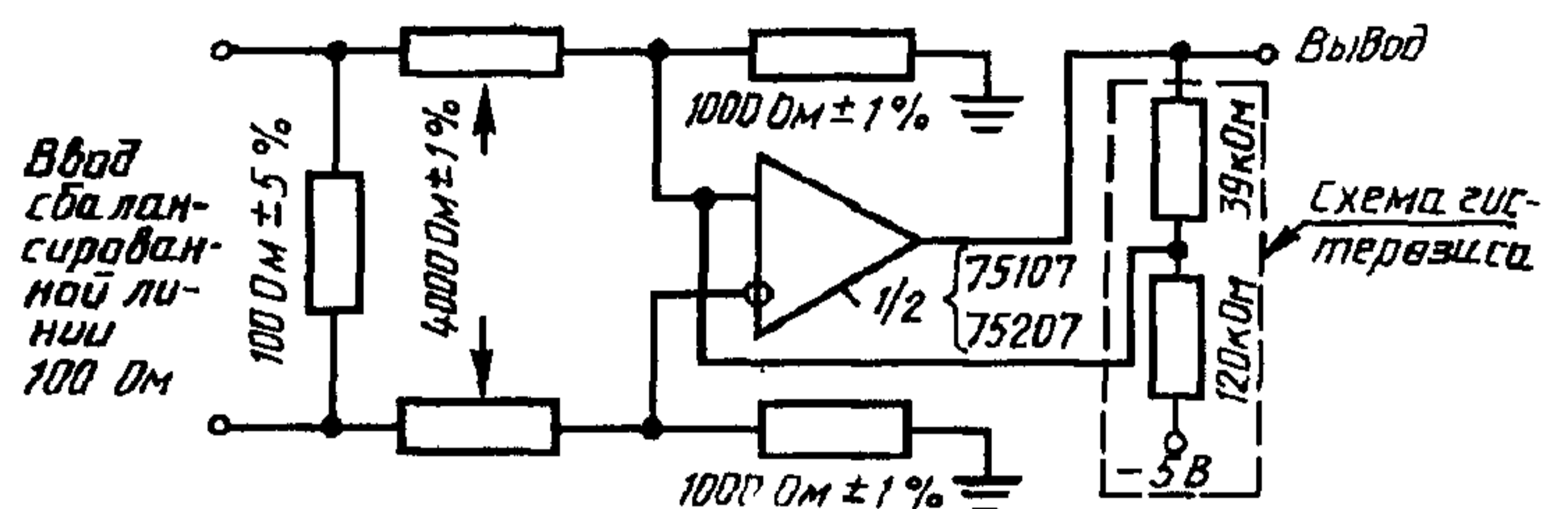
Пример приемника с гистерезисом, дополненным внешними резисторами
