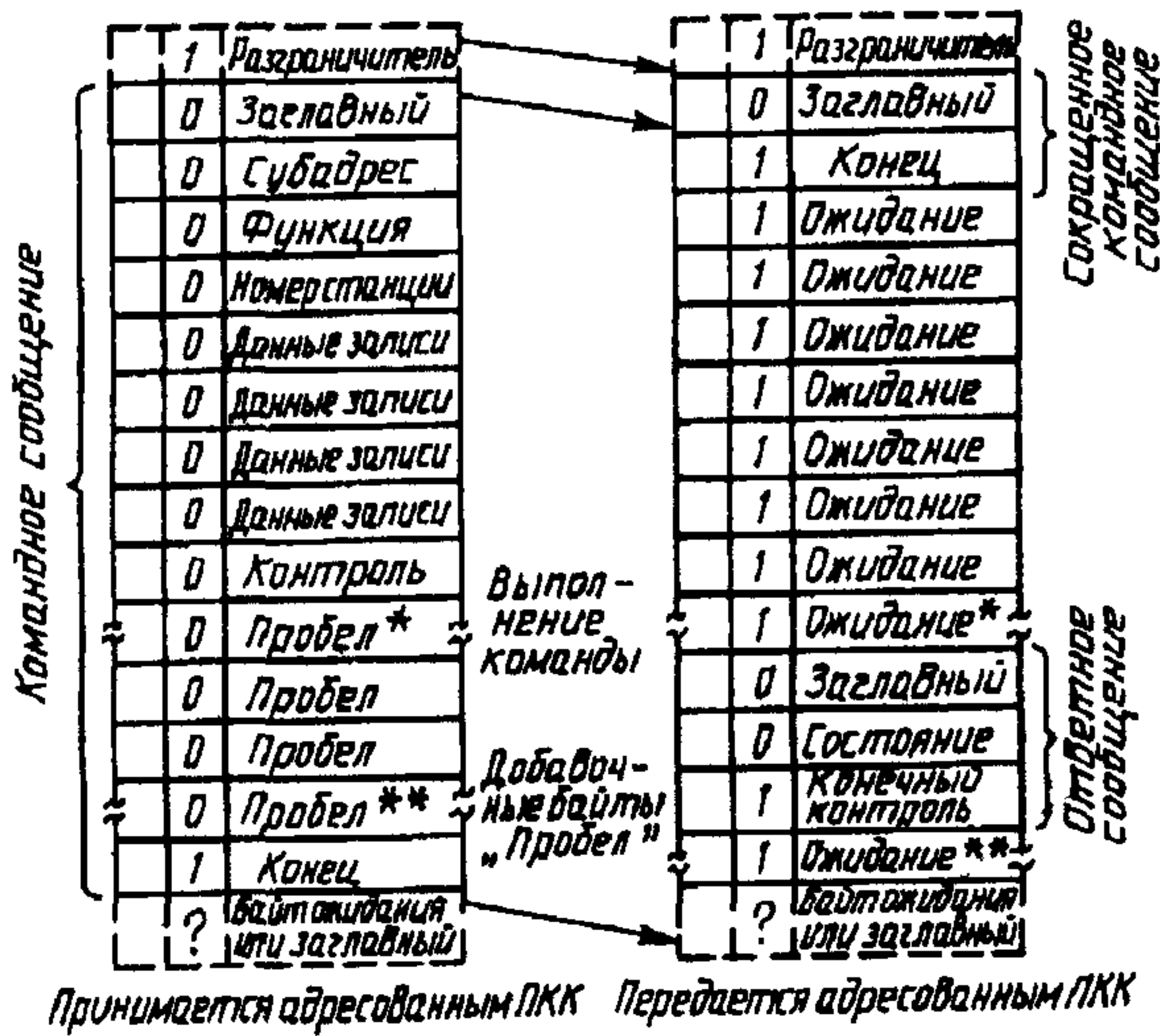
Последовательность обмена команда/ответ: операция записи, поразрядно-последовательный режим
