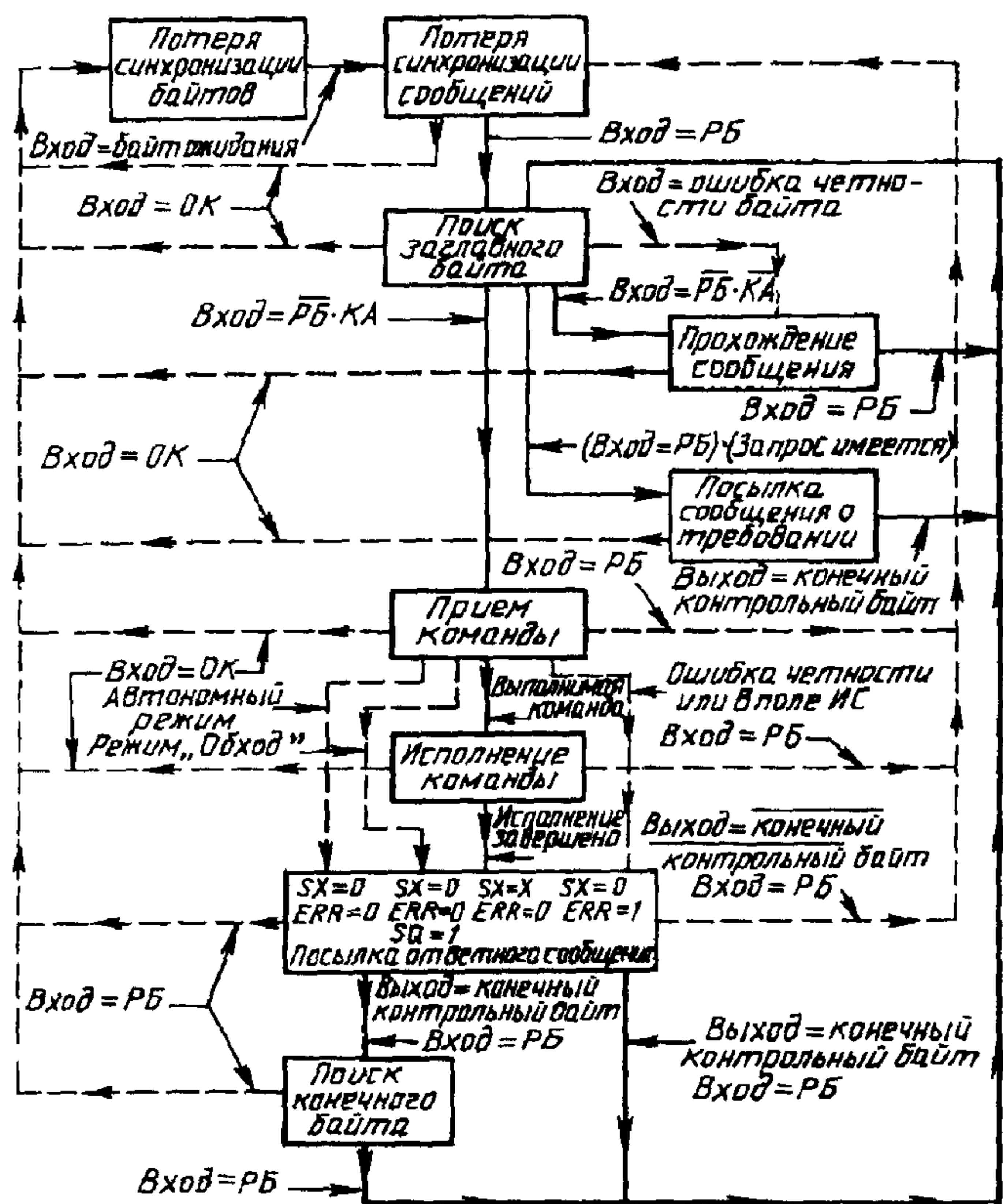
Последовательность основных состояний ПКК
