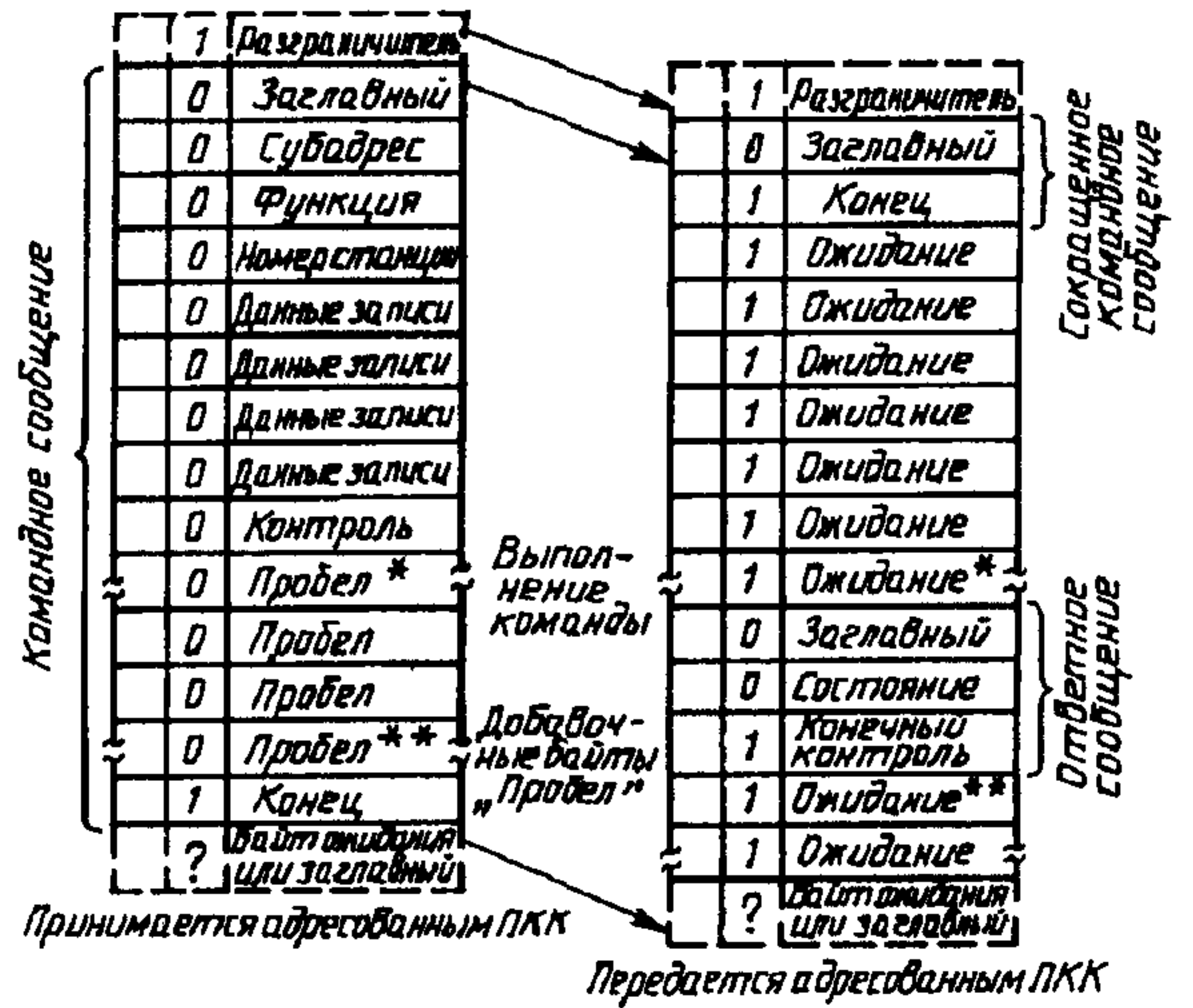
Последовательность обмена команда/ответ: операция записи, побайтно-последовательный режим
