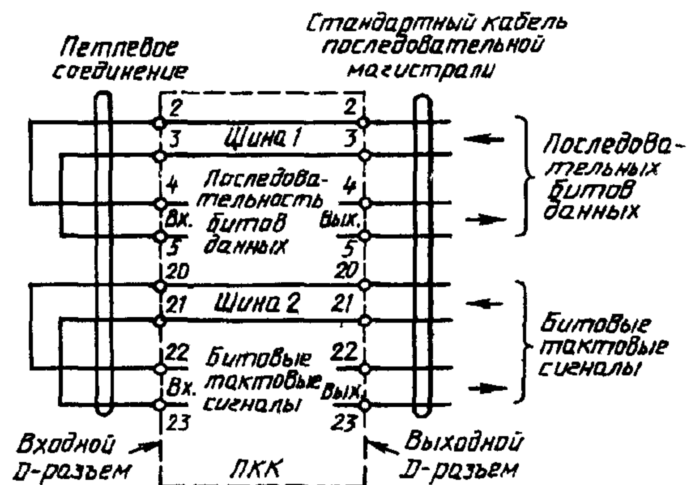
Пример использования контактов шин 1 и 2 D-соединителей
