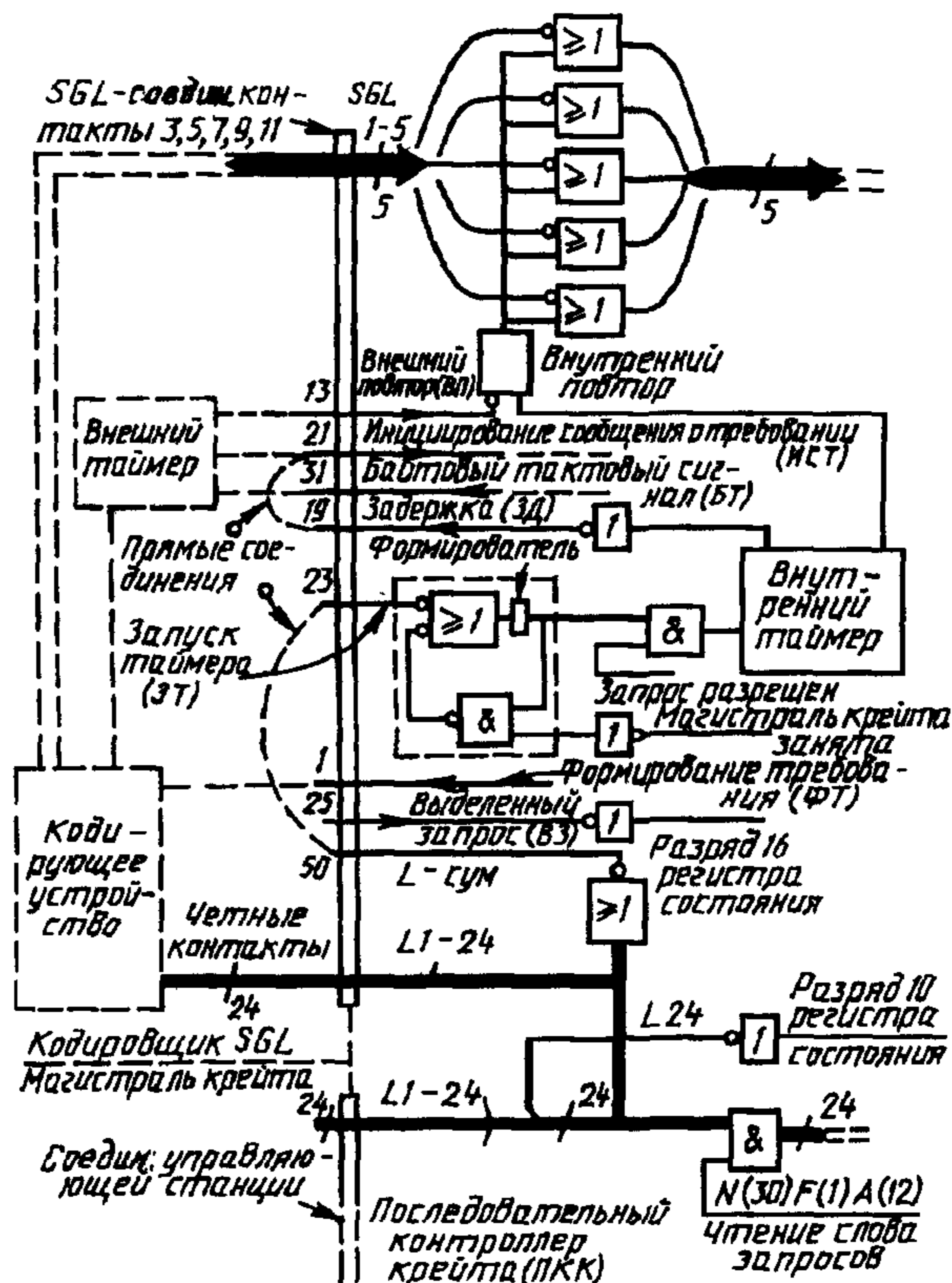
Пример схемы взаимодействия ПКК и кодировщика
