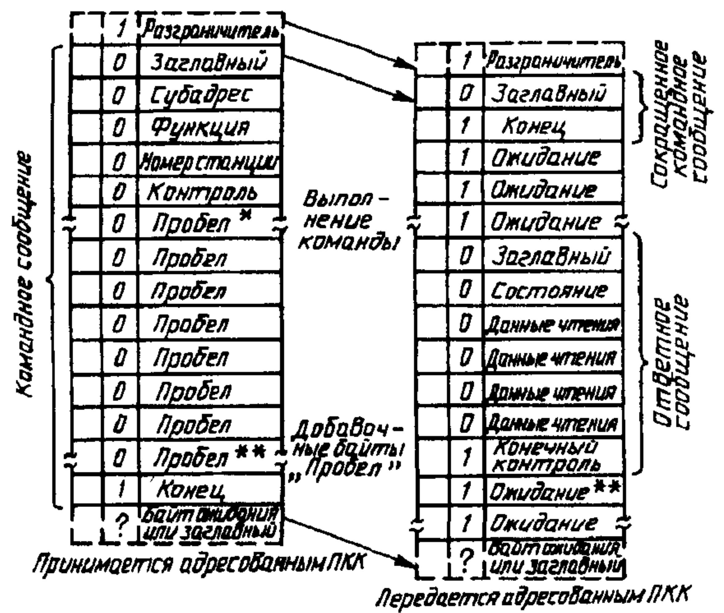
Последовательность обмена команда/ответ: операция чтения, побайтно-последовательный режим
