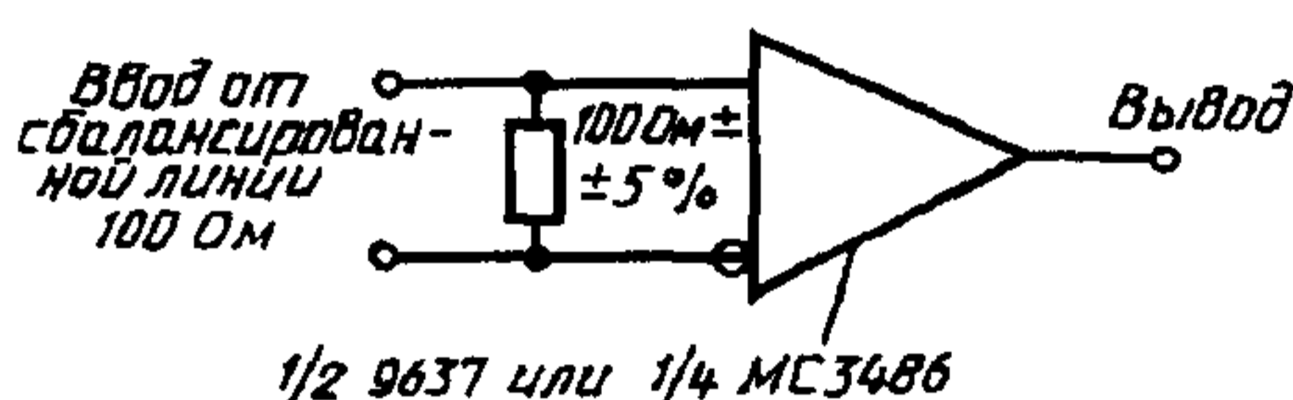
Пример дифференциального приемника
