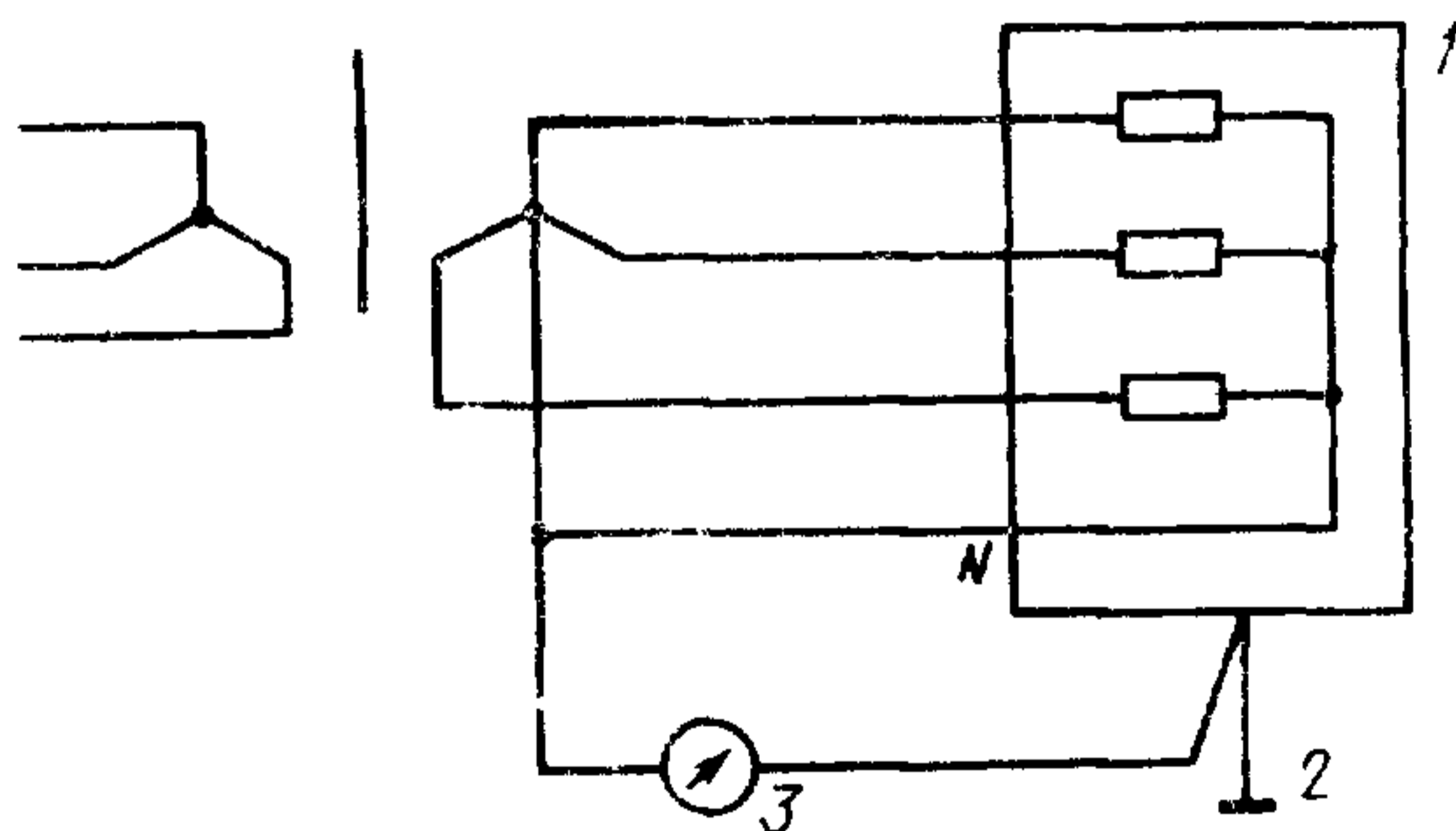
1 — испытуемое устройство, 2 — соединительный зажим заземления; 3 — измерительный прибор
