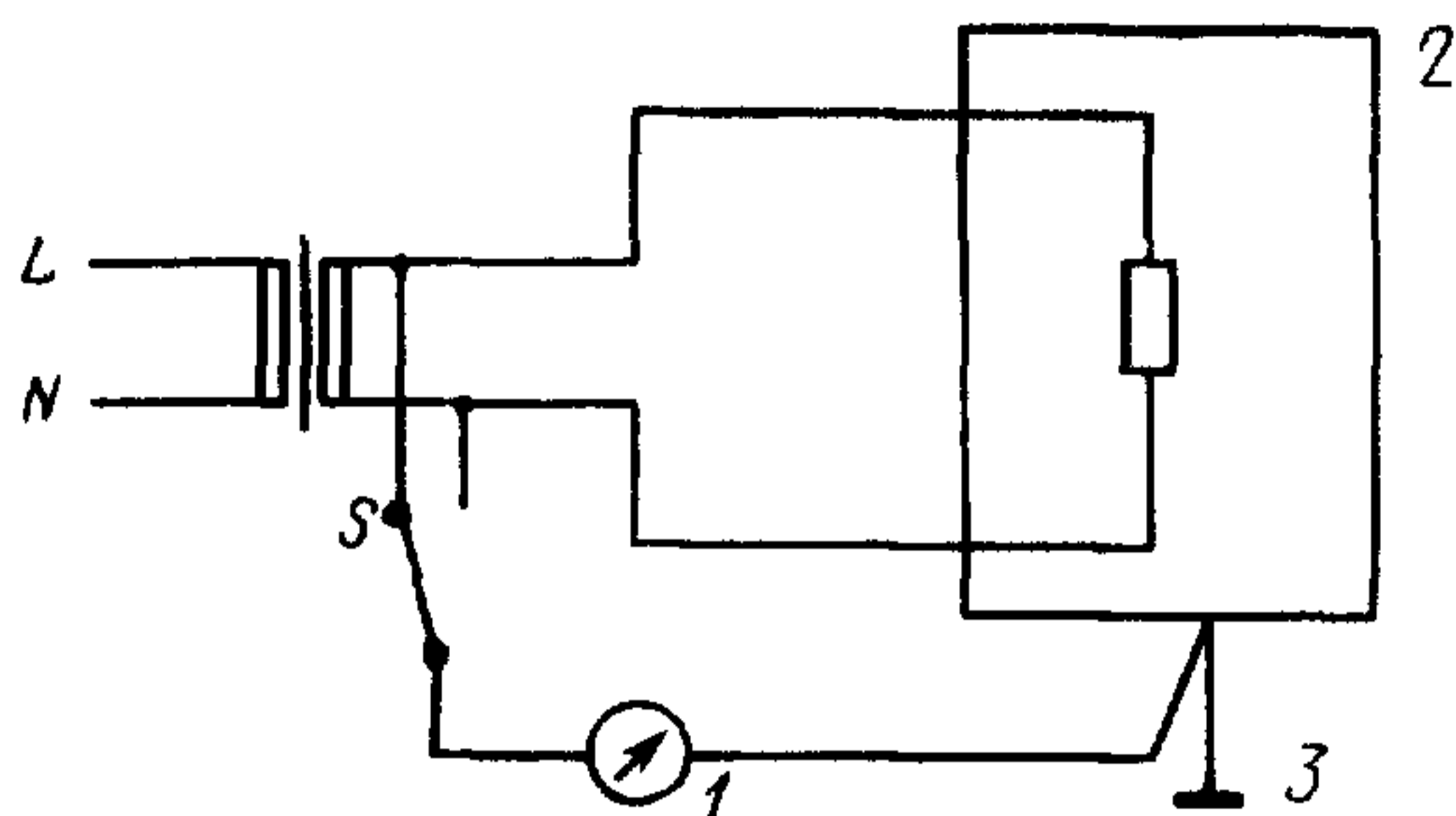
1 — измерительный прибор; 2 — испытуемое устройство; 3 — соединительный зажим заземления
