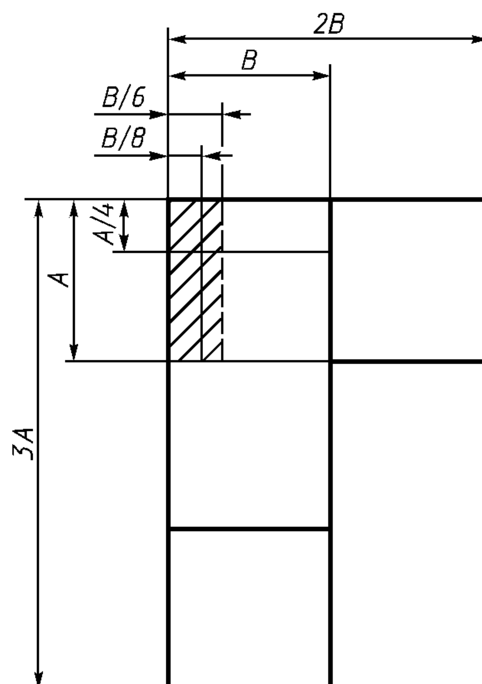
Размеры посадочных окон для панелей, устройств нестоечного типа, блочных каркасов и блоков различного назначения
