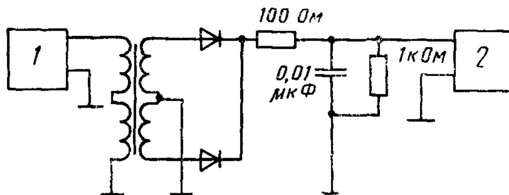
1—испытываемый диктофон; 2—детонометр.
