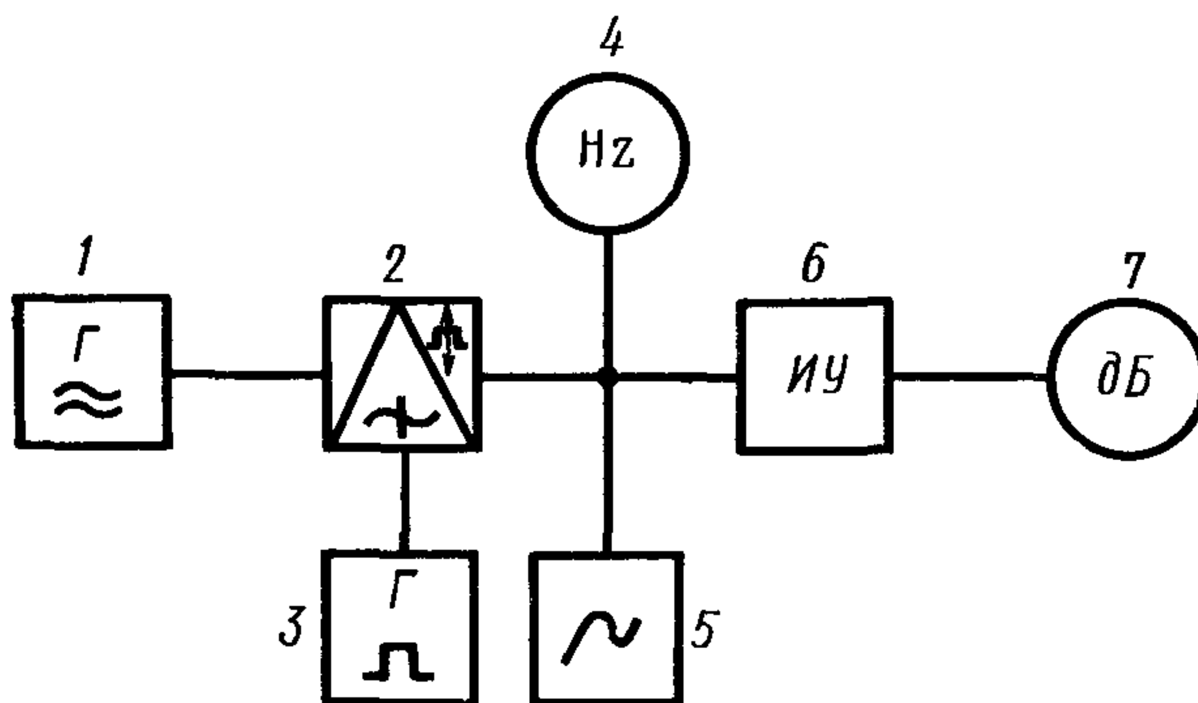
1—звуковой генератор; 2—ключевая схема (импульсный модулятор), 3—генератор прямоугольного напряжения, 4—электро-но-счетный частотомер, 5—осциллограф; 6—электрическая часть испытуемого ИУ, 7—показывающий прибор ИУ.
