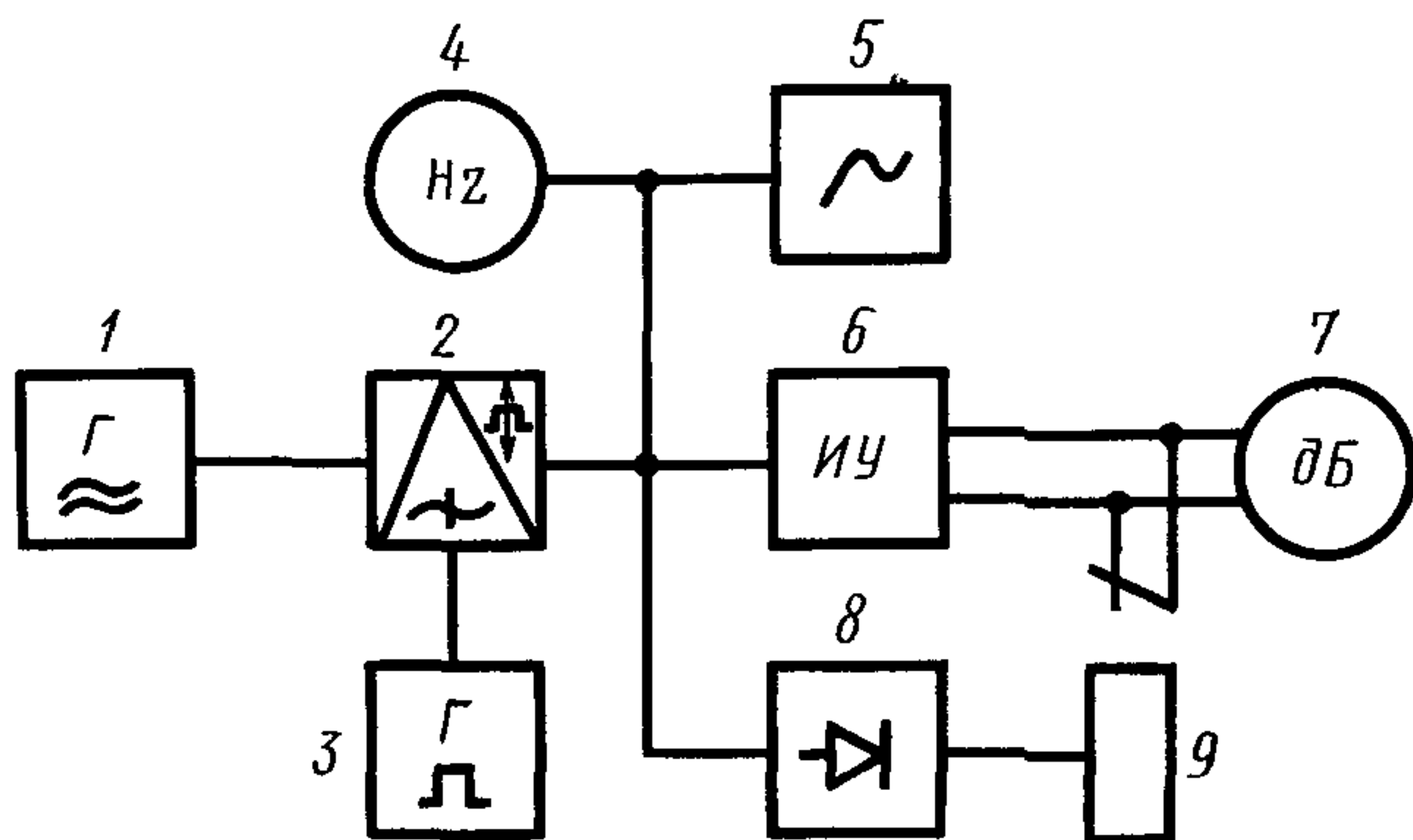
1—звуковой генератор; 2—ключевая схема; 3—генератор прямоугольного напряжения; 4—электронно-счетный частотомер; 5—осциллограф; 6—электрическая часть испытуемого ИУ; 7—показывающий прибор ИУ; 8—мостиковый диодный выпрямитель; 9—реле с временем срабатывания менее 3 мс.
