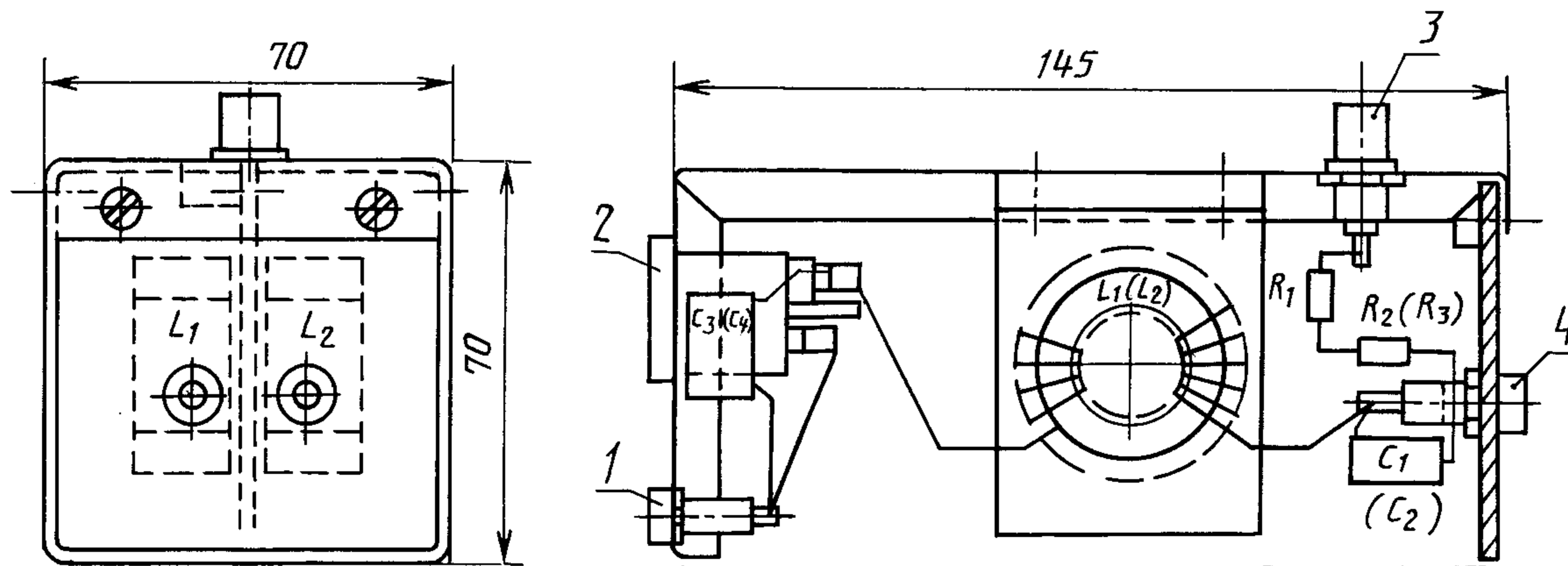
Блок связи типа М. Сборочный чертеж
