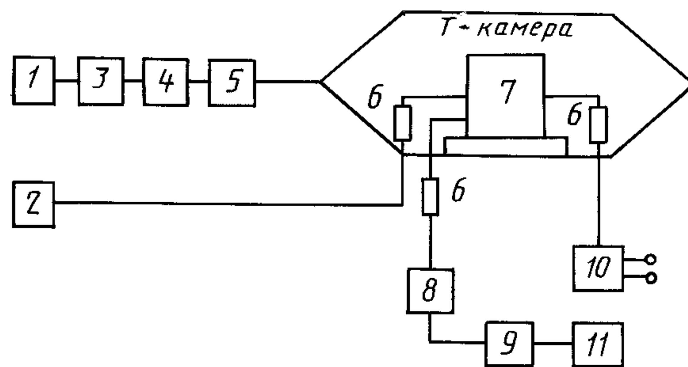
Схема расположения аппаратуры и оборудования при испытаниях на устойчивость к внешним электромагнитным полям в диапазоне частот 0,15—150 МГц
