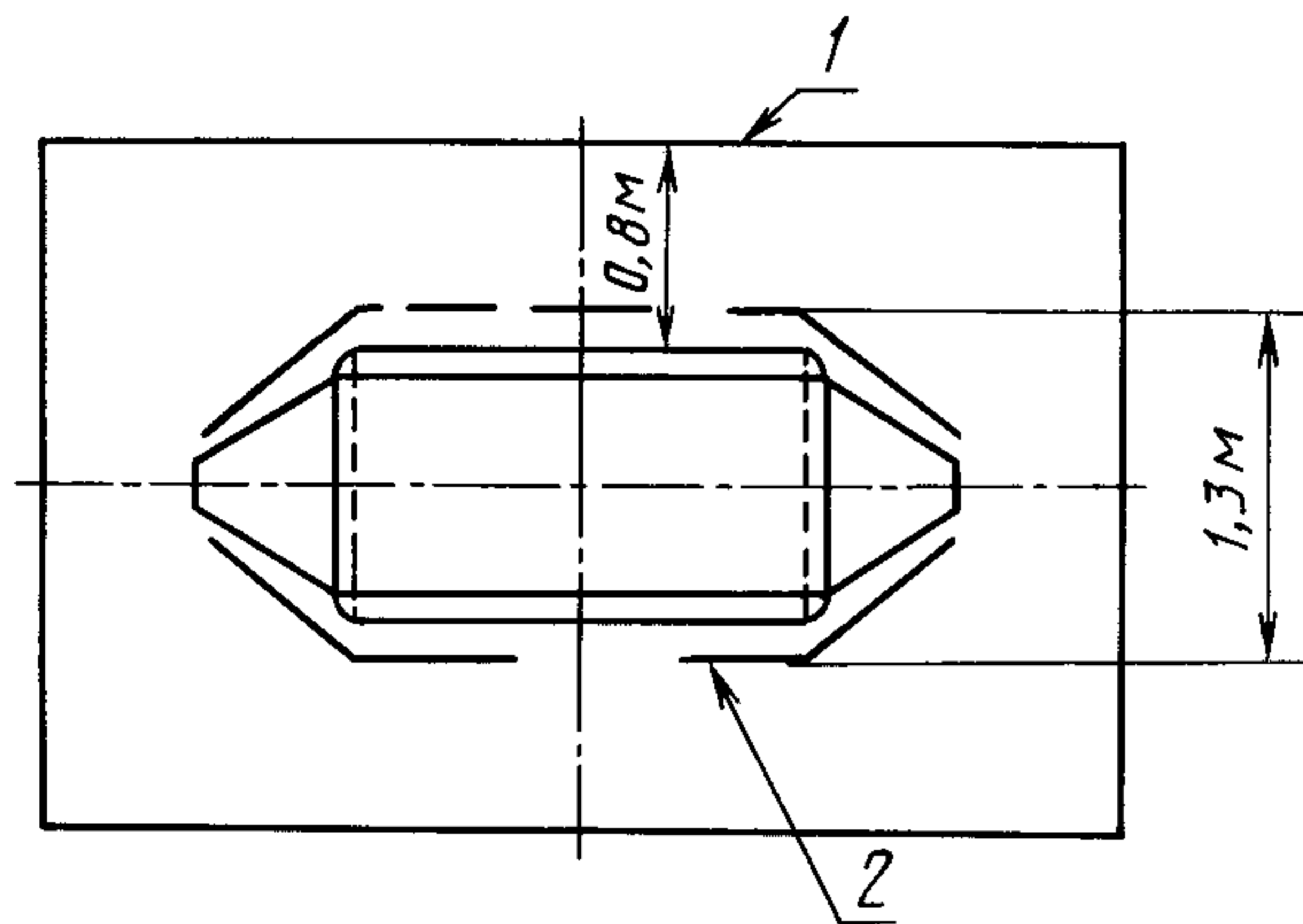
Схема расположения открытой Т-камеры в экранированном помещении
