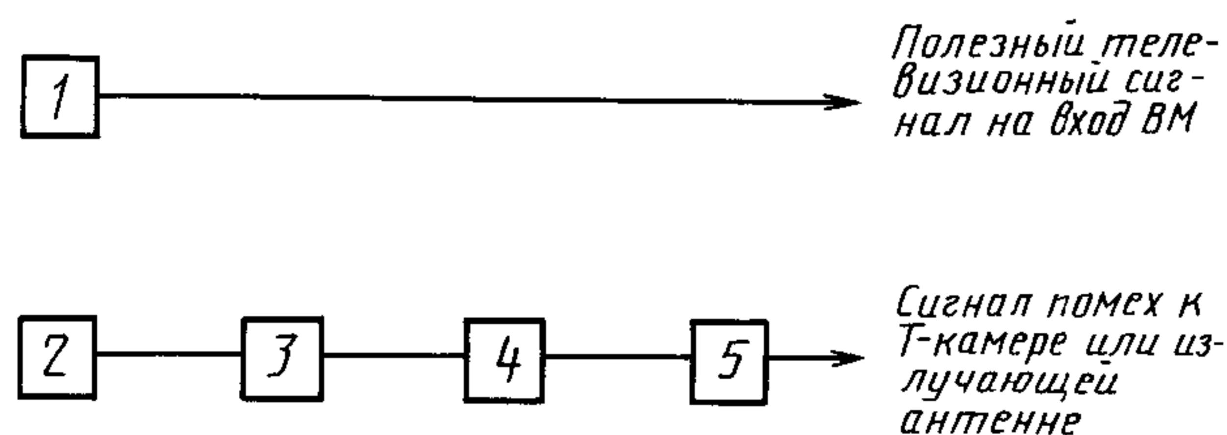
Схема проведения испытаний на устойчивость ВМ к внешним электромагнитным полям
