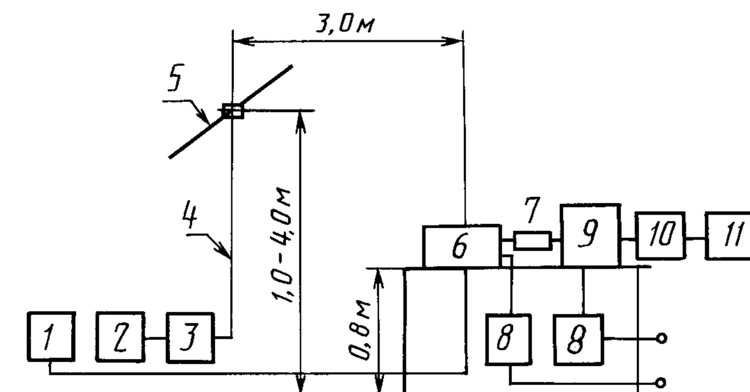
Схема расположения оборудования на измерительной площадке
