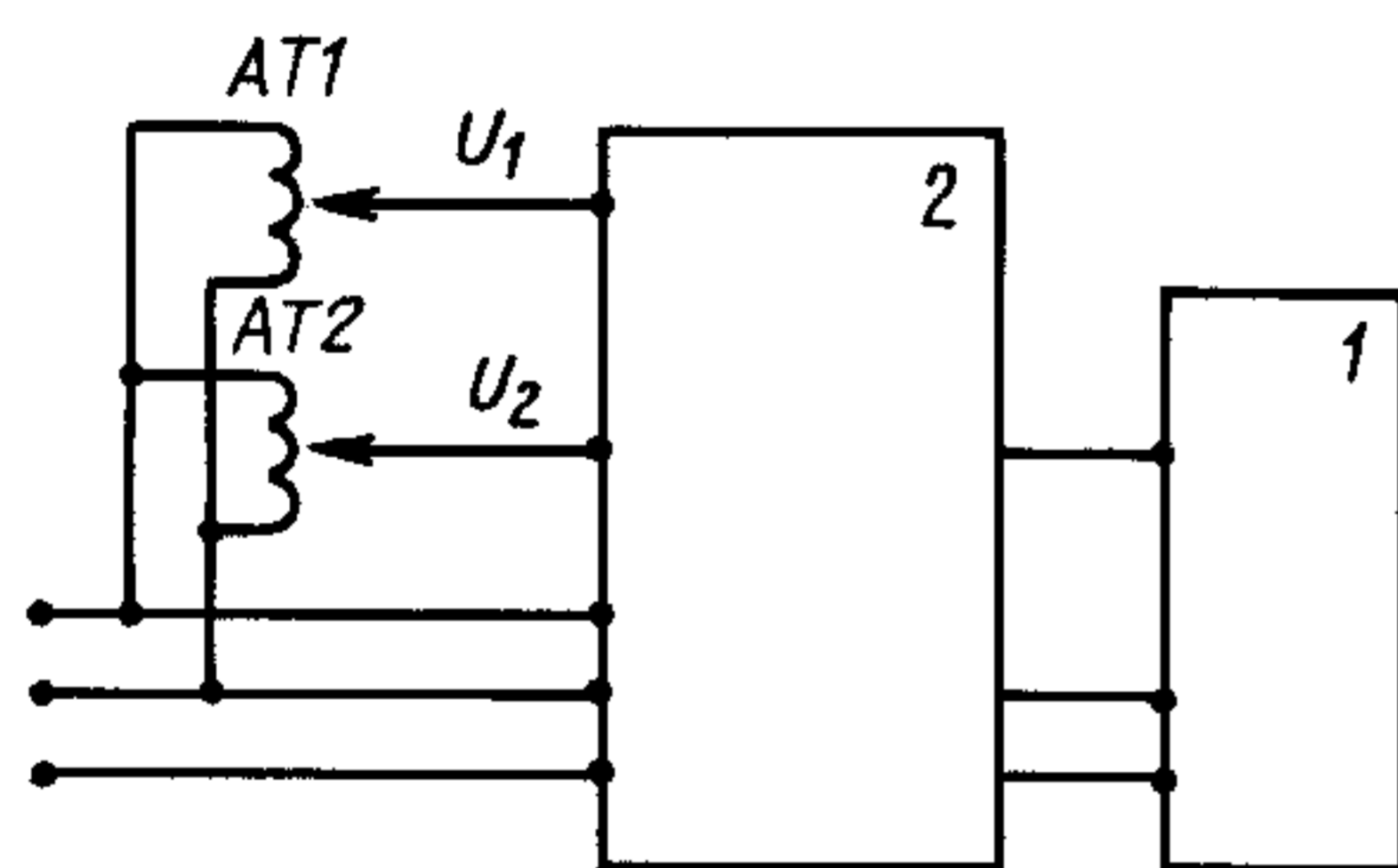
1 — испытуемое изделие; 2 — имитатор помех; AT1, AT2 — автотрансформаторы
