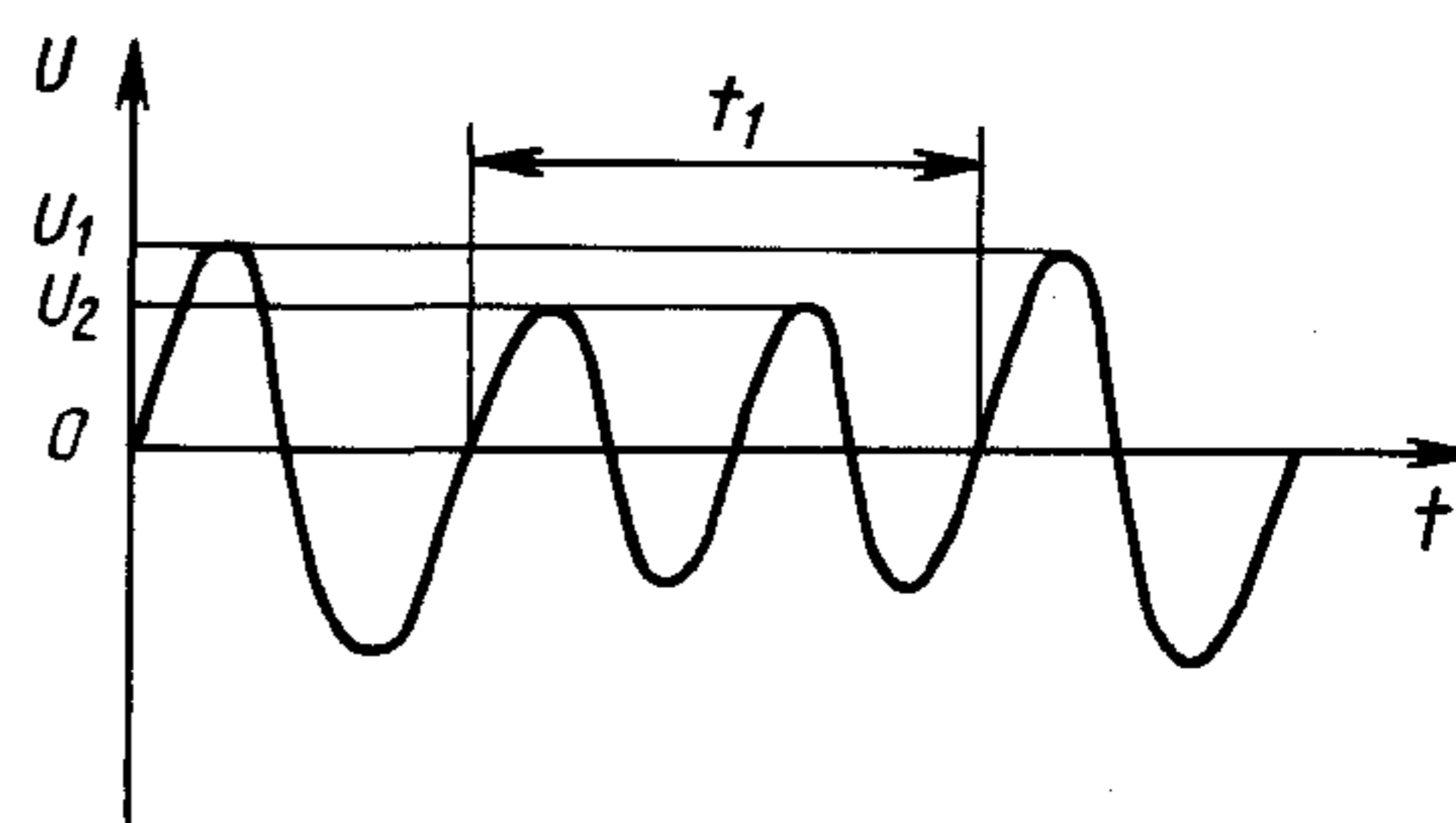
Форма сигнала провала переменного напряжения
