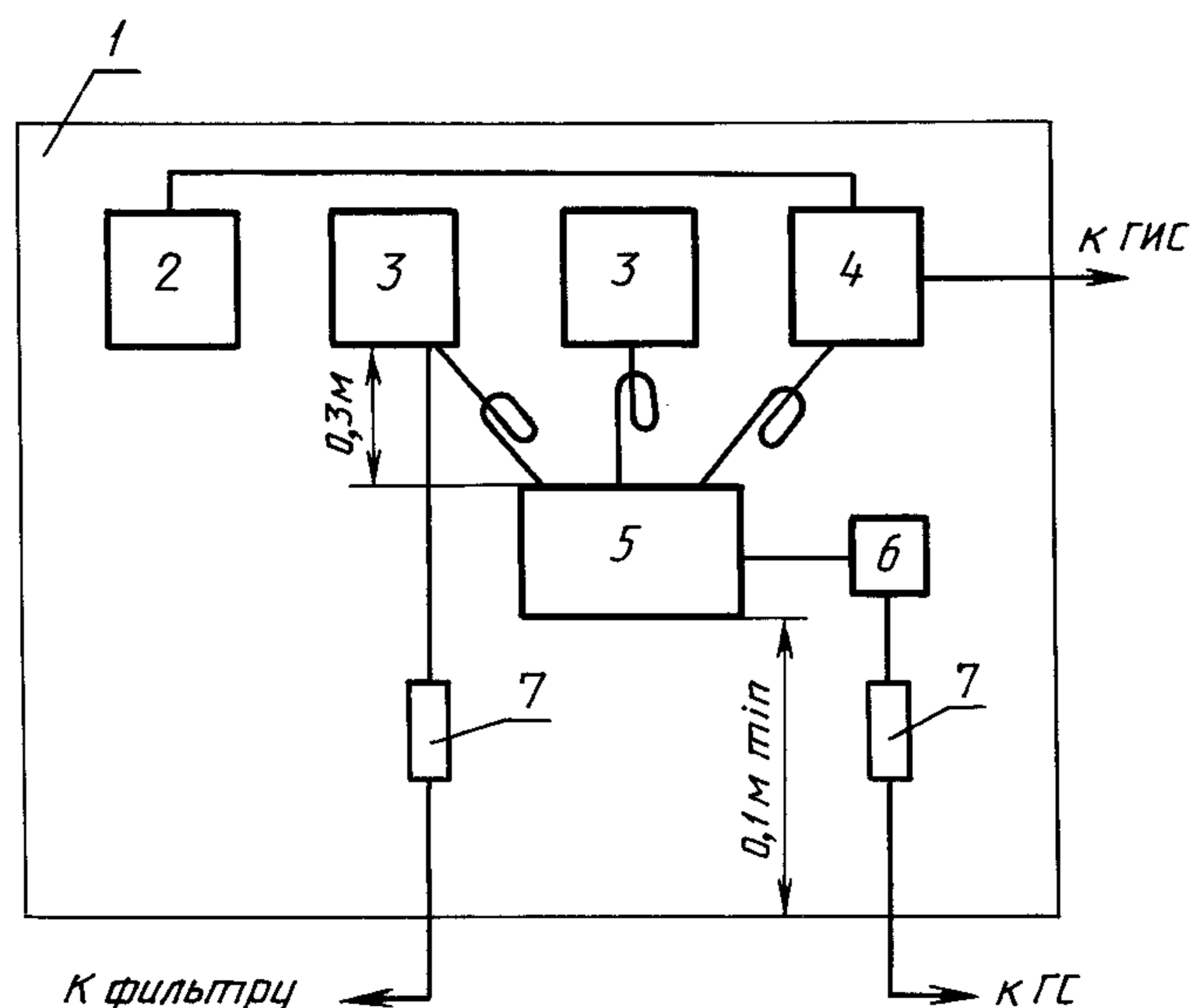
Расположение аппаратуры при измерениях помехозащищенности приемника
