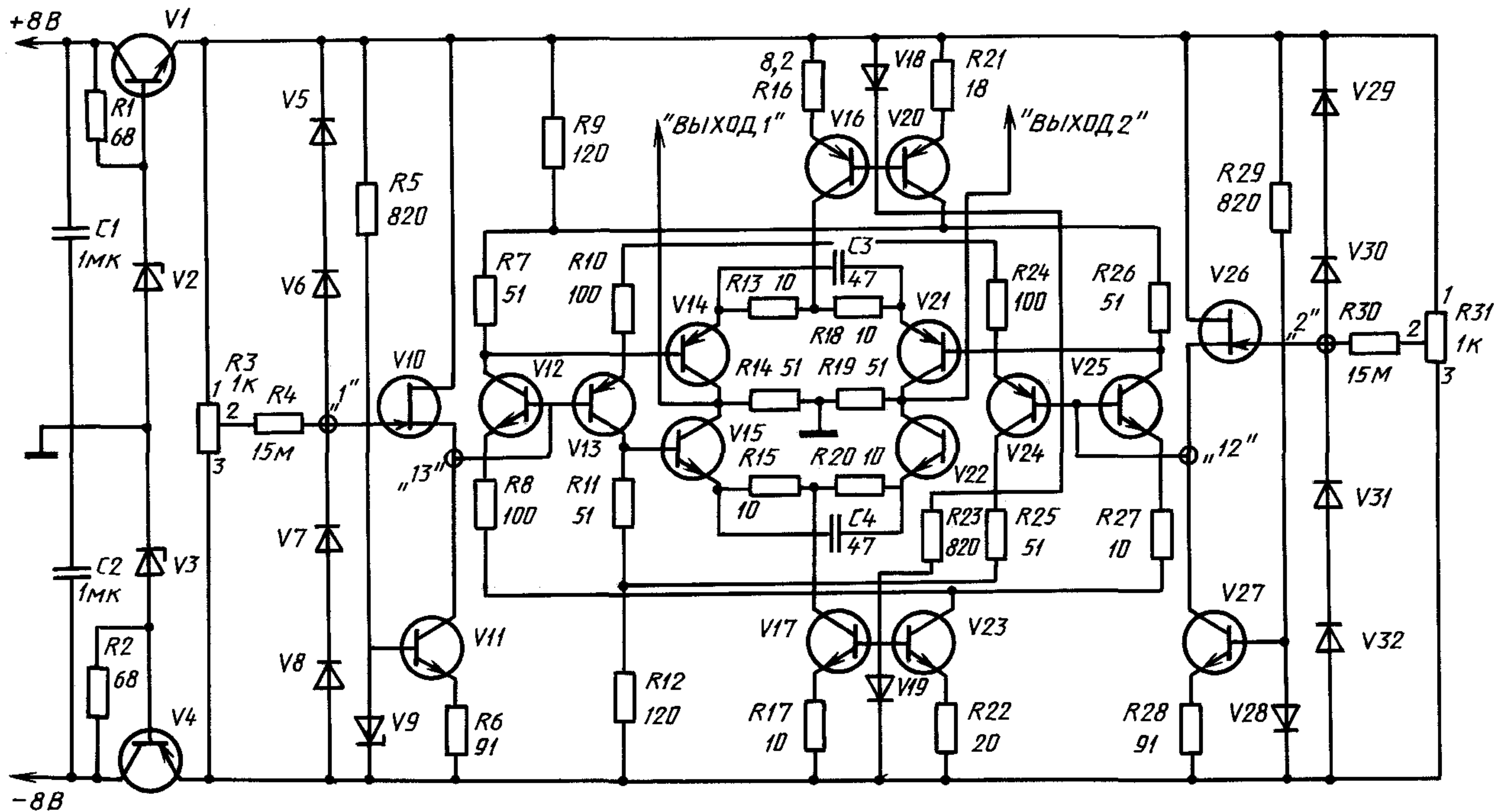
Схема электрическая принципиальная активной дипольной антенны
