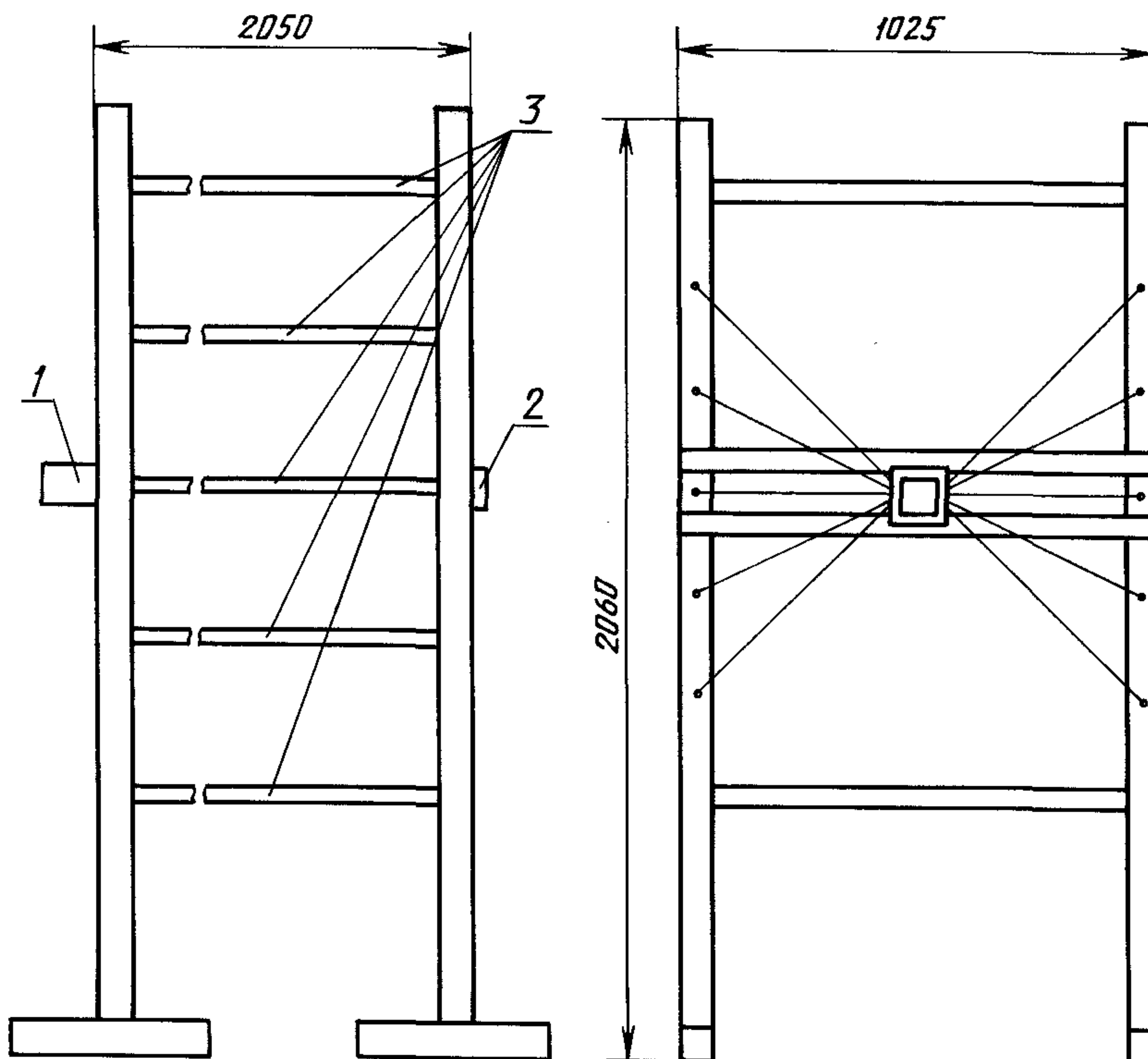
Общий вид Е-установки
