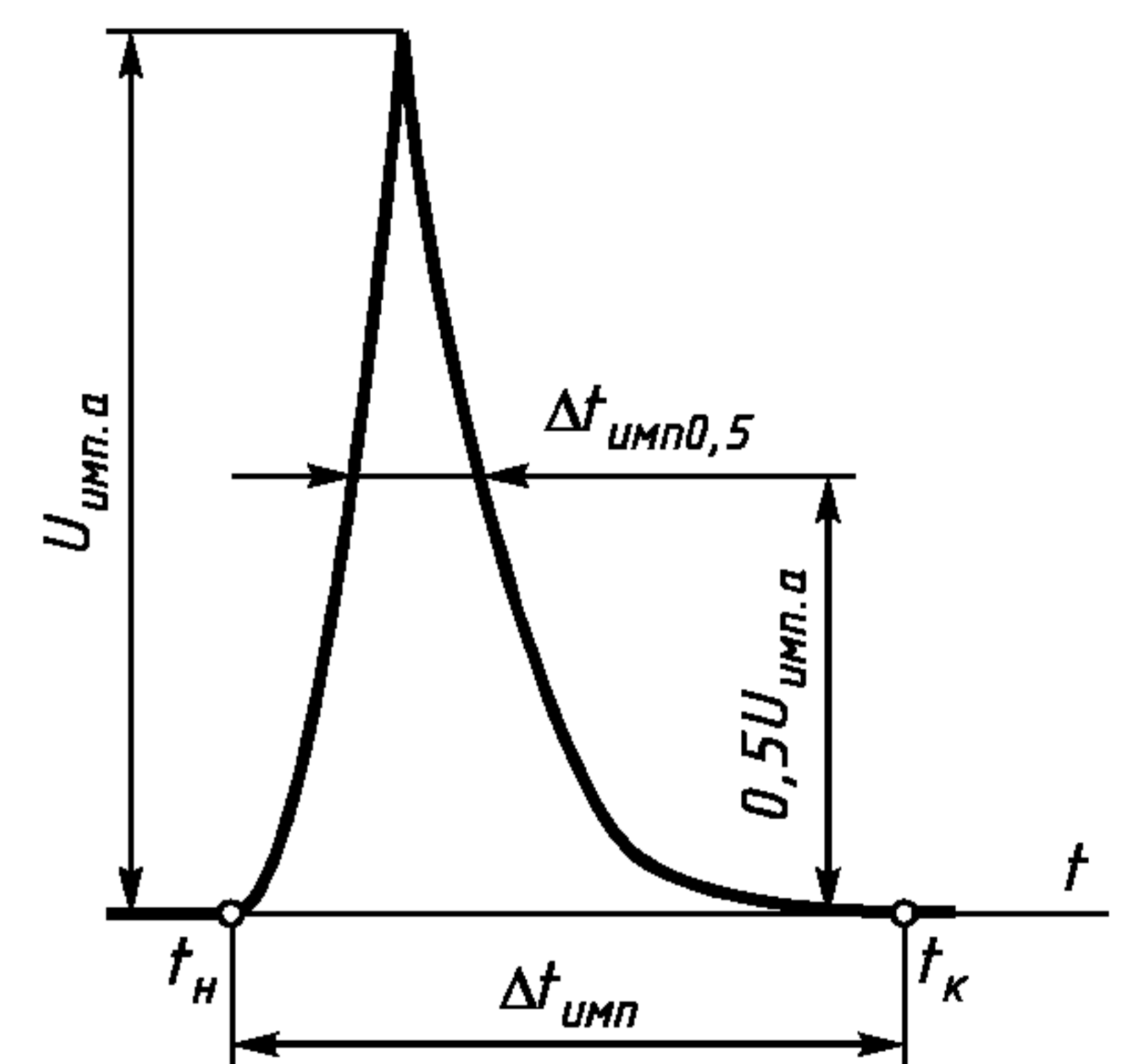
Рисунок Б.3 — Параметры импульсного напряжения
