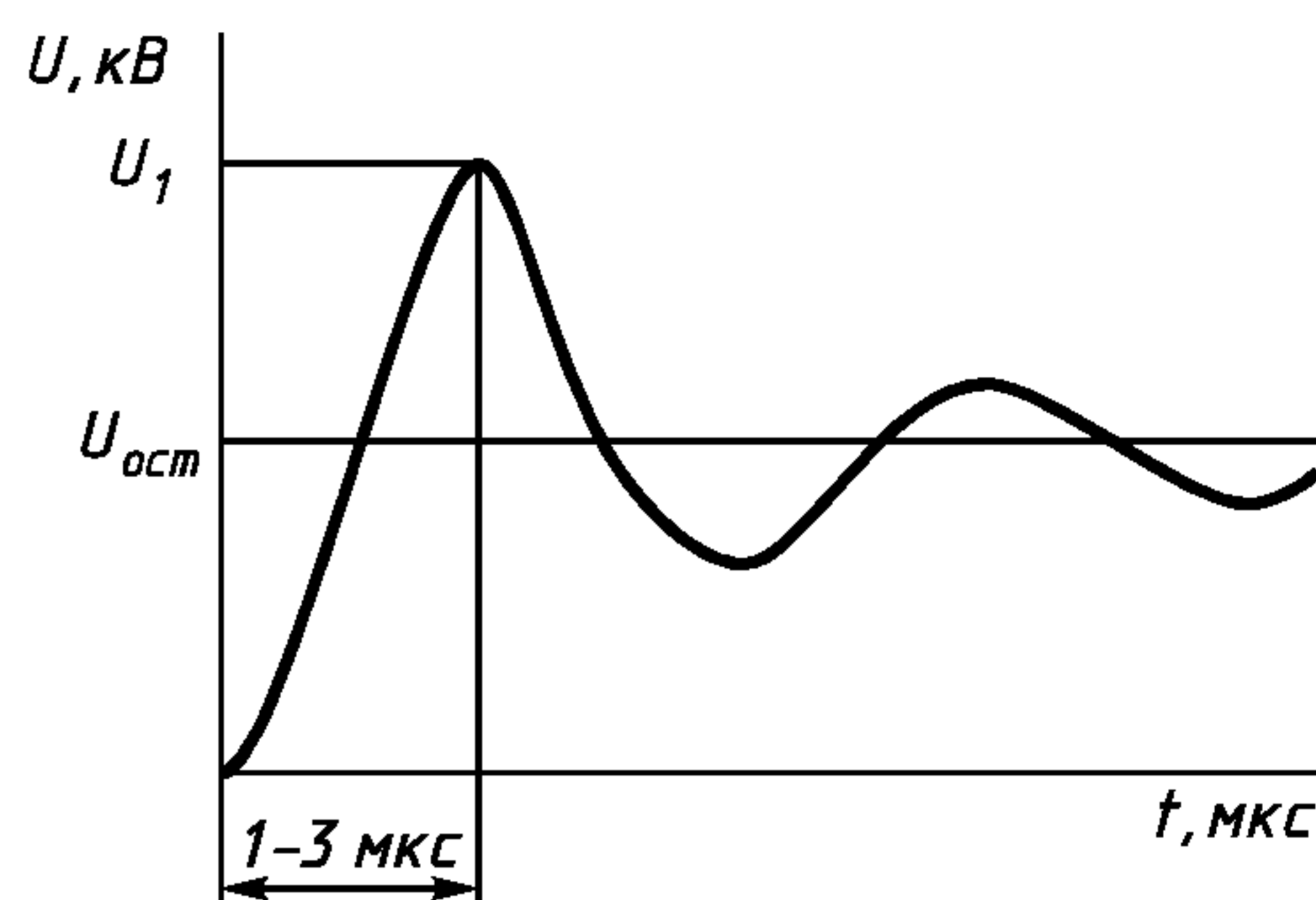
Рисунок Д.2 — Форма грозовых импульсов, характерная для точек присоединения a , в , г , д на рисунке Д.1.
