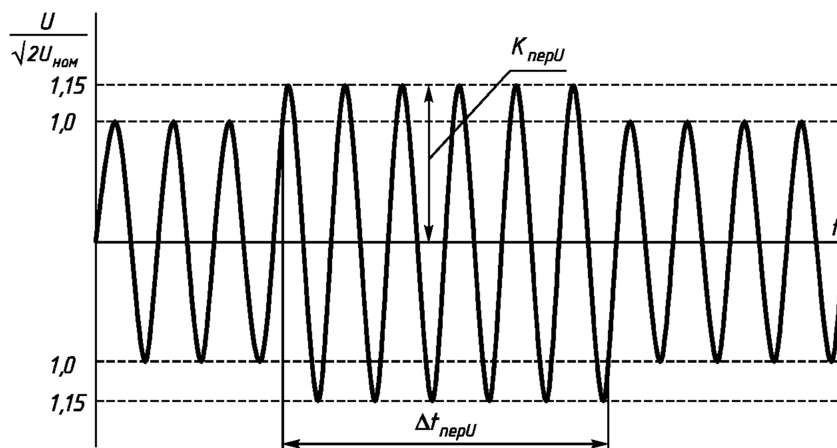
Рисунок Б.4 — Временное перенапряжение
