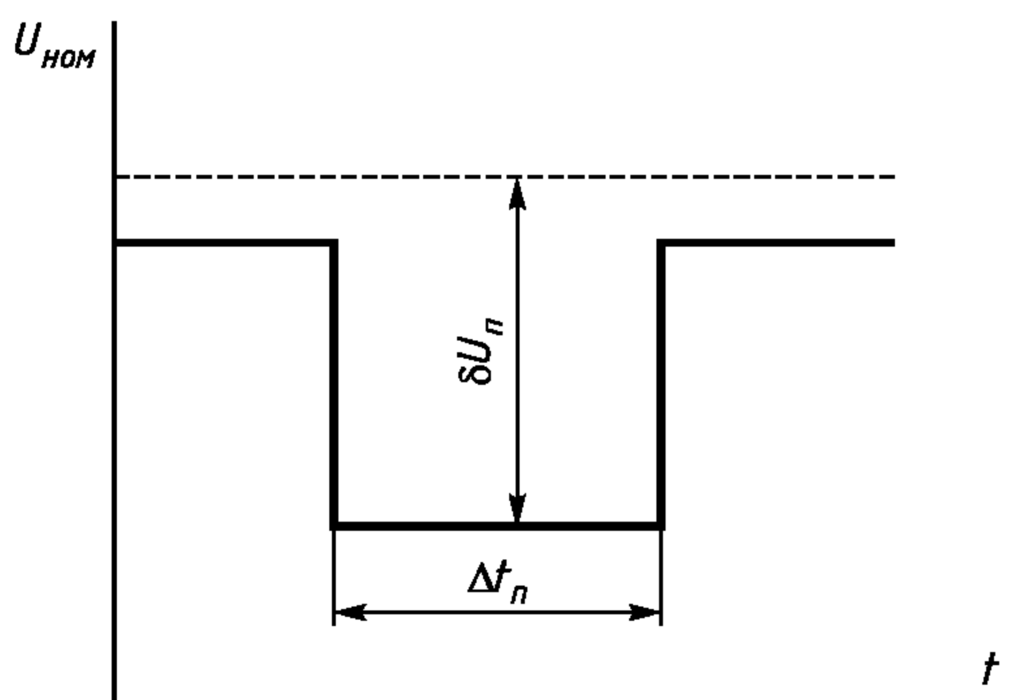
Рисунок Б.2 — Провал напряжения
