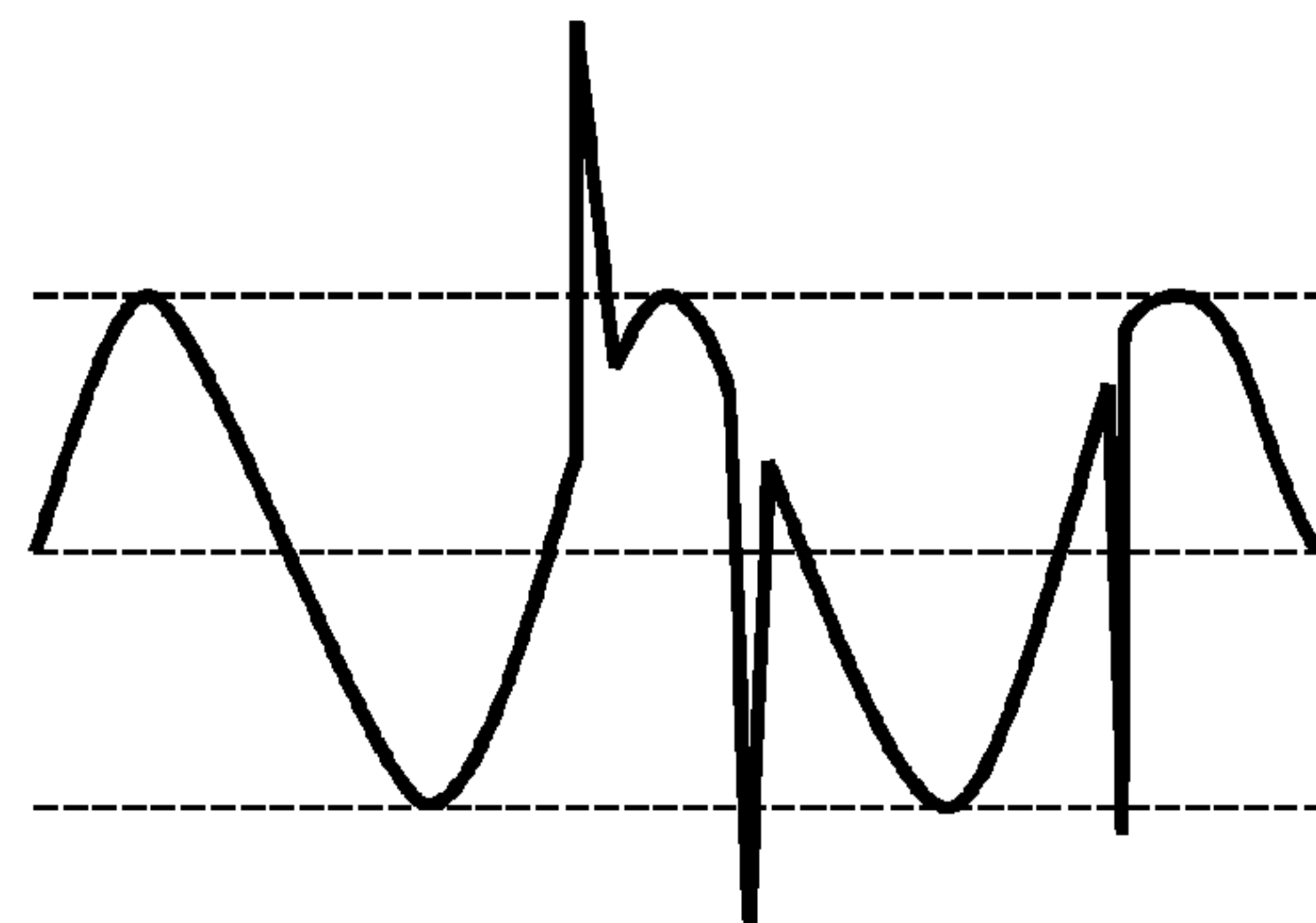
Рисунок А.3 — Импульсы напряжения
