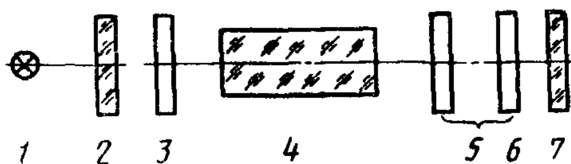
1 — источник излучения; 2 — матовое стекло, 3 — поляризатор, 4 — измеряемый образец оптического материала; 5 — компенсатор; 6 — анализатор, 7 — съемный светофильтр
