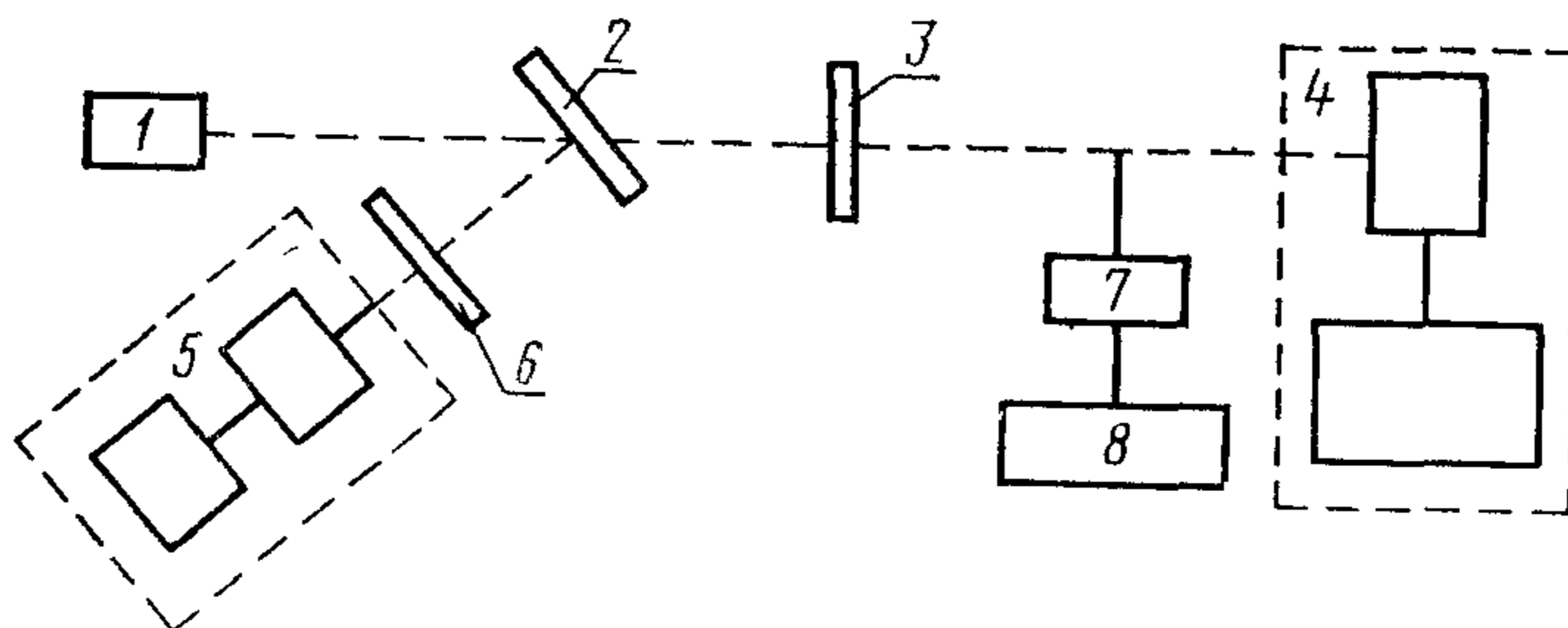
Схема установки для определения коэффициента преобразования (чувствительности) СИ ММ
