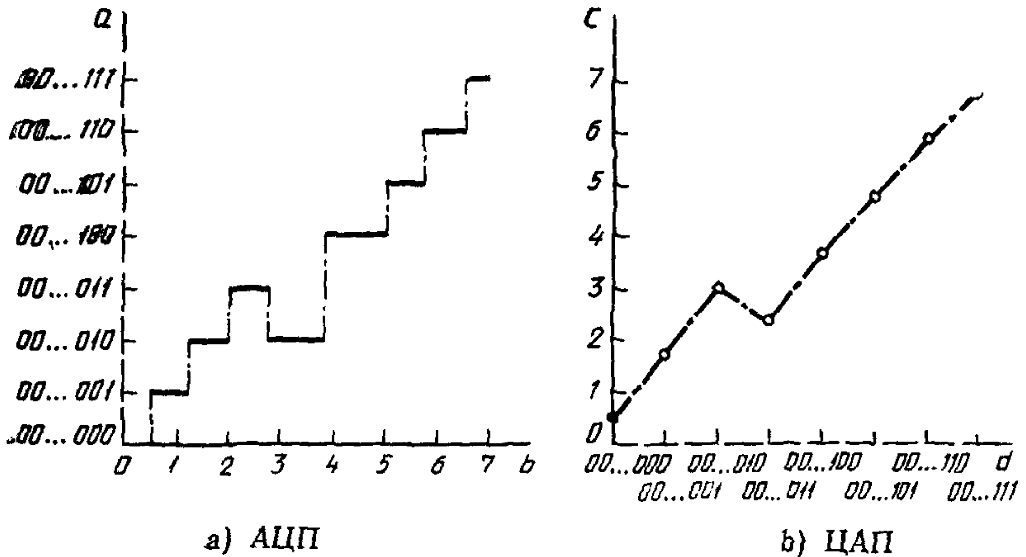
a) АЦП b) ЦАП a — цифровые выходные коды; b — аналоговые входные величины (LSB); c — аналоговые выходные величины (LSB); d — цифровые входные коды
