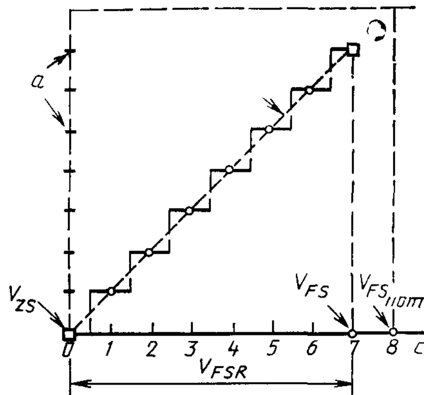
а) Однополярный АЦП
