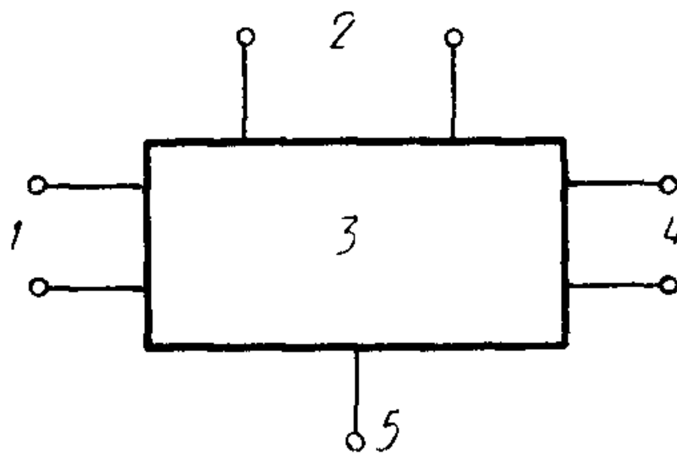
1 входы включая при необходимости входы сигнальная или управляющая 2 источники питания 3 интерфейсная интегральная схема 4 входы 5 — контрольный вывод
