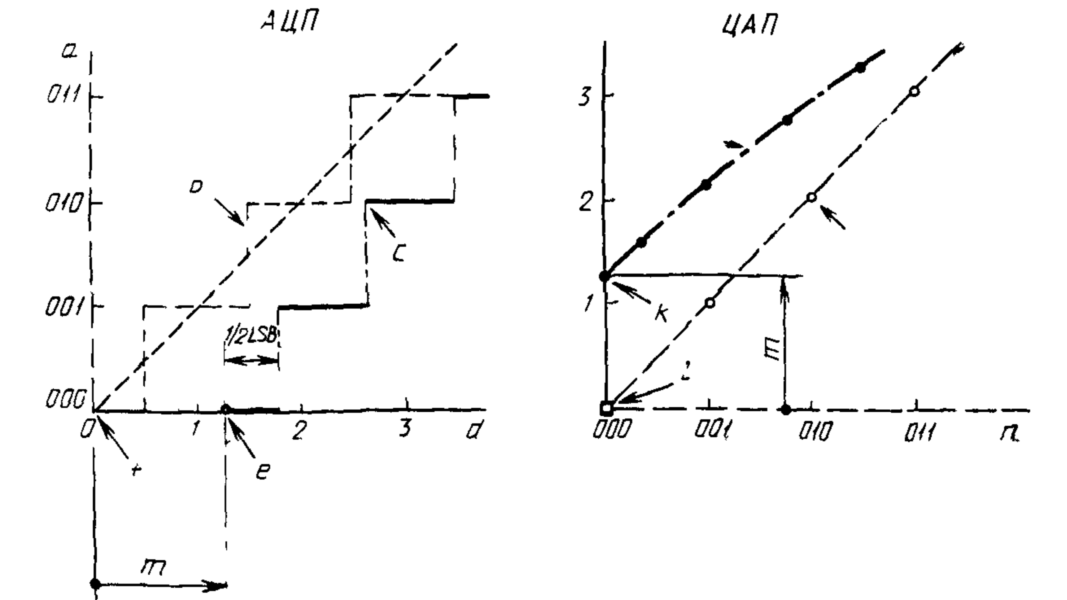
а) Смещение (указано для ступени 000)
