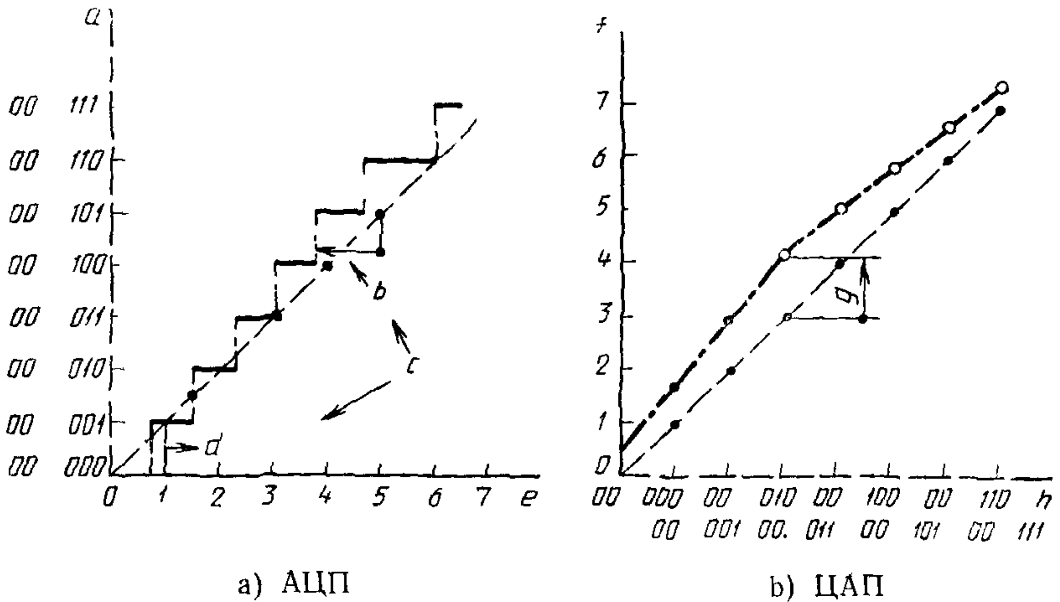
a) АЦП b) ЦАП a — цифровые выходные коды b — на ступени 00 101 ( -1 \frac{1}{4} LSB), c — полная погрешность, d — на ступени 00 001 ( +1 \frac{1}{2} LSB) e — аналоговые входные величины (LSB), f — аналоговые выходные величины (LSB), g — общая погрешность на ступени 00 011 ( +1 \frac{1}{2} LSB), h — цифровые входные коды
