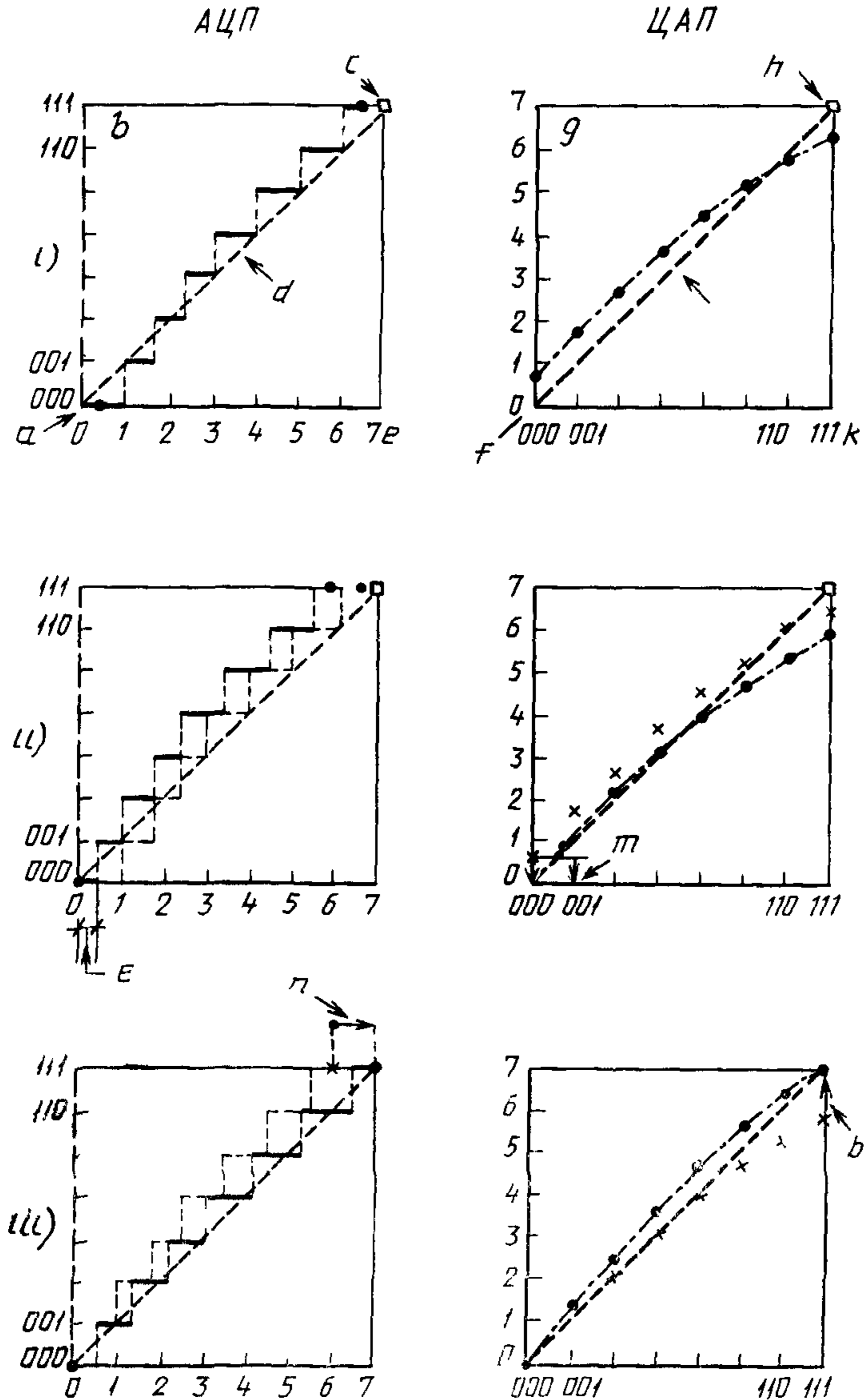
i) — до регулировки, ii) — после регулировки смещения, iii) — после регулировки смещения и коэффициента преобразования a , f — точки смещения, b — цифровые выходные коды h — точка наклона; d , l — идеальная прямая, e — аналоговые входные величины; g — аналоговые выходные величины k — цифровые входные коды l , m — регулировка смещения, n , p — регулировка коэффициента преобразования
