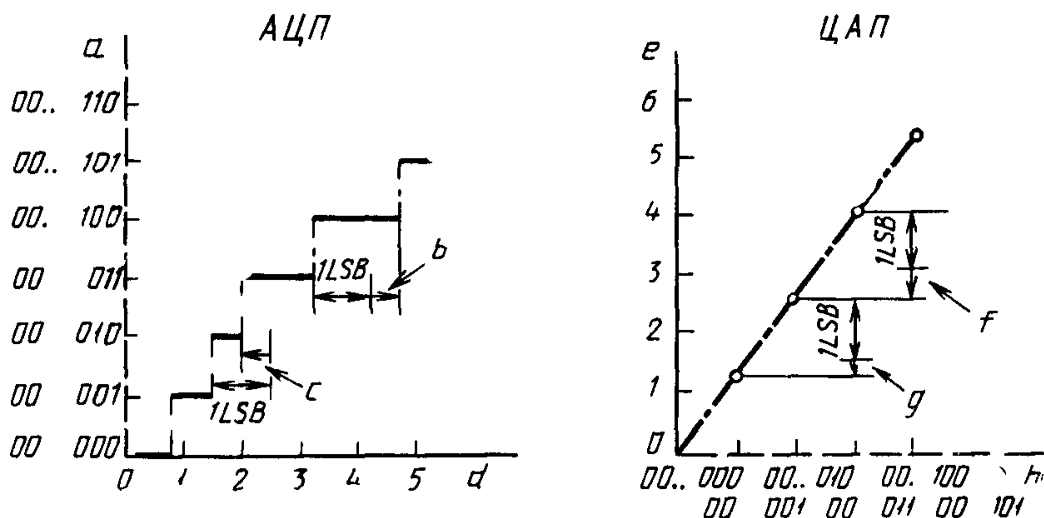
a — цифровые выходные коды; b, f — дифференциальная нелинейность ( +1/2 LSB), c — дифференциальная нелинейность ( +1/2 LSB); d — аналоговые входные величины (LSB); e — аналоговые выходные величины (LSB); g — дифференциальная нелинейность ( +1/4 LSB); h — цифровые входные коды
