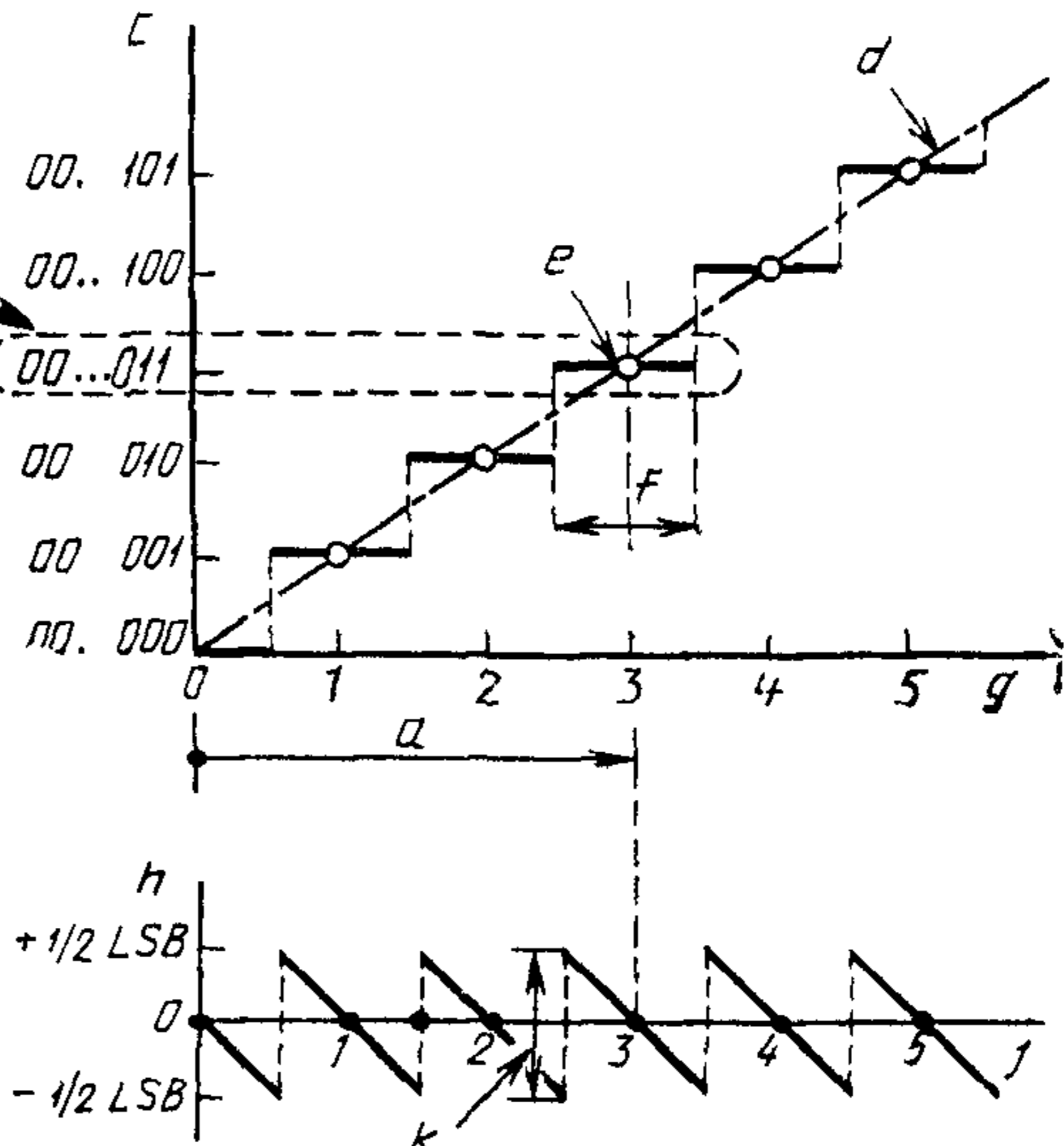
а) Идеальный линейный АЦП
