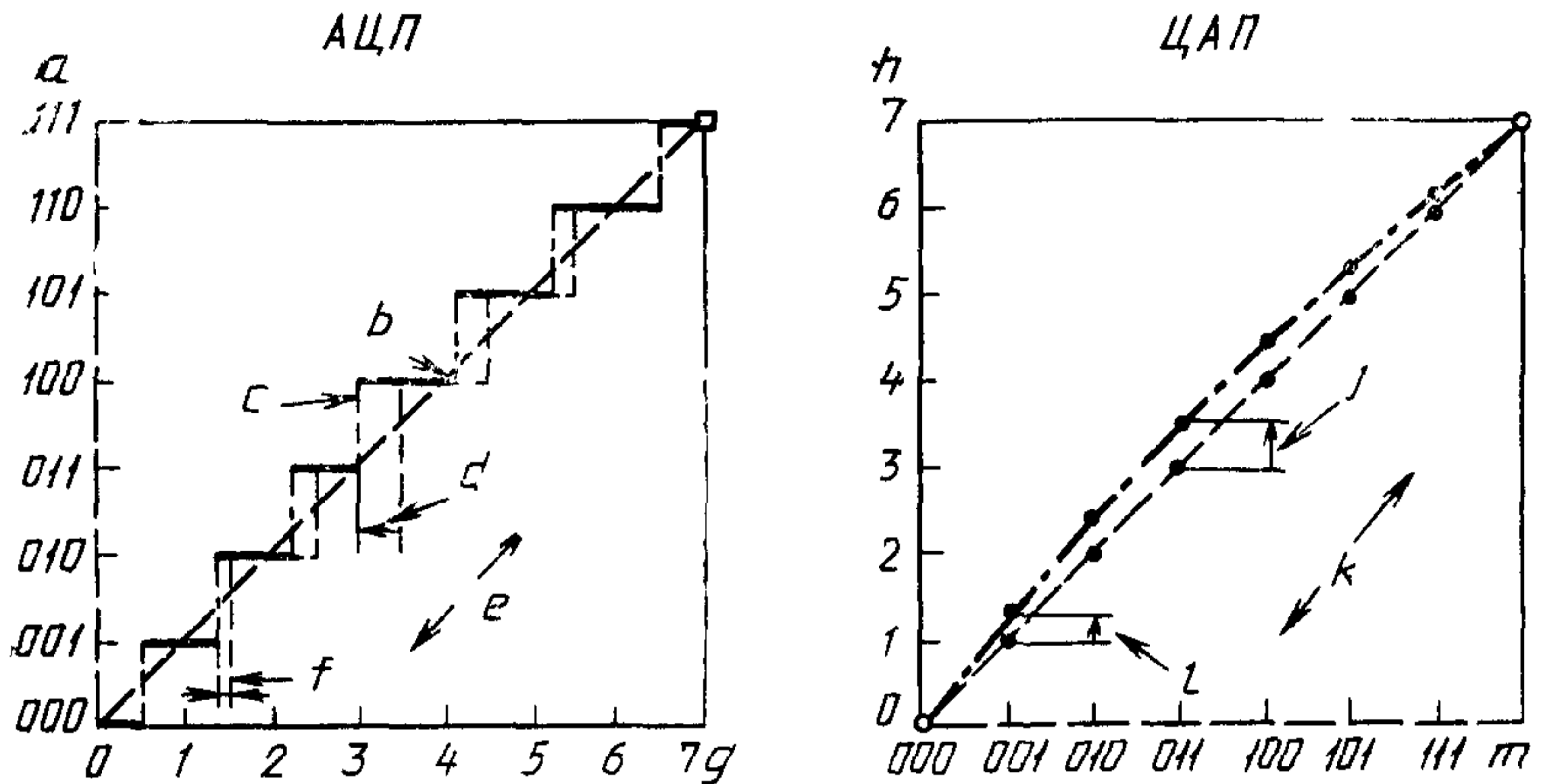
а) Нелинейность относительно прямой, проведенной через начальную и конечную точки характеристики преобразования АЦП или ЦАП (смещение и погрешность коэффициента преобразования сведены к нулю) a — цифровые выходные коды; b — идеальный переход; c — действительный переход; d — при переходе 011/100 ( -1/2 LSB); e , k — нелинейность относительно прямой, проведенной через начальную и конечную точки; f — при переходе 001/010 ( -1/8 LSB); g — аналоговые входные величины (LSB); h — аналоговые выходные величины (LSB), i — на ступени 011 ( +1/2 LSB); e — на ступени 001 ( +1/4 LSB); m — цифровые входные коды
