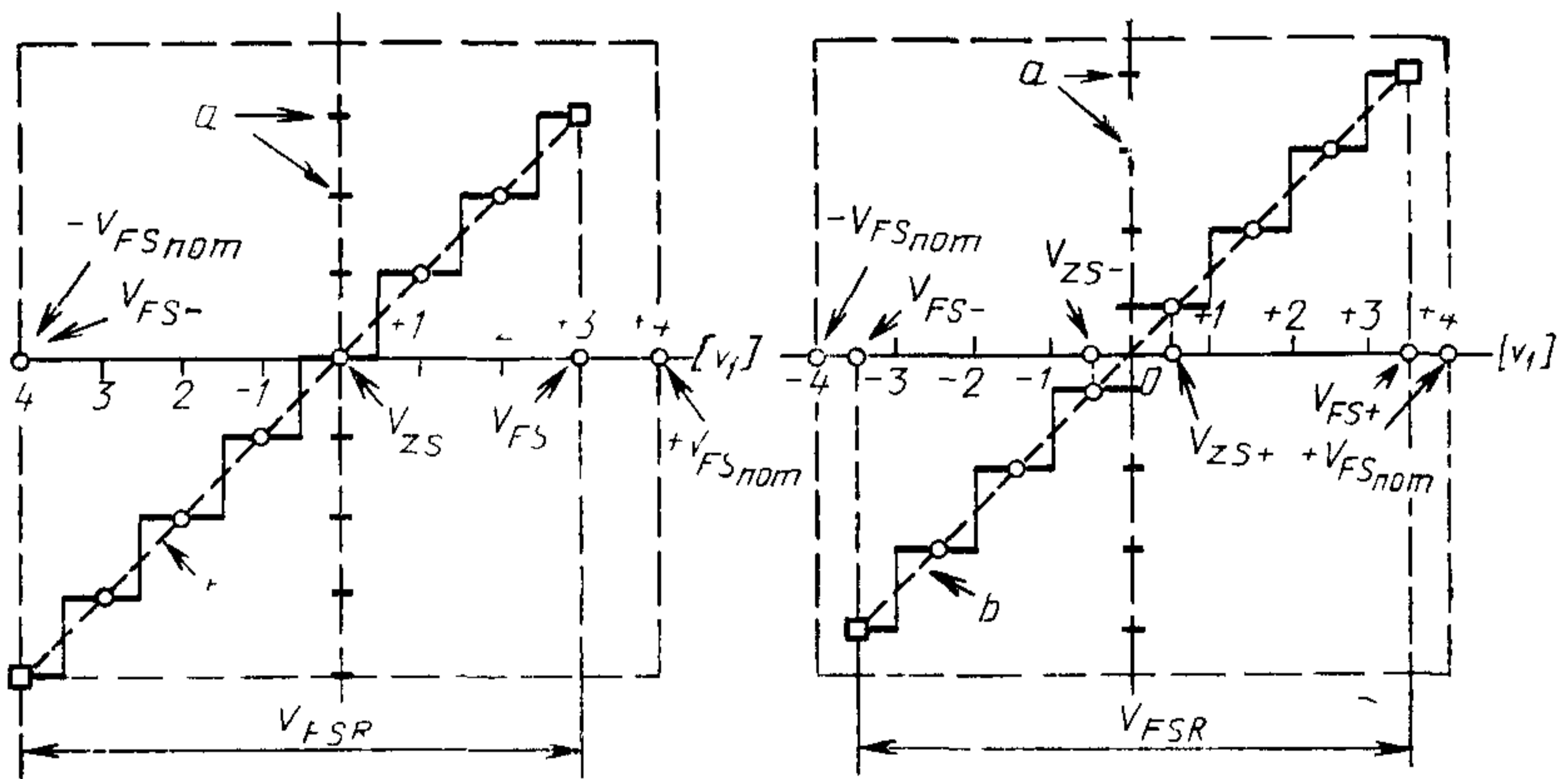
б) Биполярный АЦП с истинным нулем
