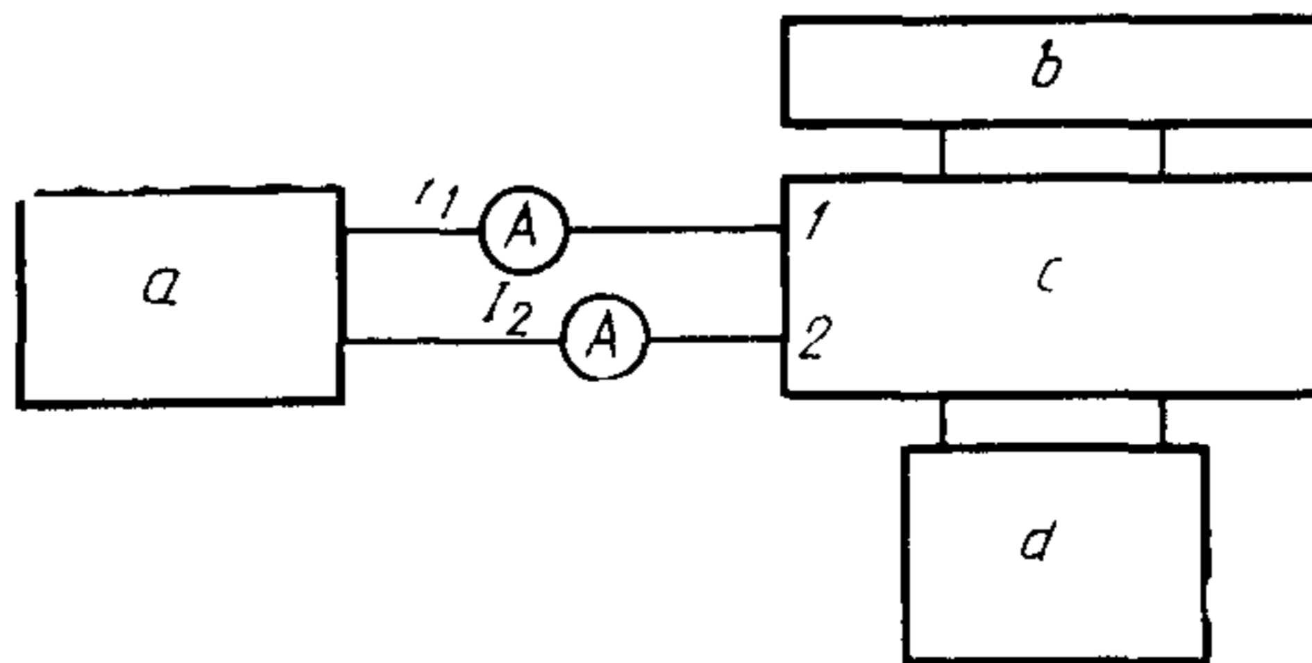
a — источники напряжения для V_{ID} и V_{IC} ; b — источники питания; c — измеряемая интегральная схема; d — дополнительные цепи
