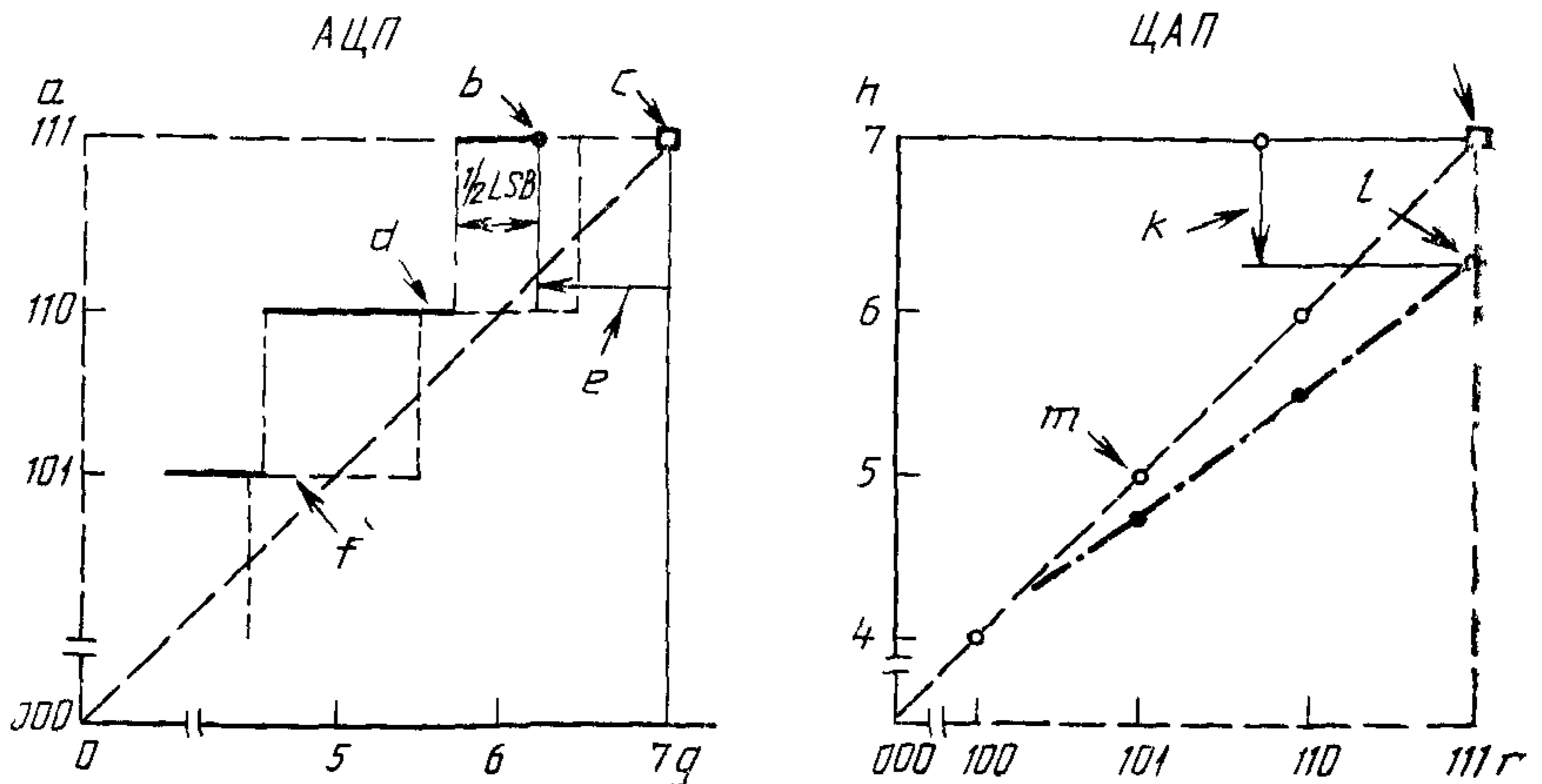
б) Погрешность коэффициента преобразования (после устранения смещения) (указано для ступени 111)
