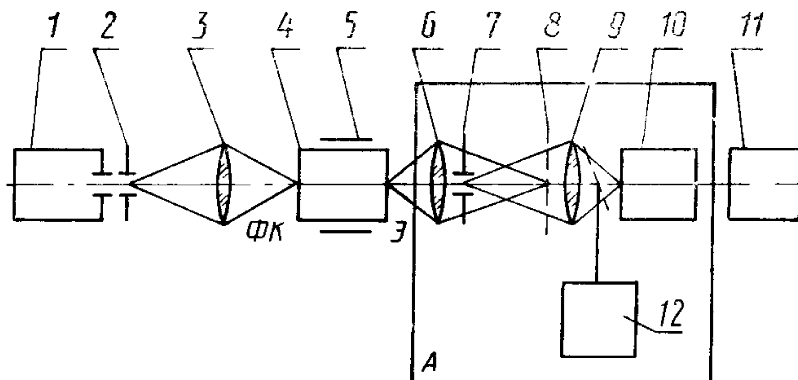
1 — осветитель; 2 — диафрагма со щелью; 3 — входная оптика (микрообъектив в обратном ходе); 4 — ЭОП; 5 — держатель ЭОП; 6 — выходной микрообъектив; 7 — выходной зрачок микрообъектива поз. 6; 8 — анализирующий растр; 9 — коллектив; 10 — приемник излучения, 11 — регистрирующее устройство; 12 — микроскоп; ФК — фотокатод; Э — экран; А — анализирующий блок
