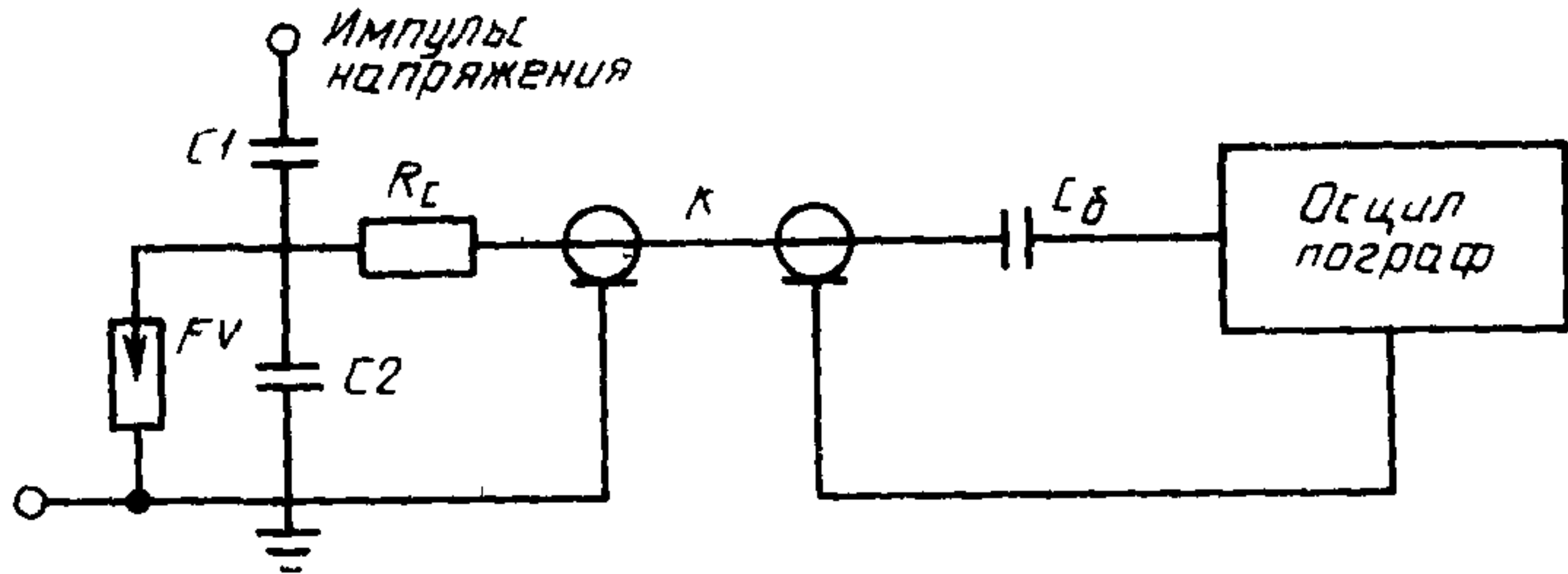
FV — разрядник; K — коаксиальный кабель; C_1 , C_2 — емкости высоковольтной и низковольтной частей делителя соответственно; C_б — блокировочный конденсатор; R_c — согласующее сопротивление
