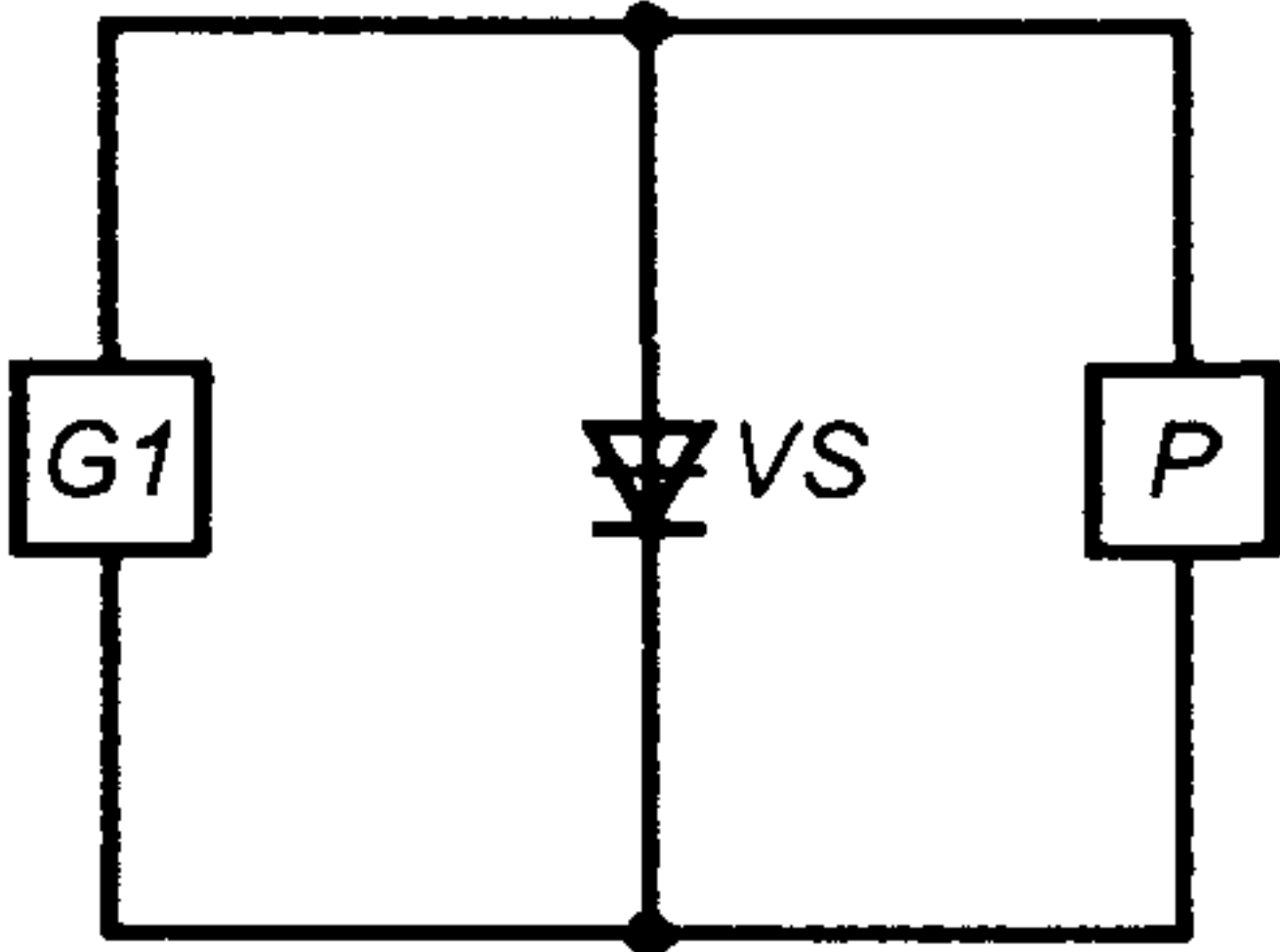
G1 — генератора отпирающих импульсов; P — измеритель временных интервалов; VS — испытуемый тиристор
