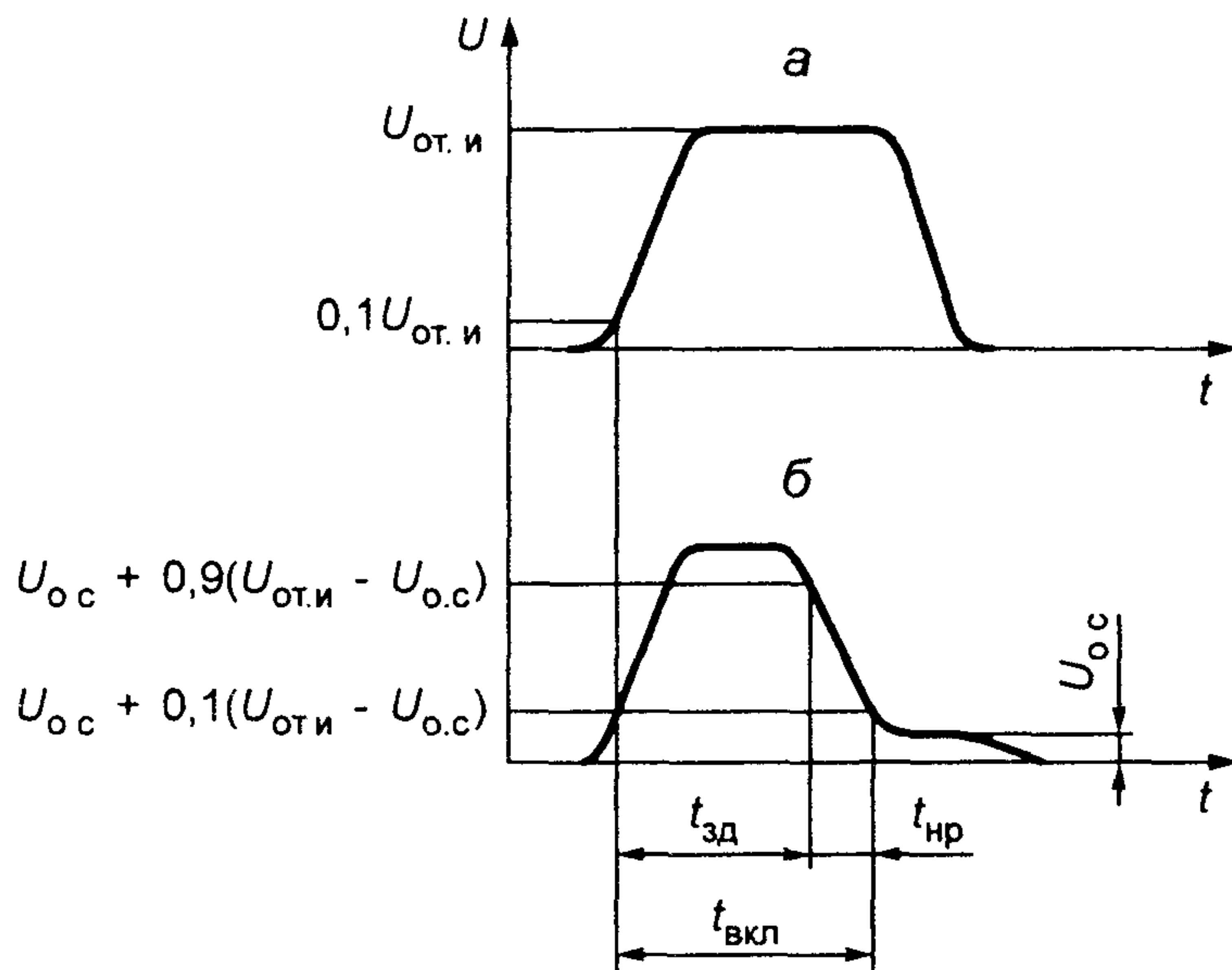
a — форма напряжения на выходе генератора G1 при отсутствии испытуемого тиристора; б — форма напряжения на испытуемом тиристоре; U_{о.с} — постоянное напряжение в открытом состоянии тиристора; U_{от.и} — импульсное отпирающее напряжение тиристора
