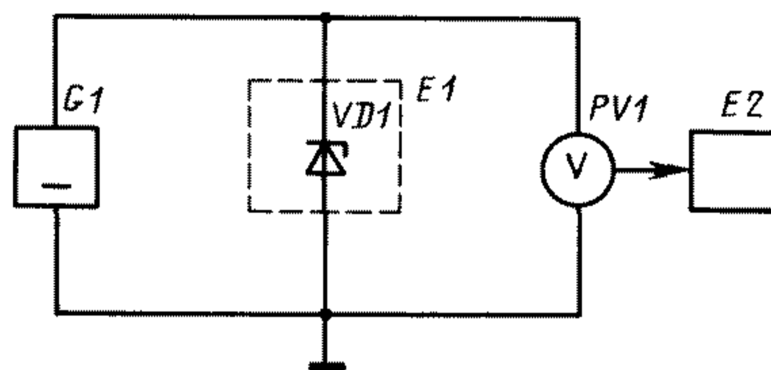
G1 — генератор постоянного тока; VD1 — измеряемый стабилитрон; E1 — термостат; PV1 — измеритель напряжения; E2 — регистрирующее устройство
