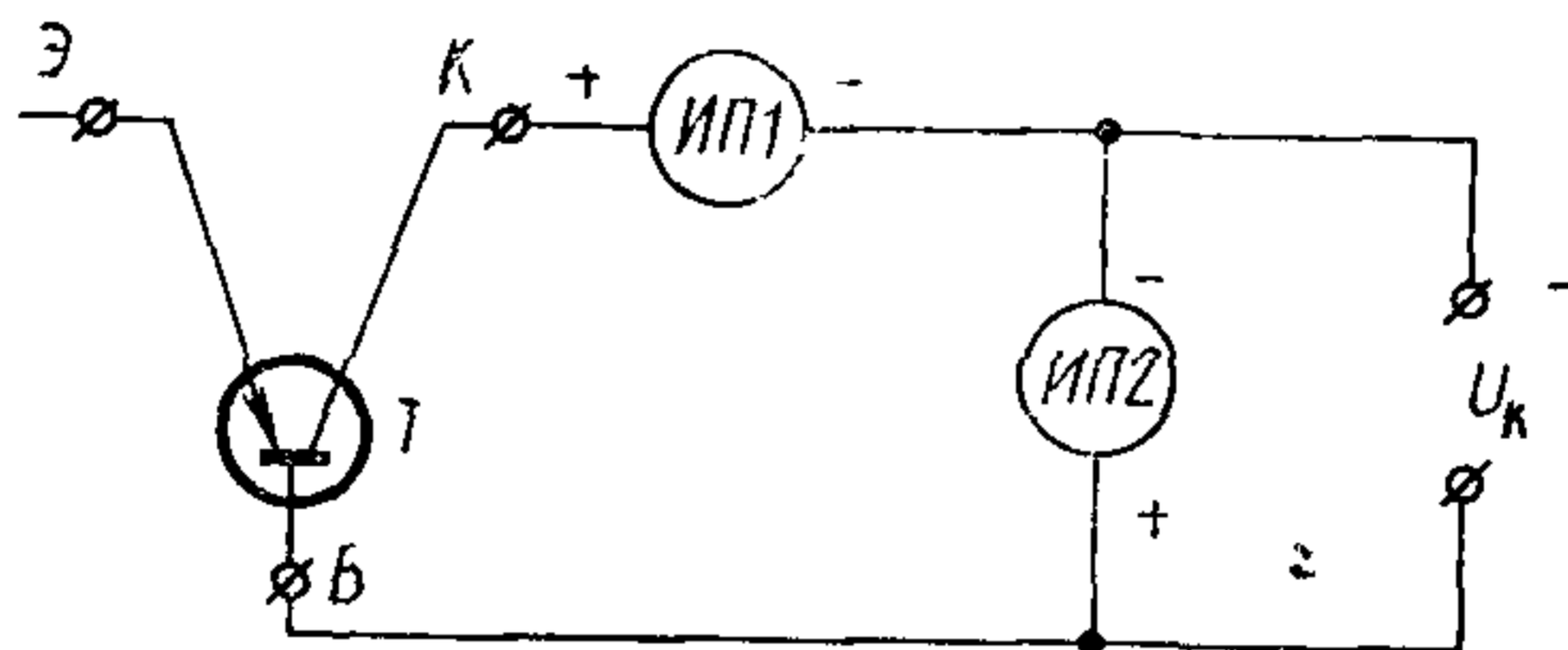
ИП1—измеритель постоянного тока, ИП2—измеритель постоянного напряжения, U_{К} —напряжение источника питания коллектора, Т—испытуемый транзистор
