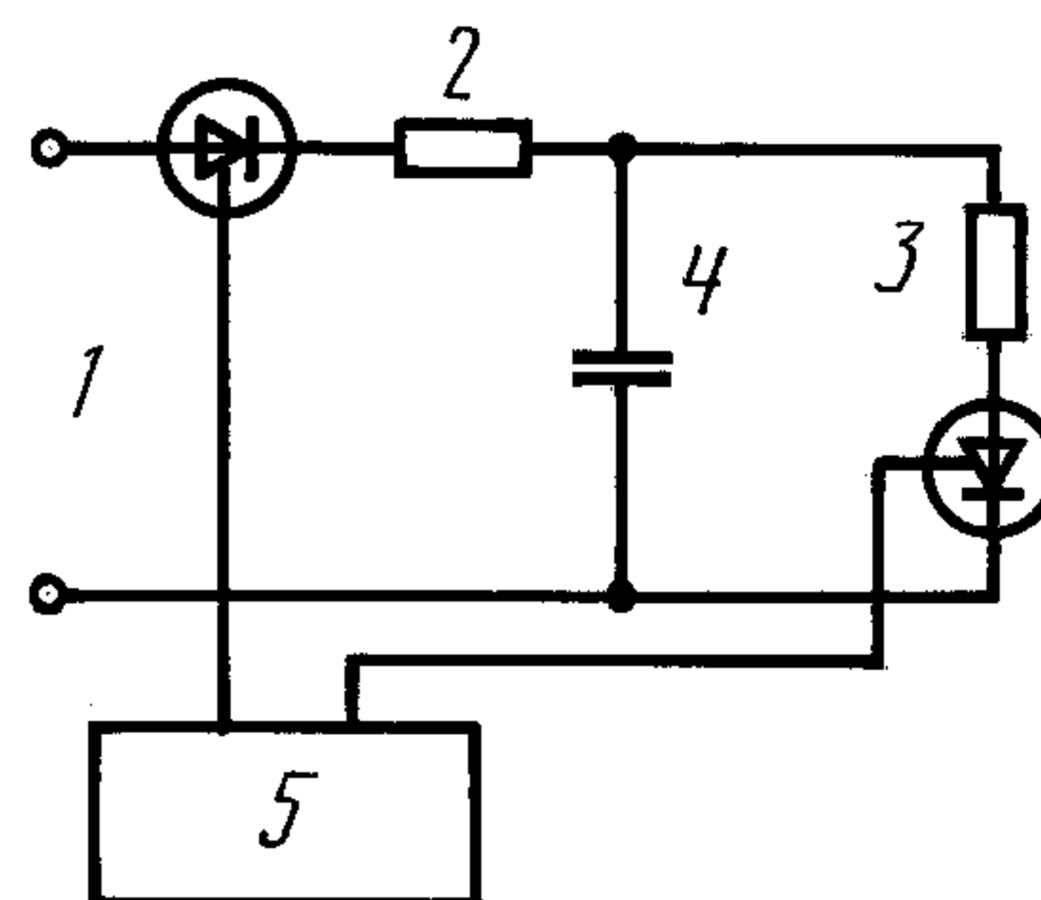
Тиристорная схема
