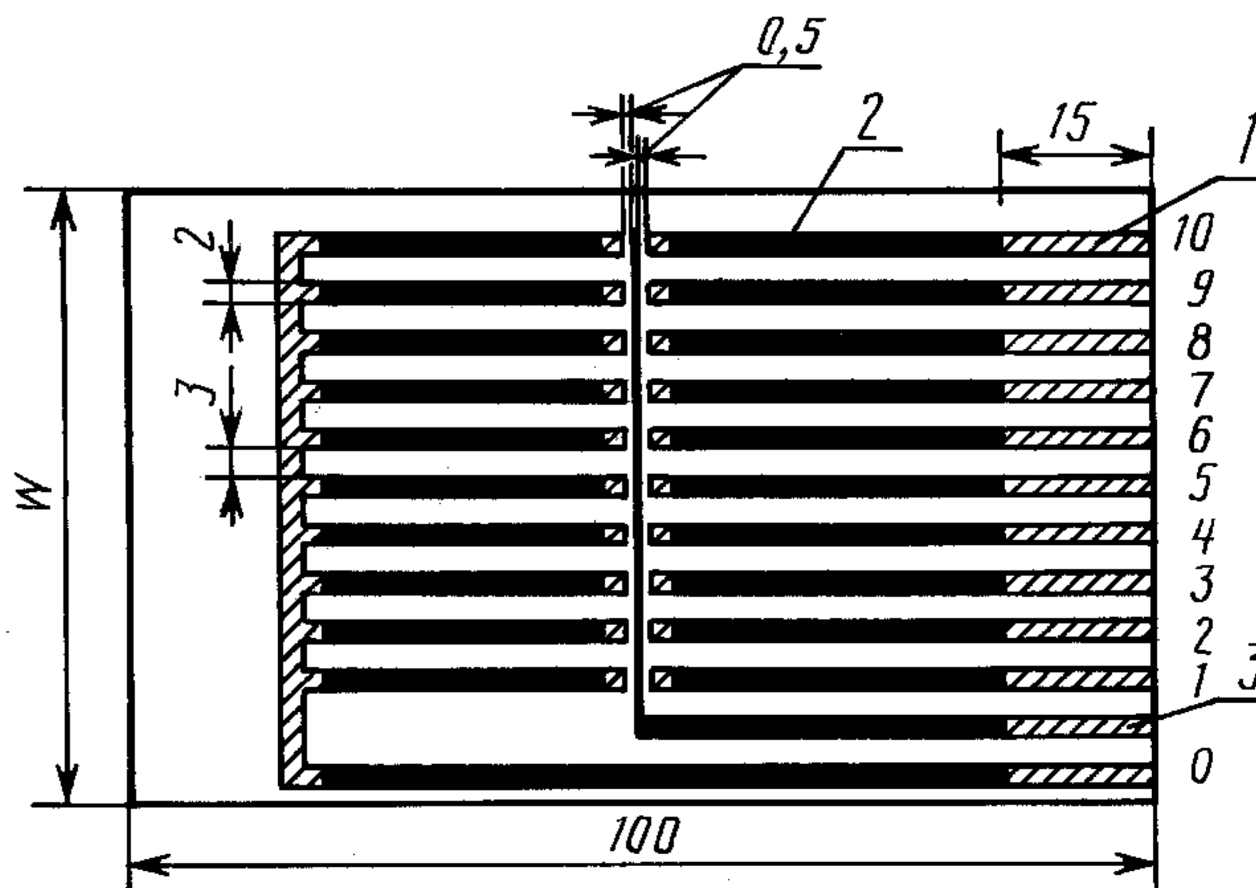
Подложка для механических и электрических испытаний
