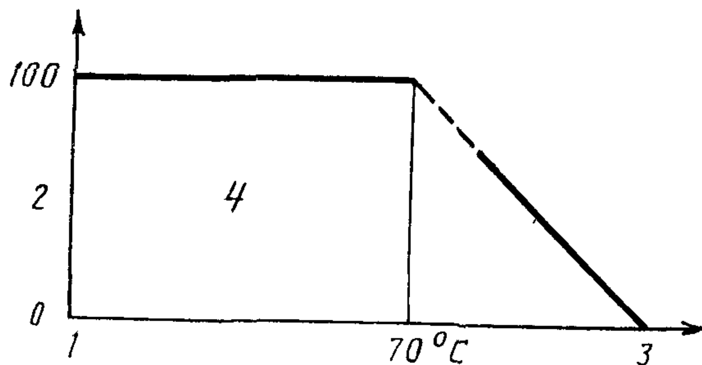
1 — нижнее значение температуры категории, 2 — процент номинальной мощности рассеяния; 3 — верхнее значение температуры категории, 4 — рекомендуемая зона эксплуатации
