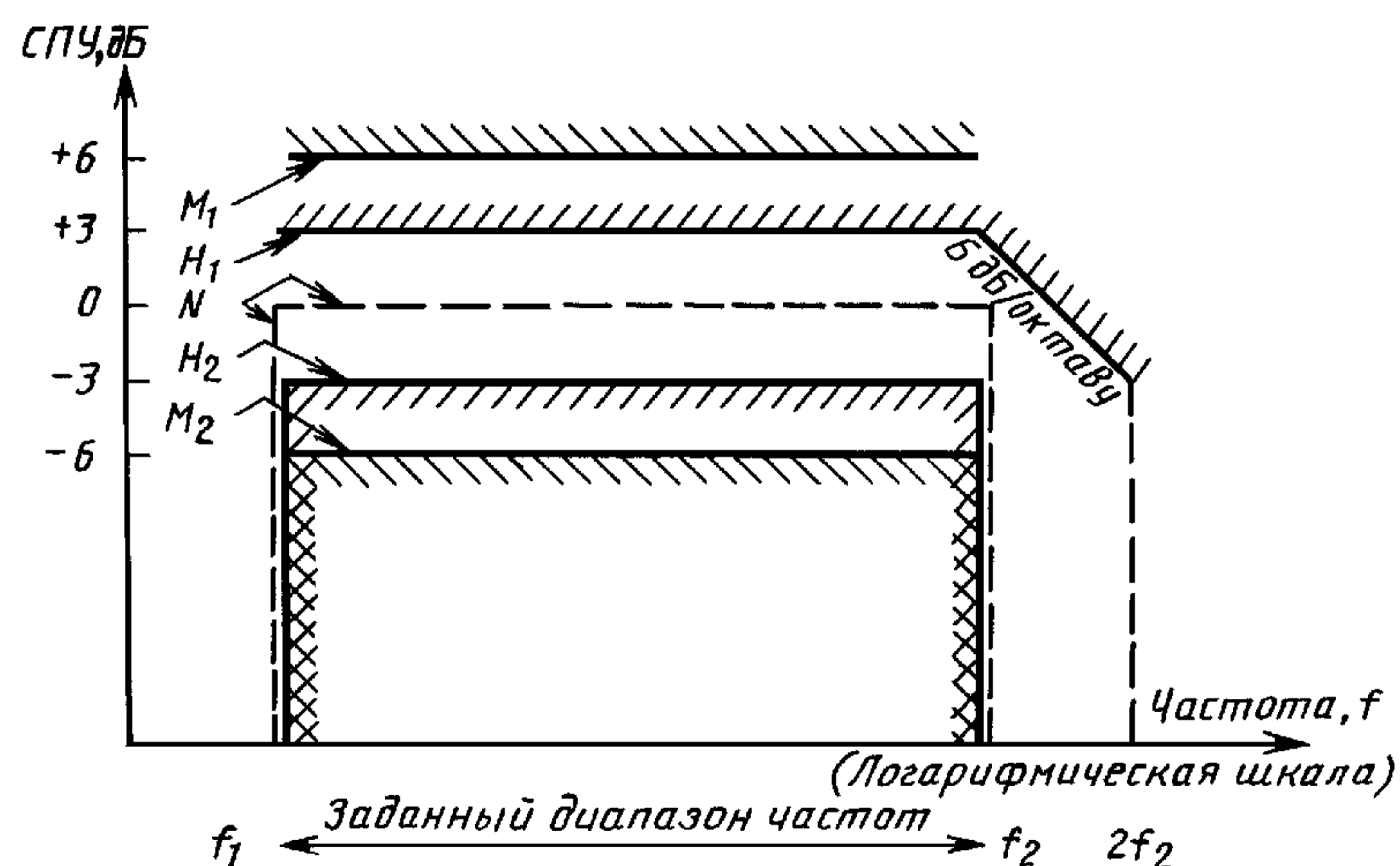
Спектр плотности ускорения (СПУ) и границы допусков
