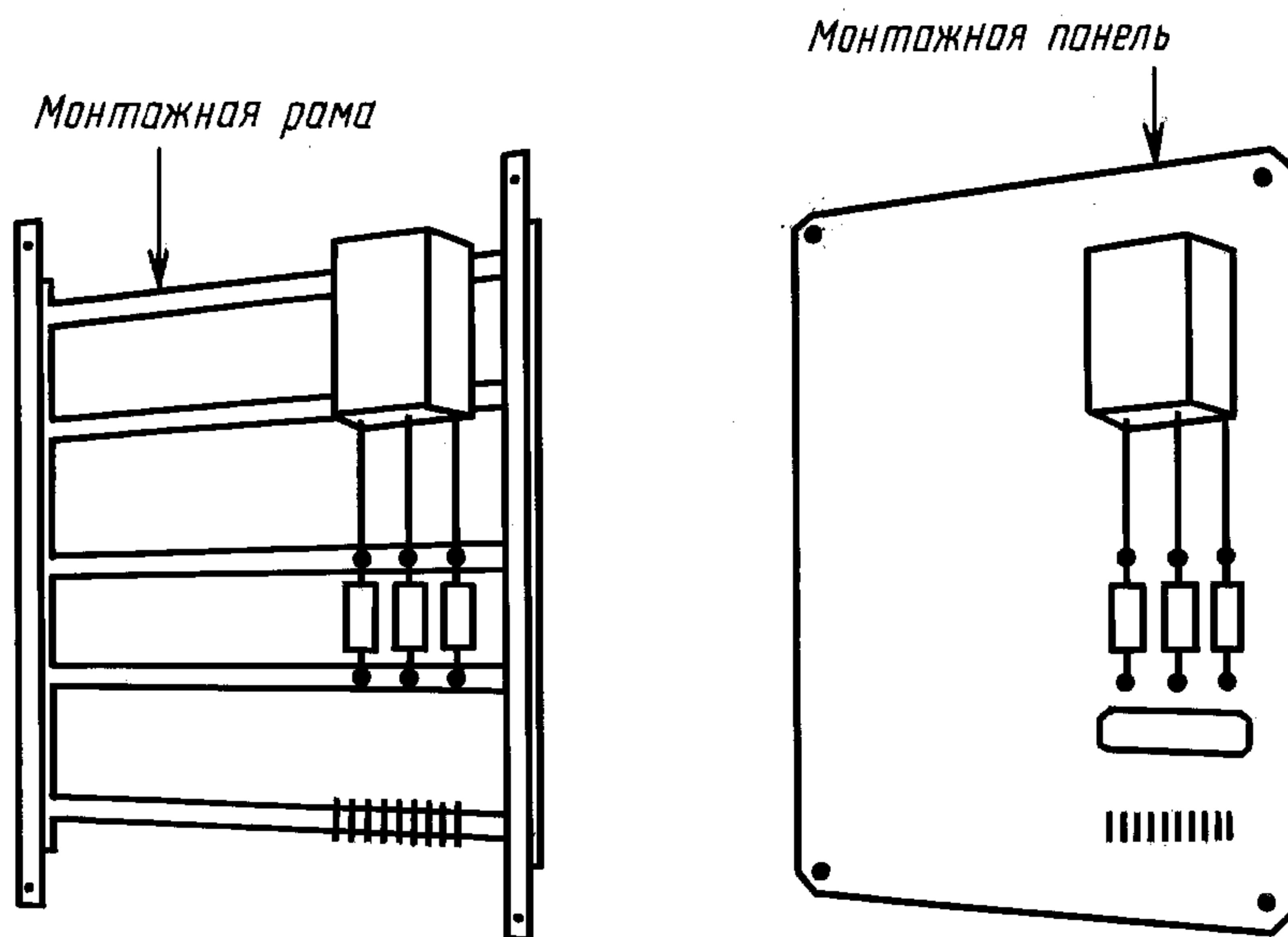
Неподвижные части
