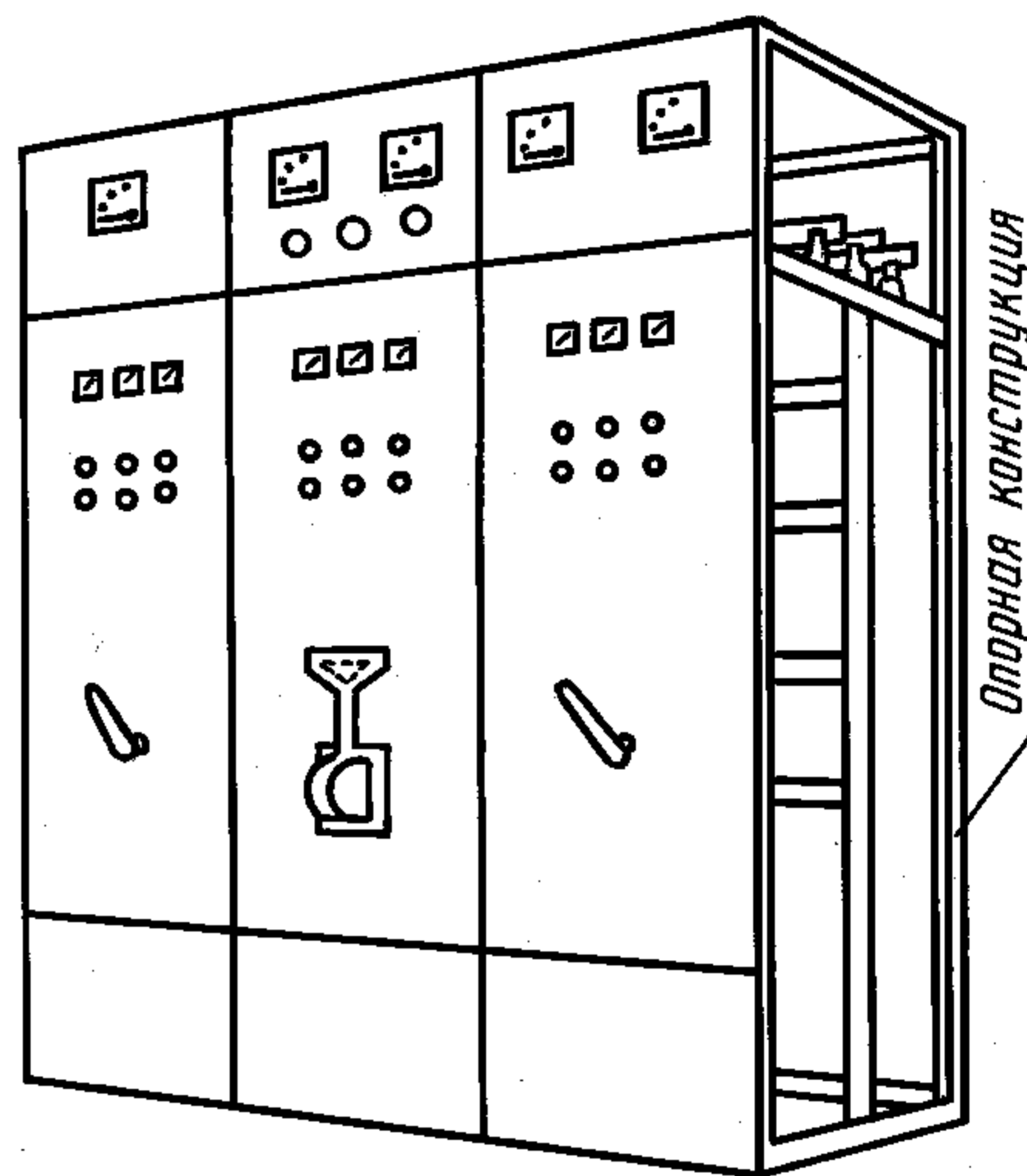
НКУ заводского изготовления открытого типа, защищенное спереди Черт. С.2
