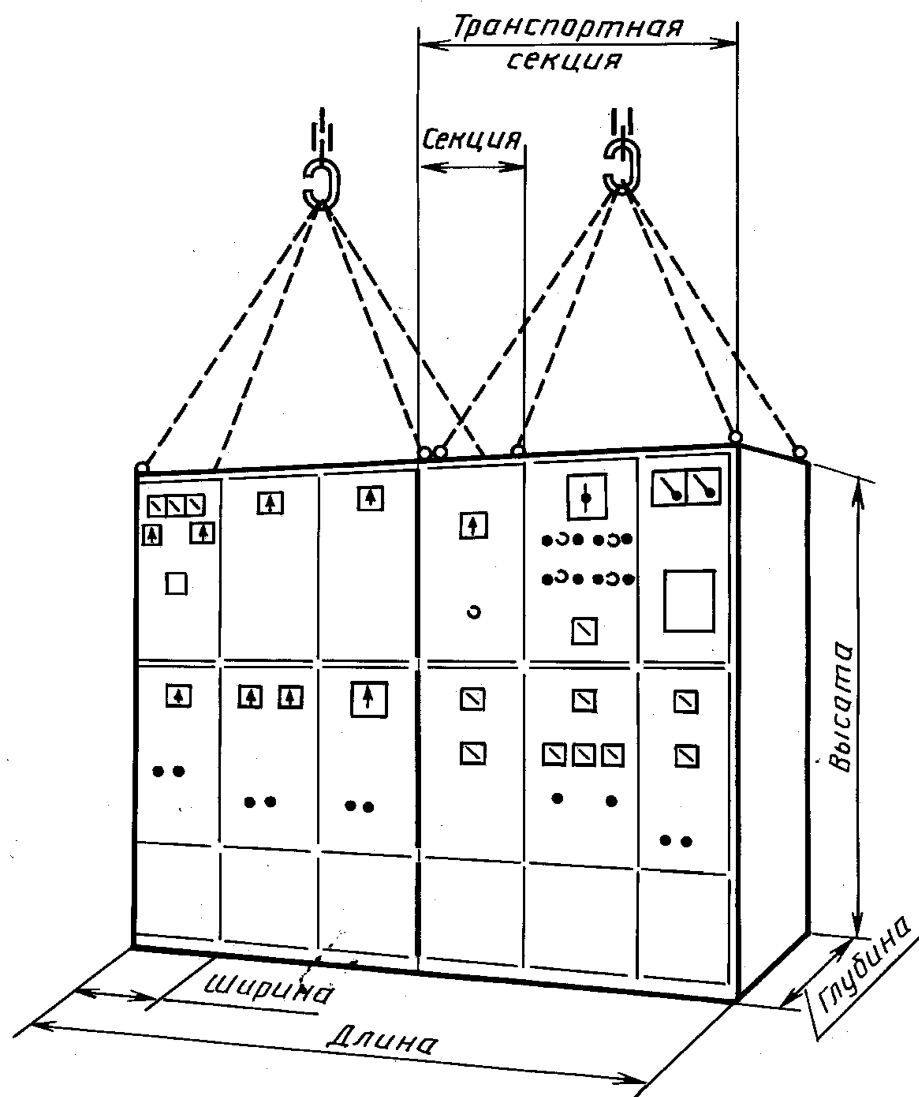
НКУ заводского изготовления многошкафного типа Черт. С.4
