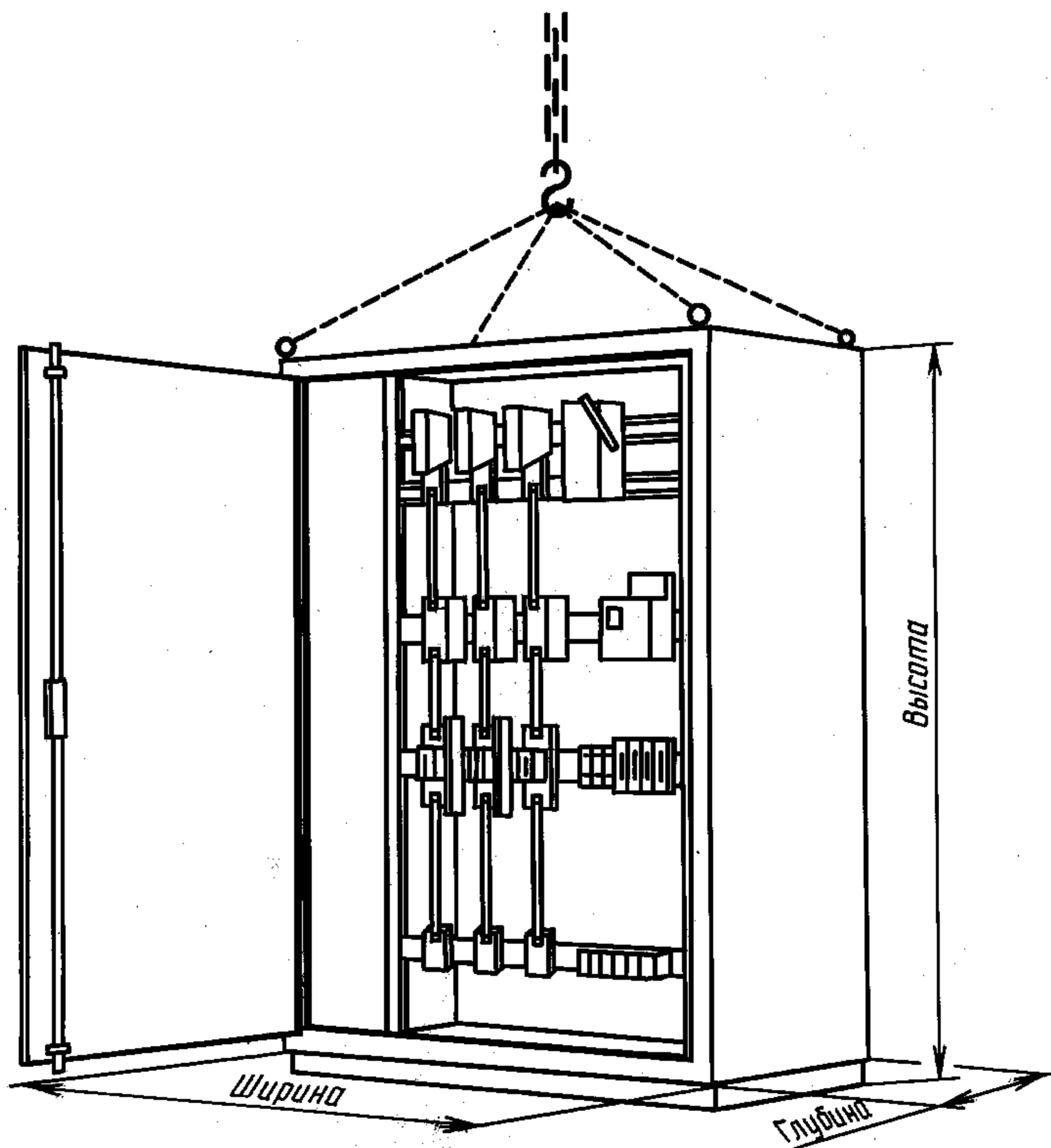
НКУ заводского изготовления шкафного типа Черт. С.3
