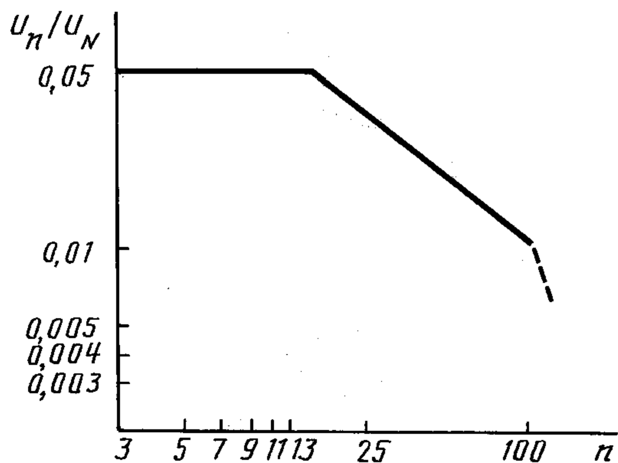
Максимально допустимая гармоническая составляющая номинального напряжения сети
