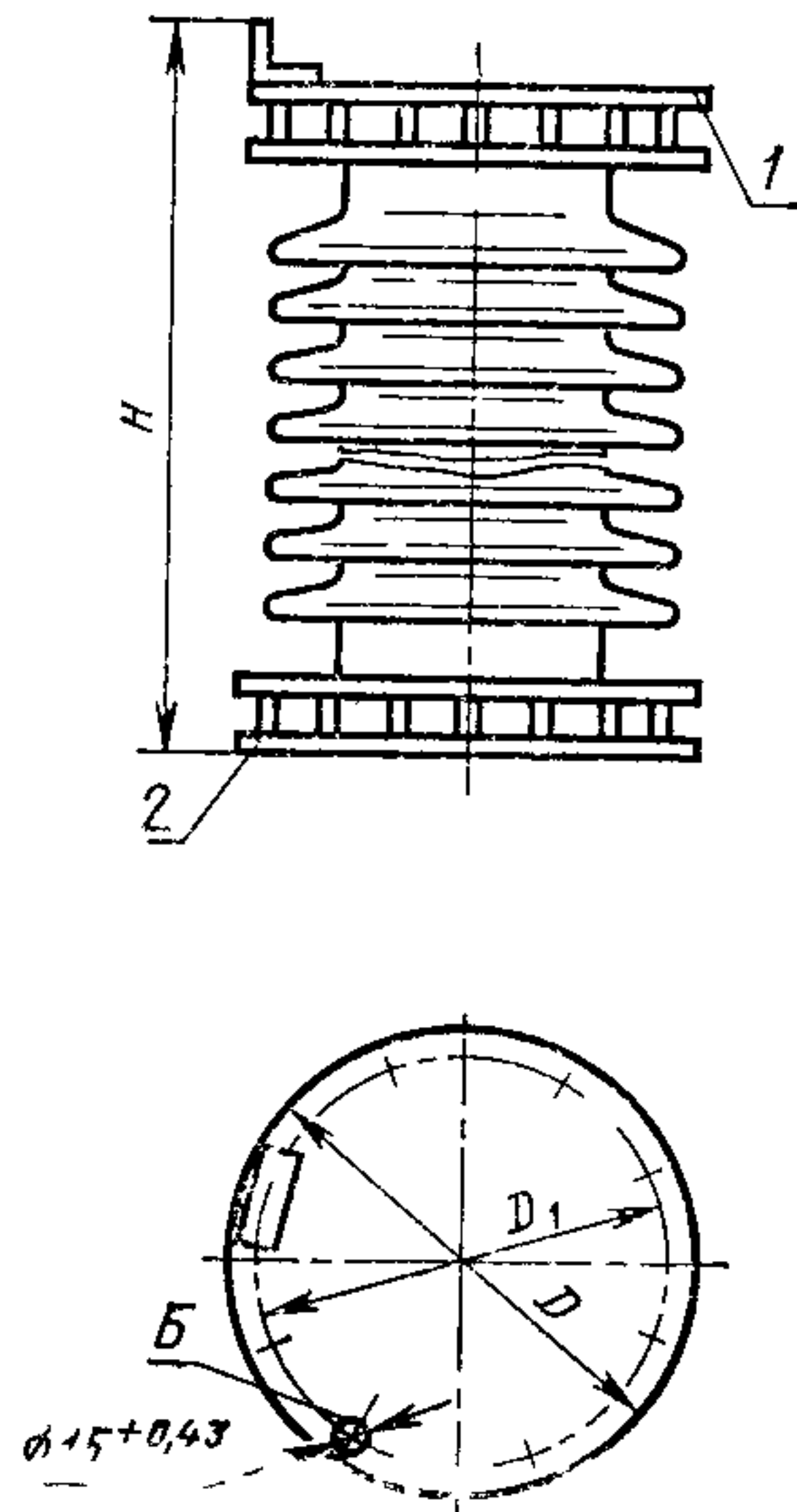
1—2 — выводы (крышки) Черт. 4
