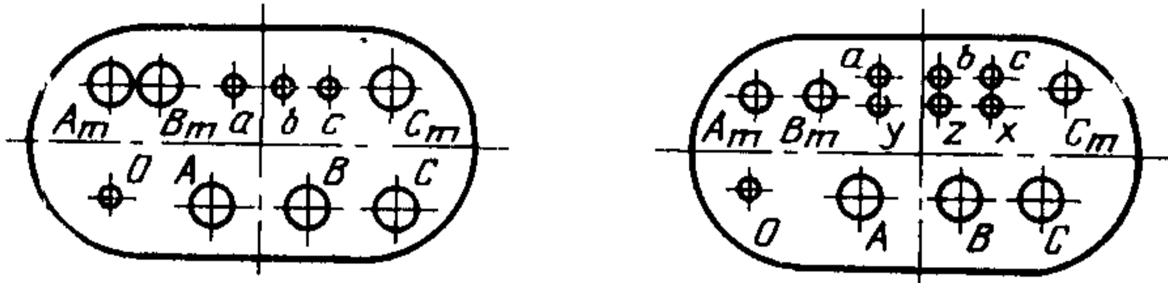
а) класс напряжения 220 кВ
