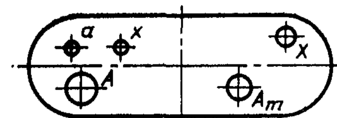
а) автотрансформатор АОДЦТН-267000/750/220
