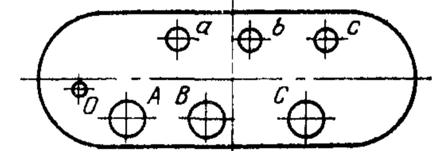
б) класс напряжения 500 кВ
