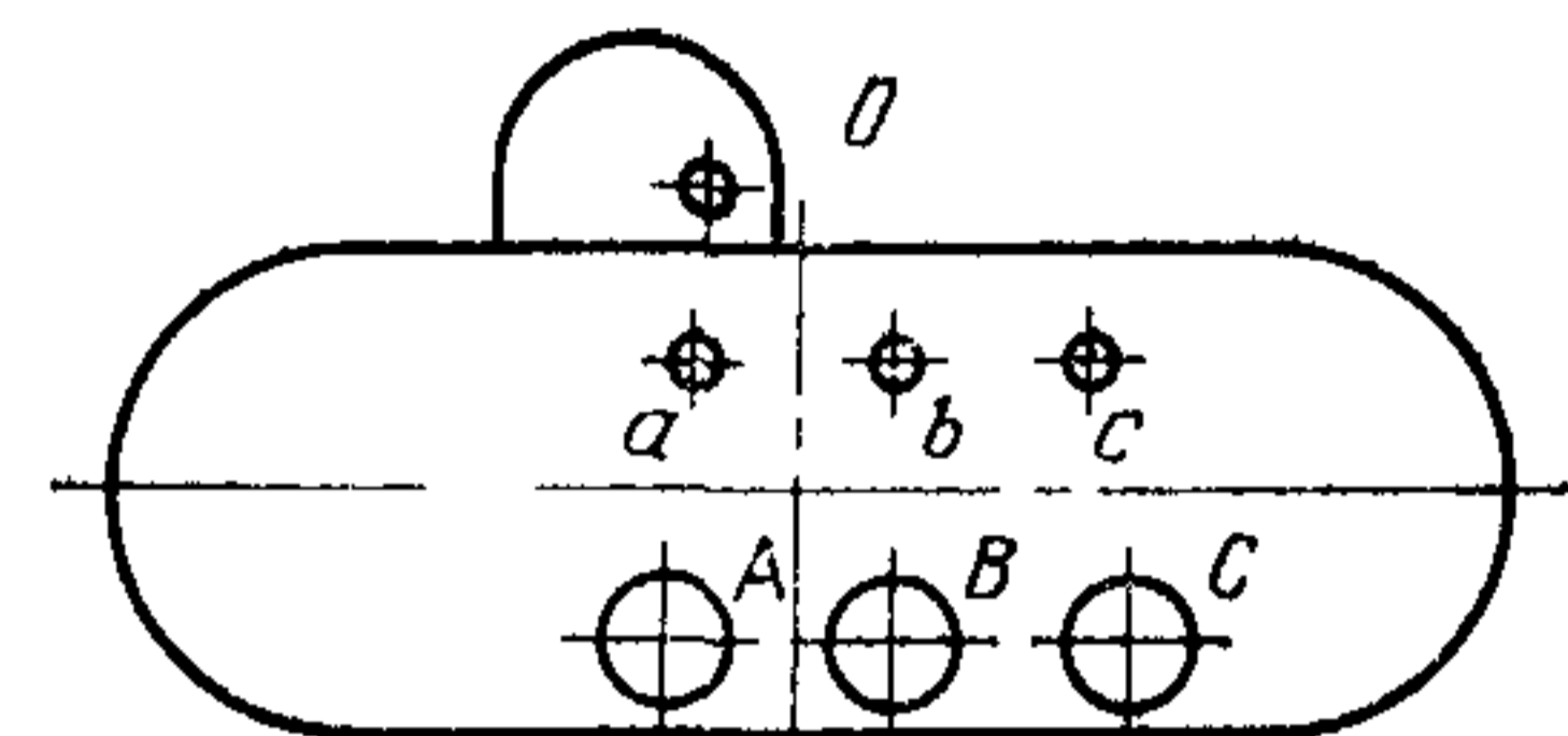
а) класс напряжения 330 кВ
