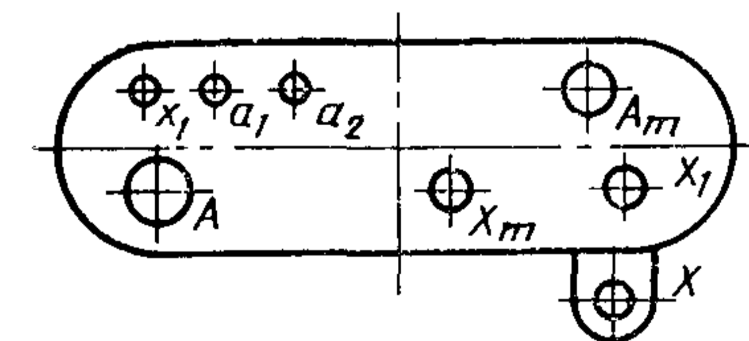
в) автотрансформатор АОДЦТН-333000/750/330
