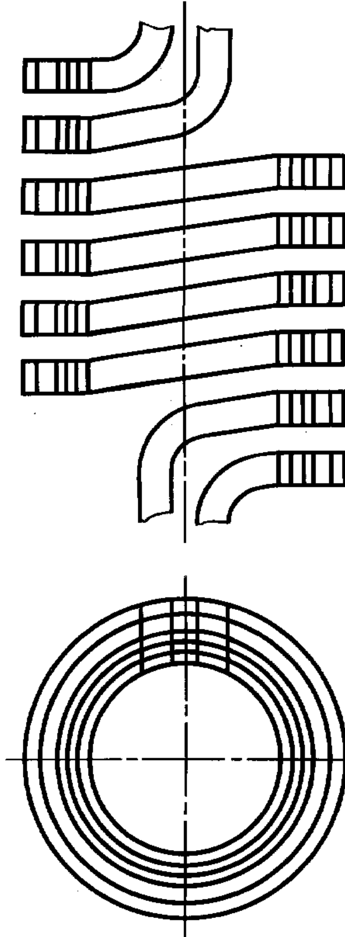
Двухходовая винтовая обмотка трансформатора (к термину 7.2.13)
