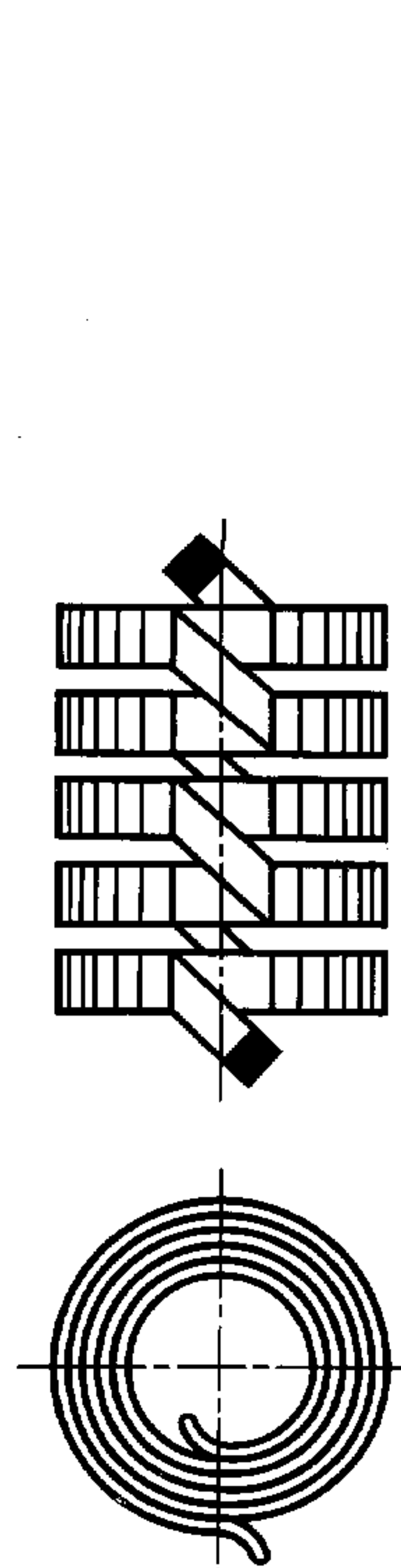
Непрерывная обмотка трансфор- матора (к термину 7.2.8)
