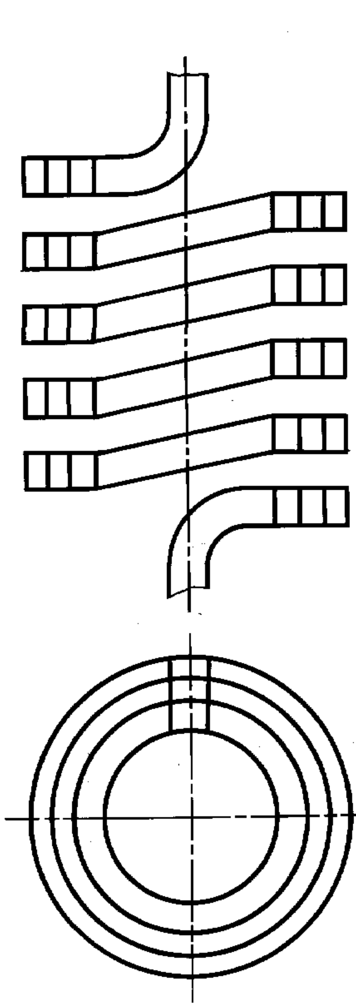
Одноходовая винтовая обмотка трансформатора (к термину 7.2.12)
