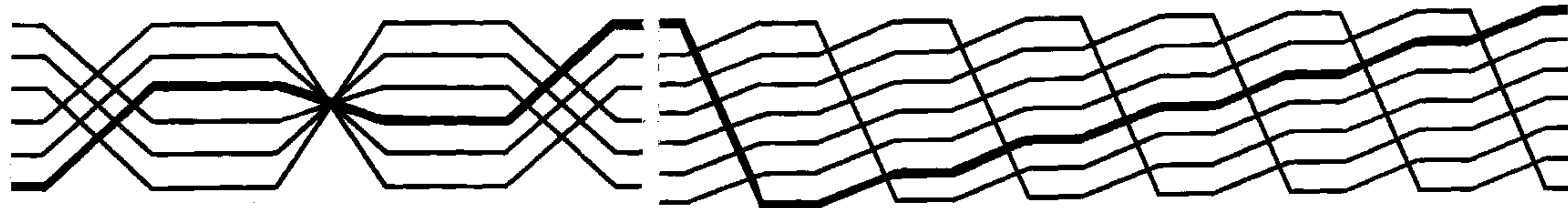
Групповая транспо- зиция Общая транспо- зиция Групповая транспо- зиция
