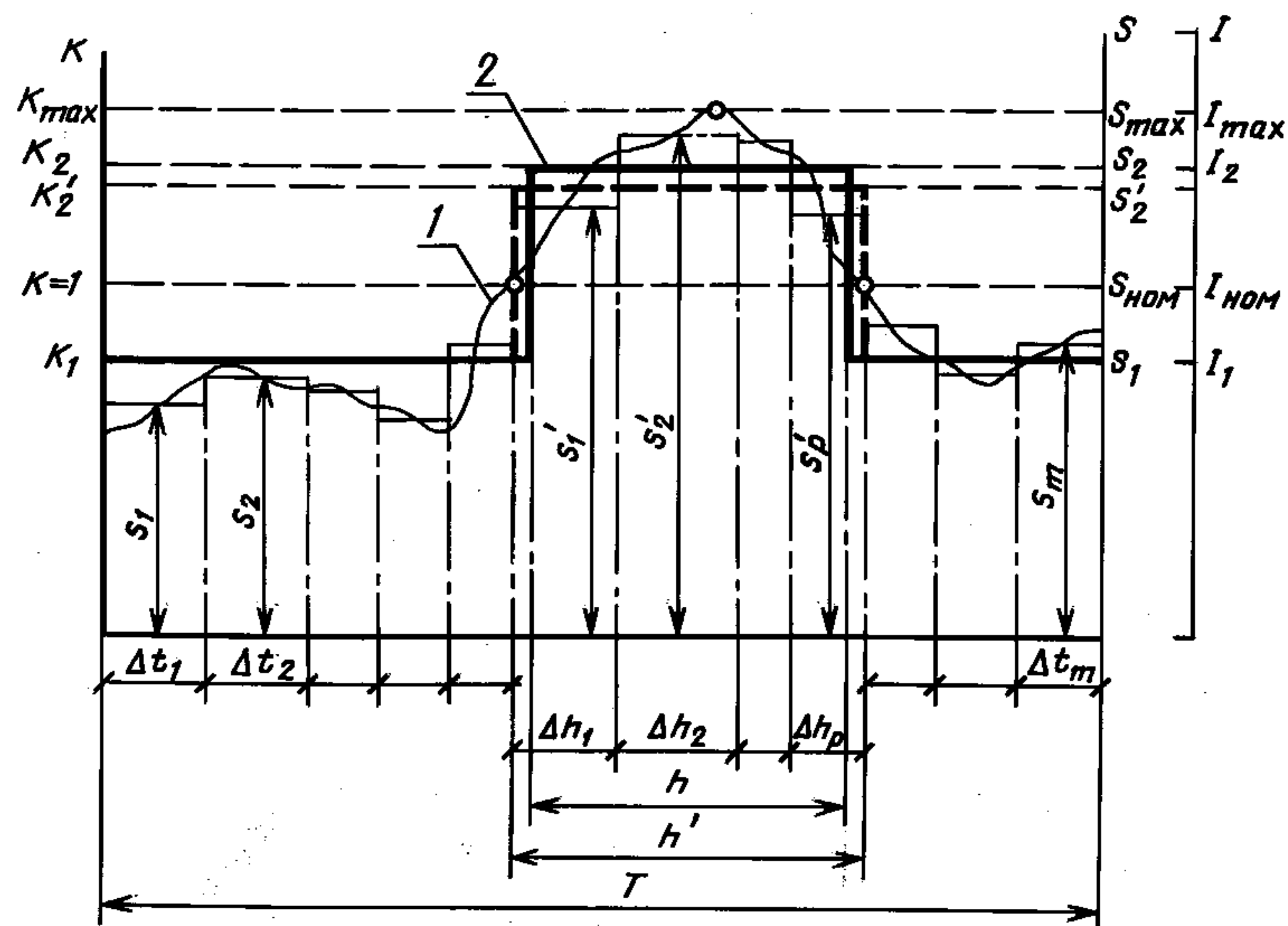
1 — исходный график нагрузки; 2 — двухступенчатый прямоугольный график нагрузки
