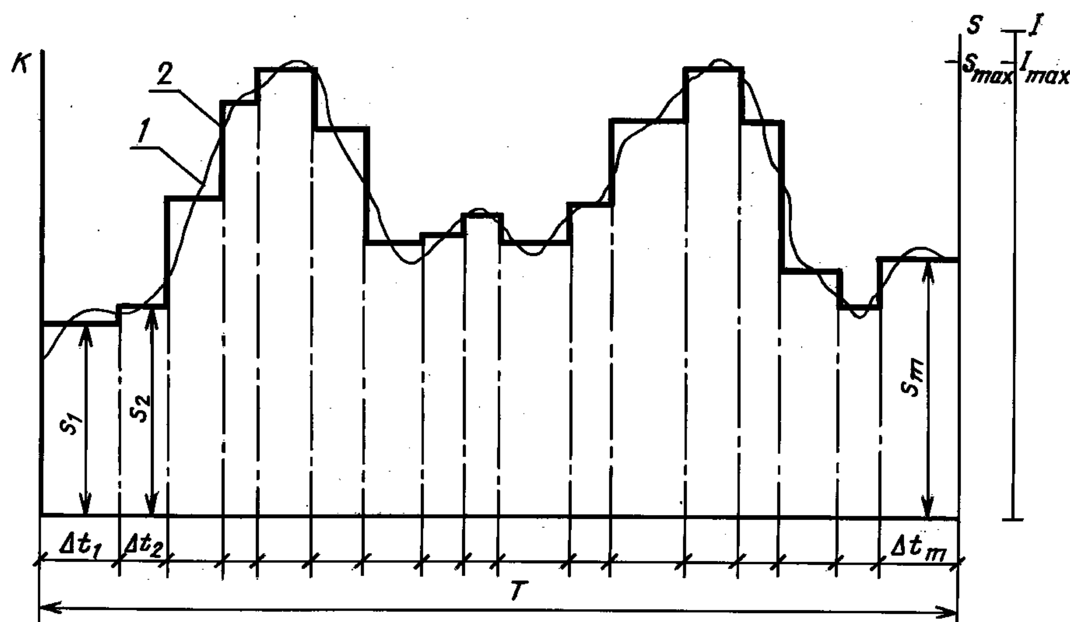
1 — исходный график нагрузки; 2 — эквивалентный прямоугольный график нагрузки
