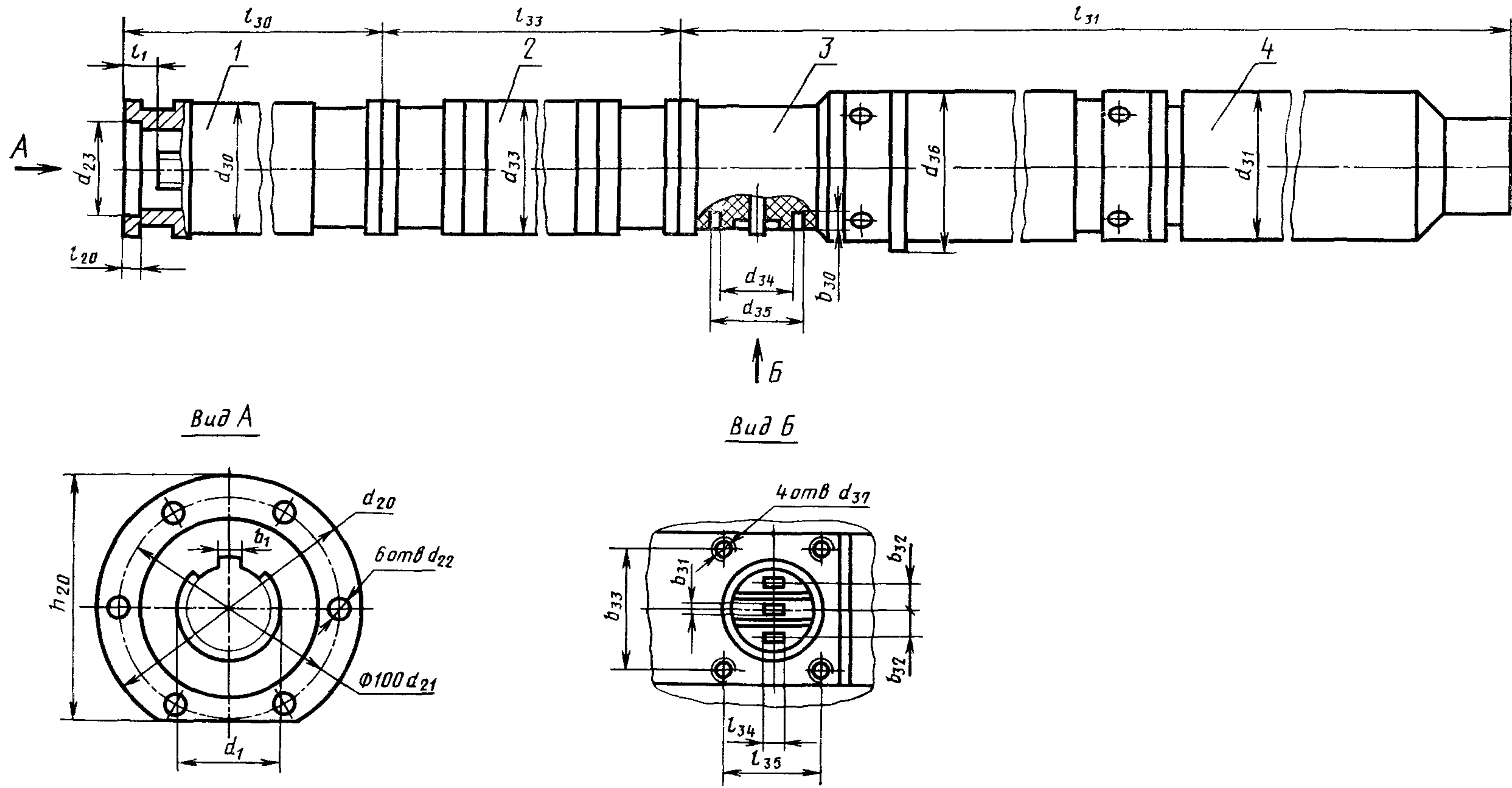
1—прожектор; 2—компенсатор; 3—верхняя секция; 4—нижняя секция
