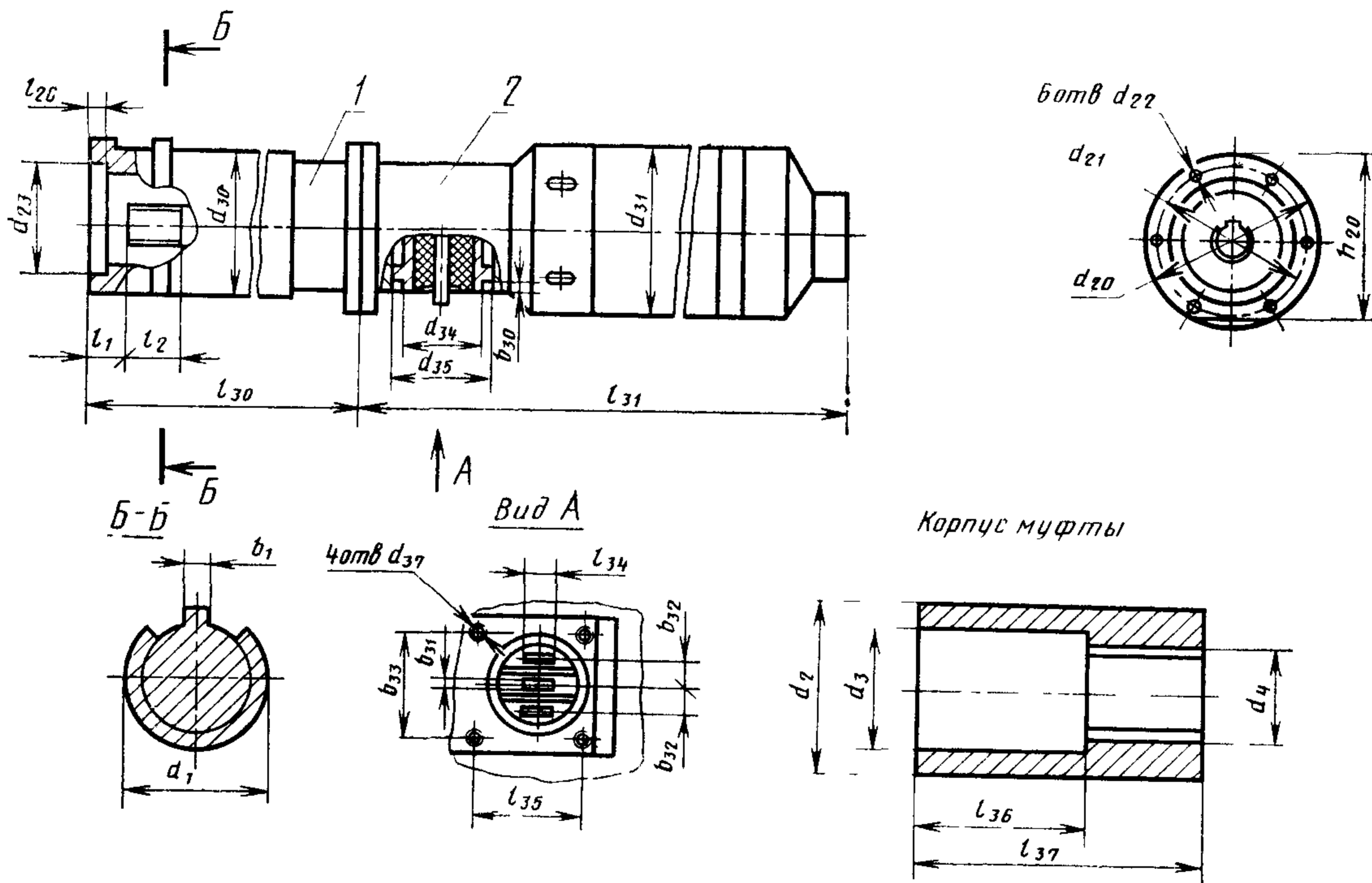
1—протектор, 2—электродвигатель
