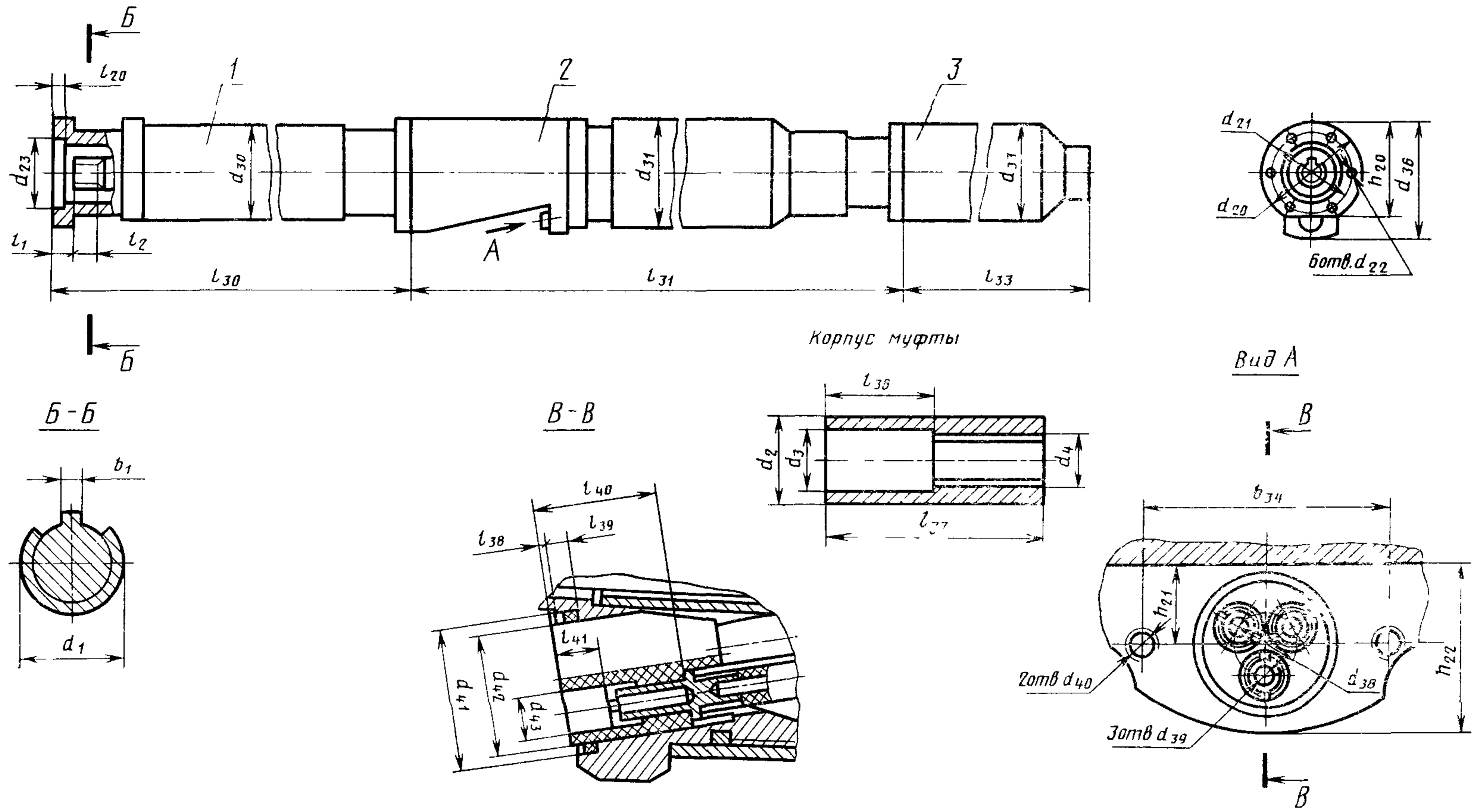
1—протектор; 2—электродвигатель; 3—компенсатор
