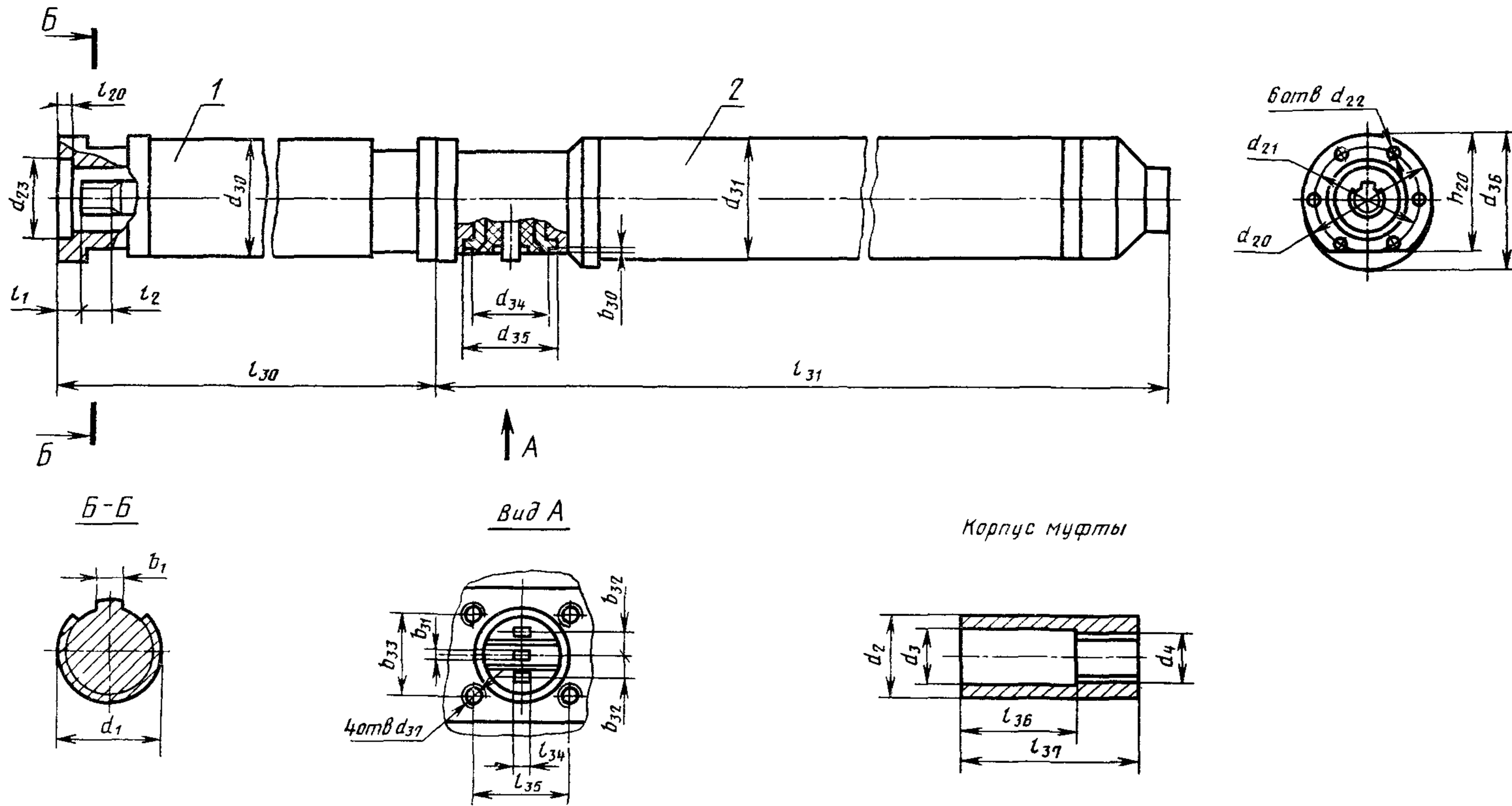
1—протектор; 2—электродвигатель Черт. 12
