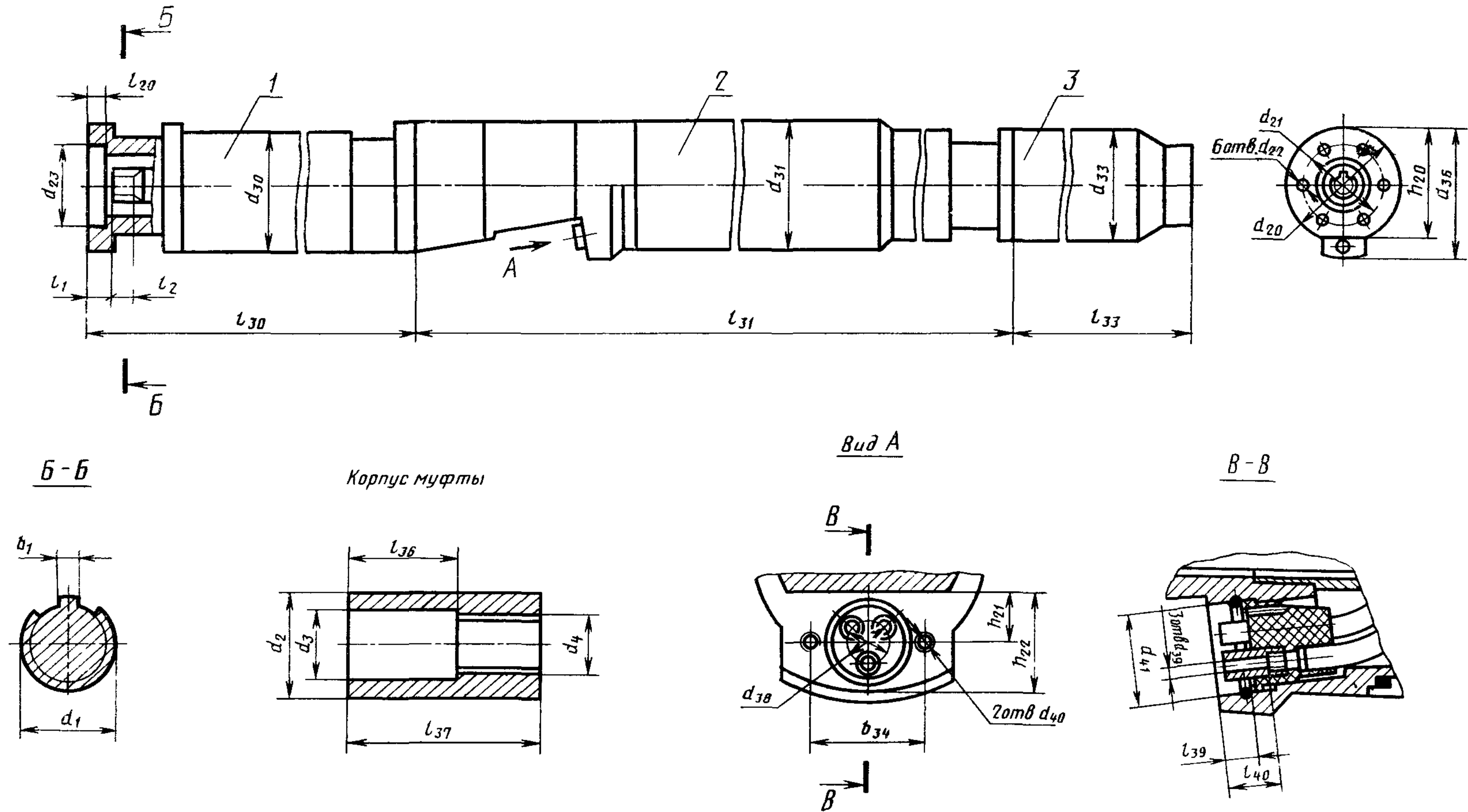
1—протектор, 2—электродвигатель; 3—компенсатор Черт. 13
