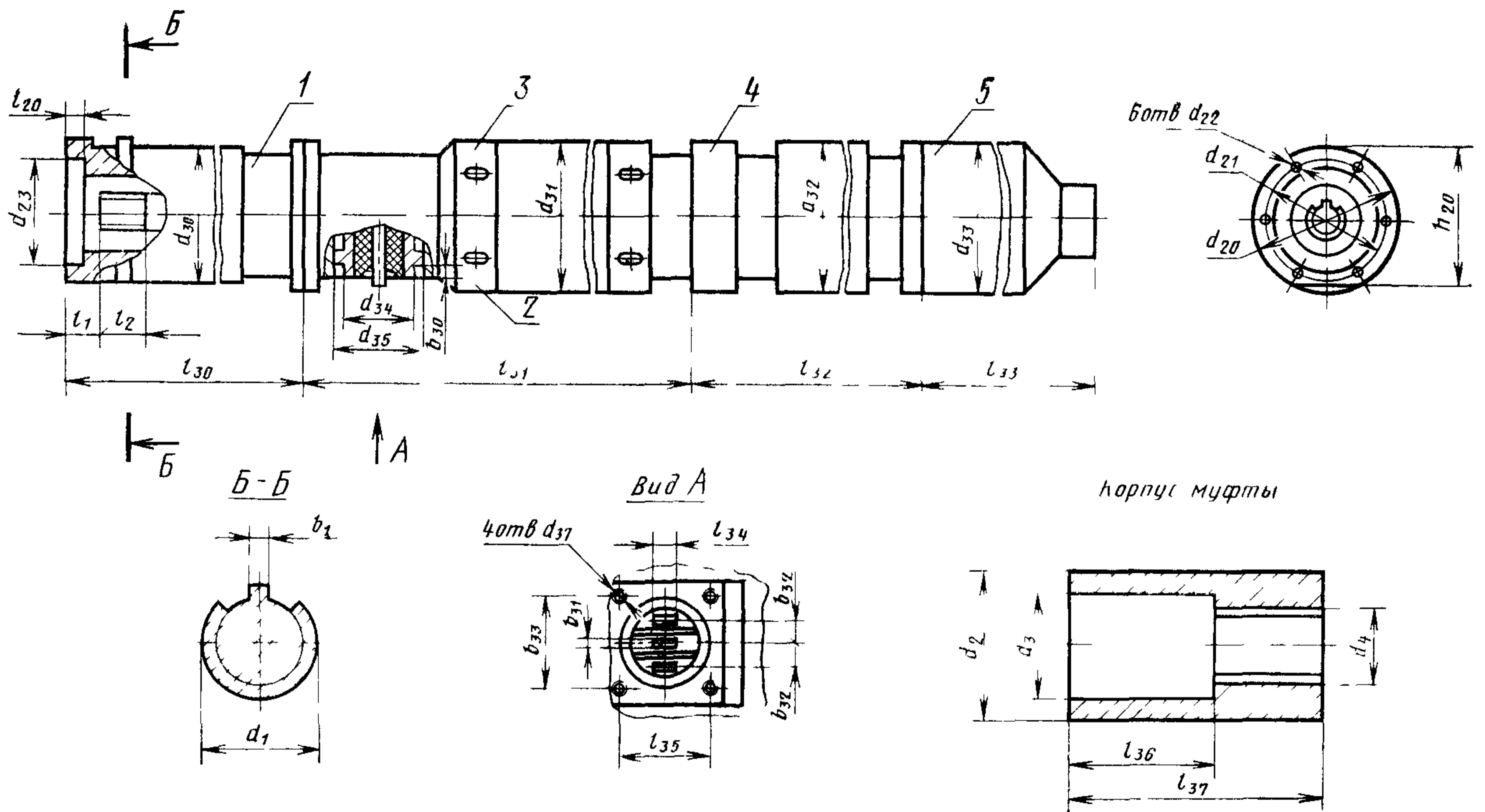
1—проектор 2—электродвигатель 3—верхняя секция; 4—нижняя секция, 5—компенсатор
