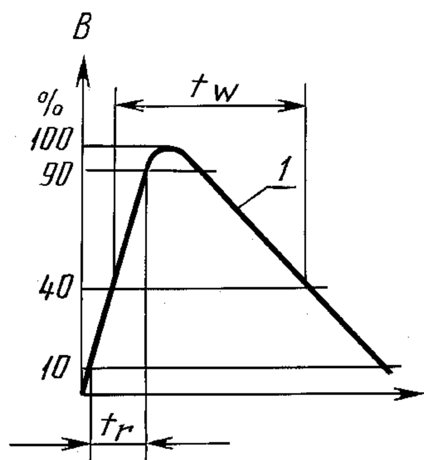
1 — напряжение, В
