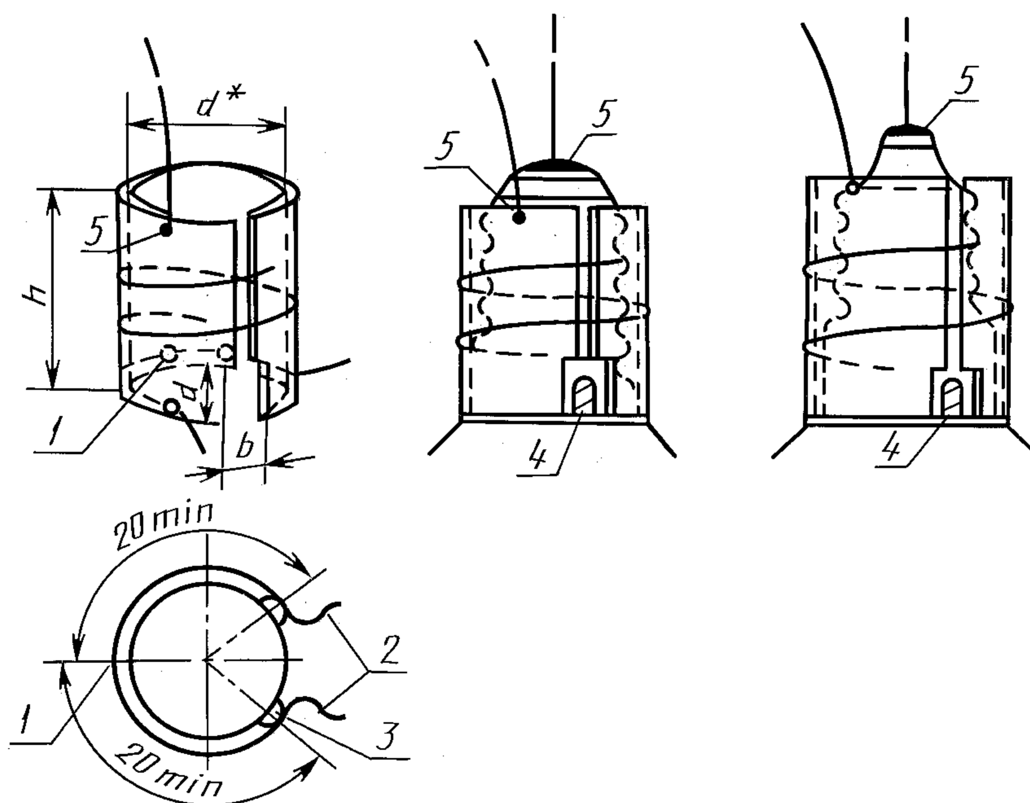
Испытательный патрон для цоколей E14/20 и E14/25 × 17
