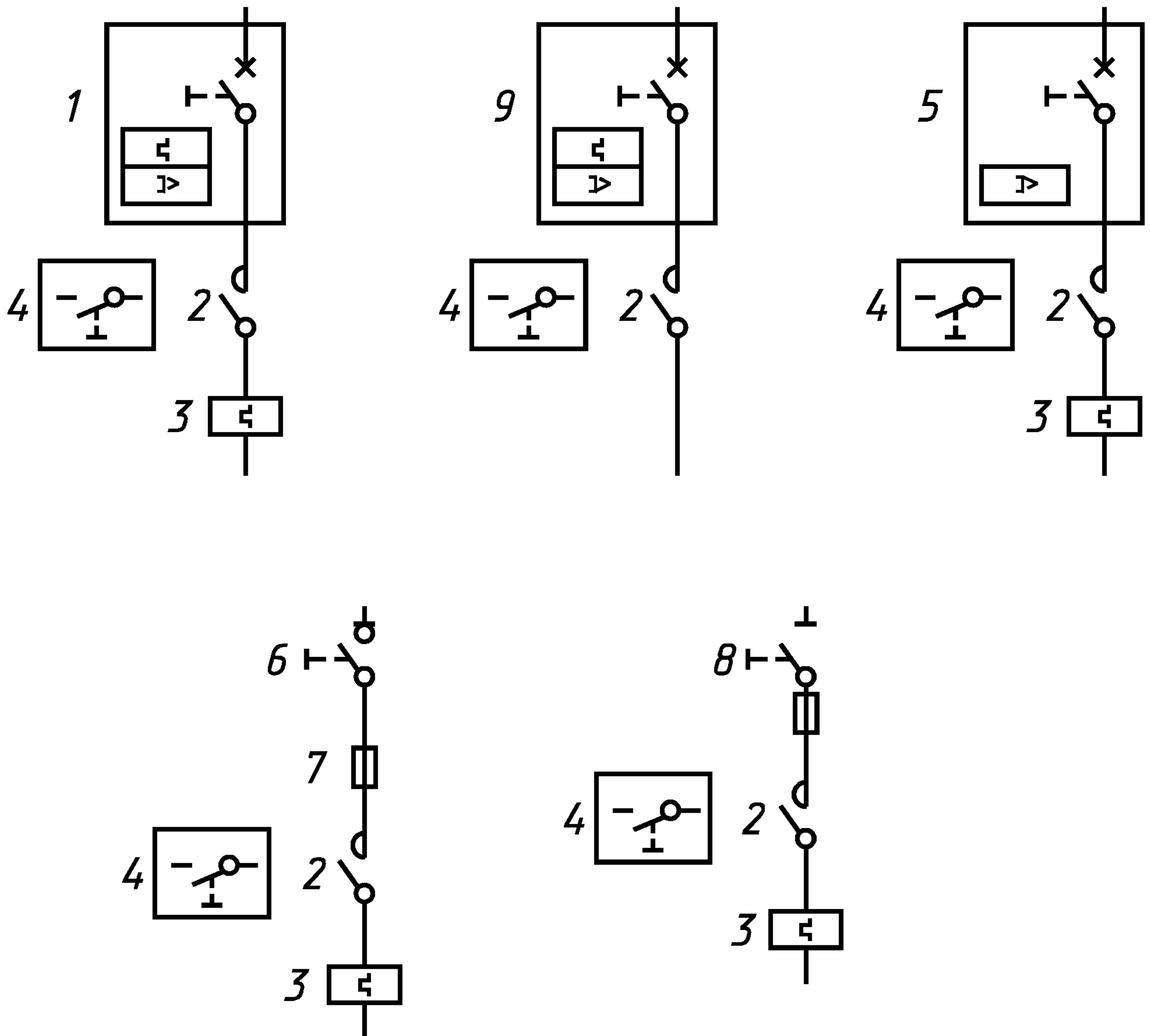
1 — автоматический выключатель; 2 — контактор; 3 — реле перегрузки; 4 — аппарат управления; 5 — автоматический выключатель с электромагнитным расцепителем; 6 — выключатель-разъединитель; 7 — плавкий предохранитель; 8 — разъединитель с плавким предохранителем; 9 — автоматический выключатель с расцепителем перегрузки, соответствующим настоящему стандарту
