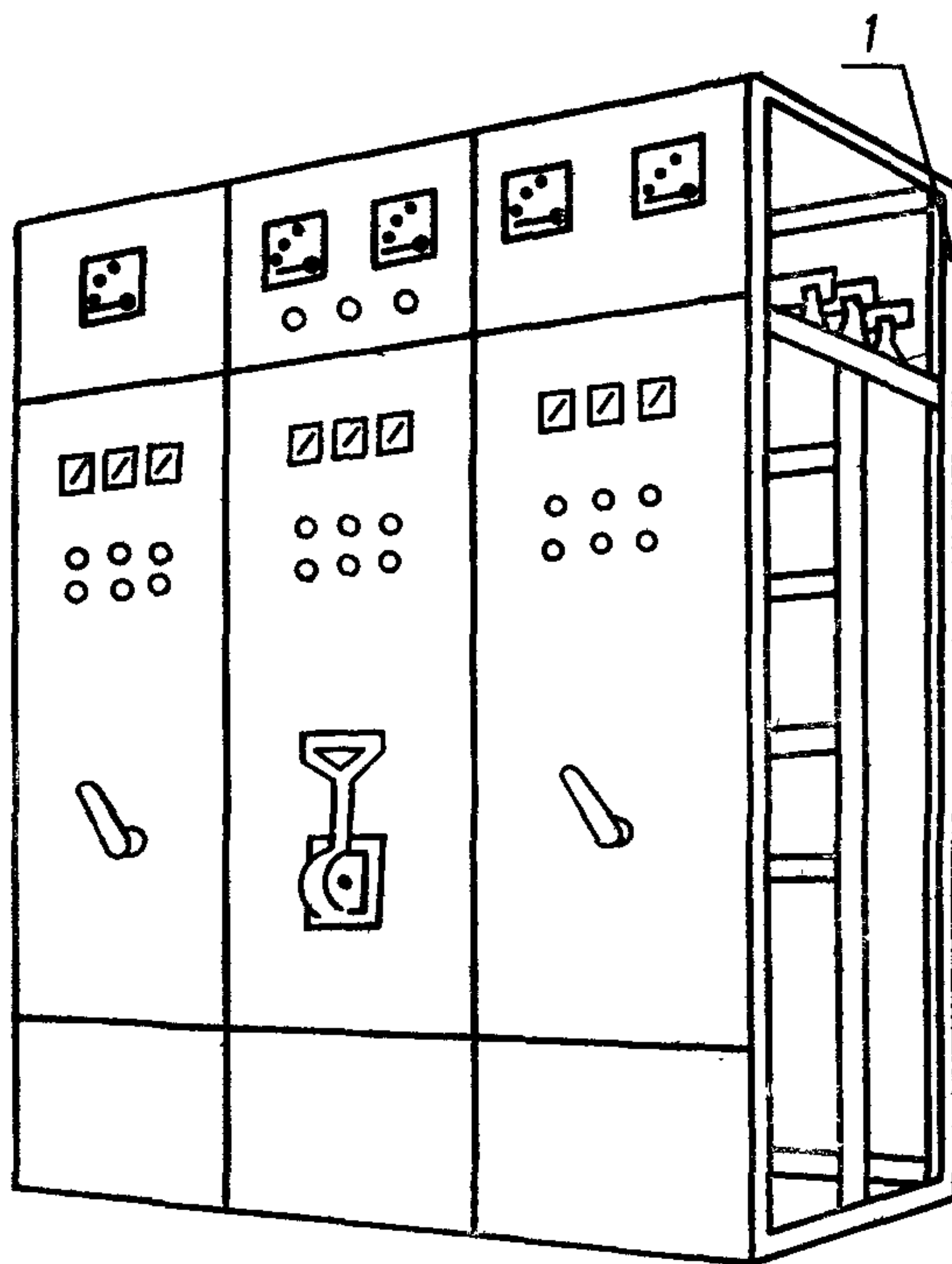
Рисунок С.2 — НКУ открытого типа, защищенное спереди
