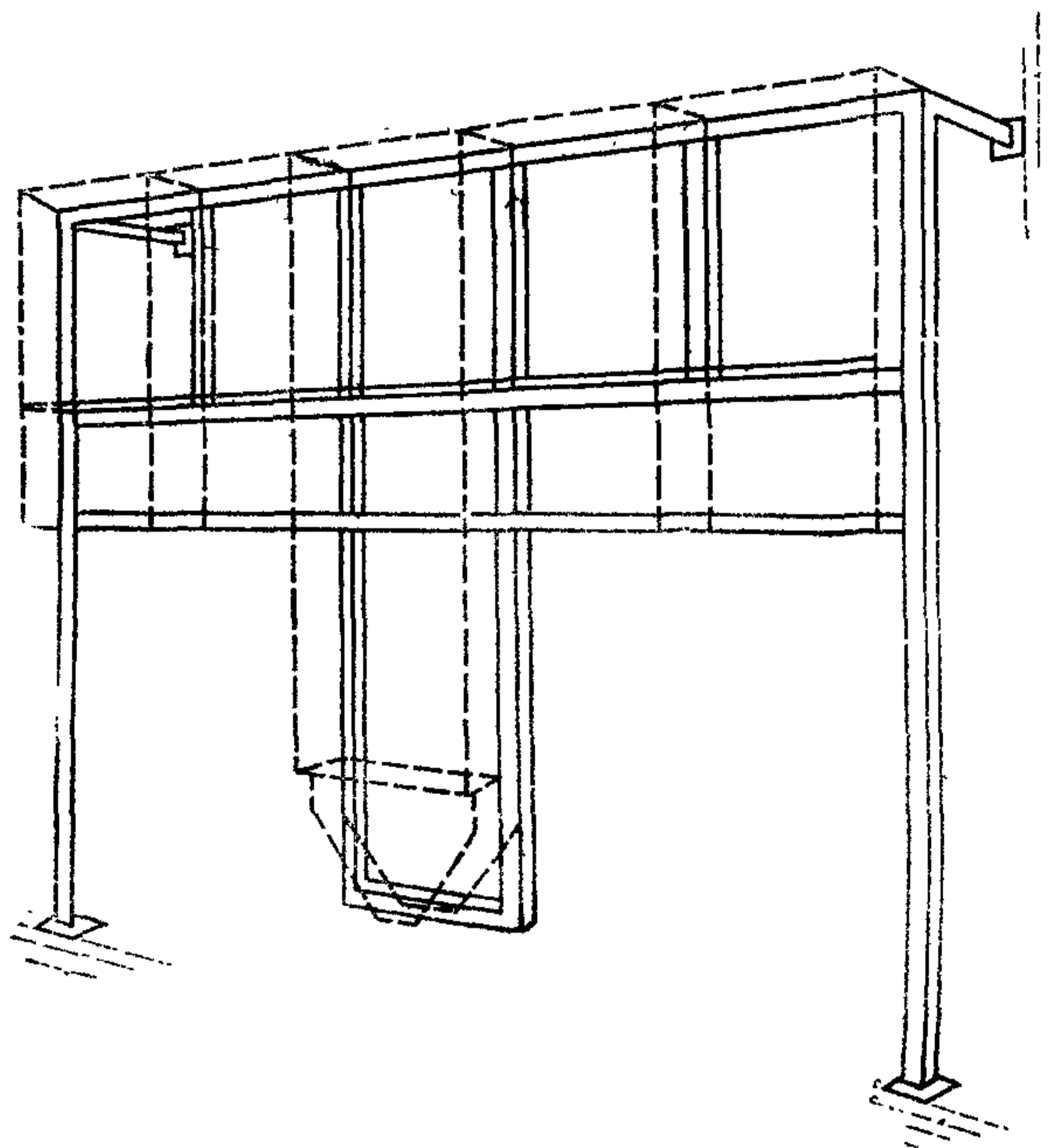
Рисунок С.8 — Монтажная конструкция
