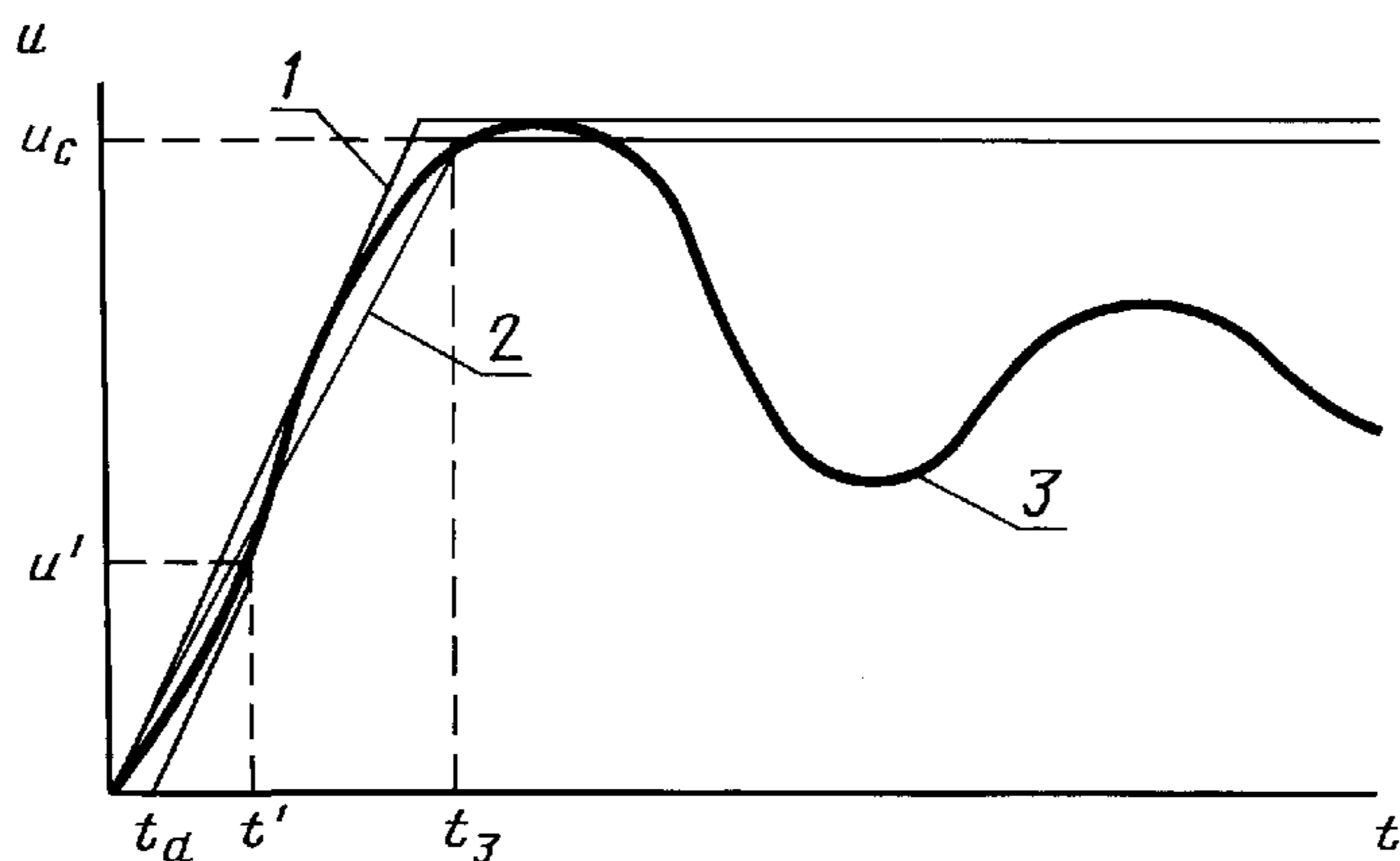
Построение огибающей ПВН, определяемого двумя параметрами
