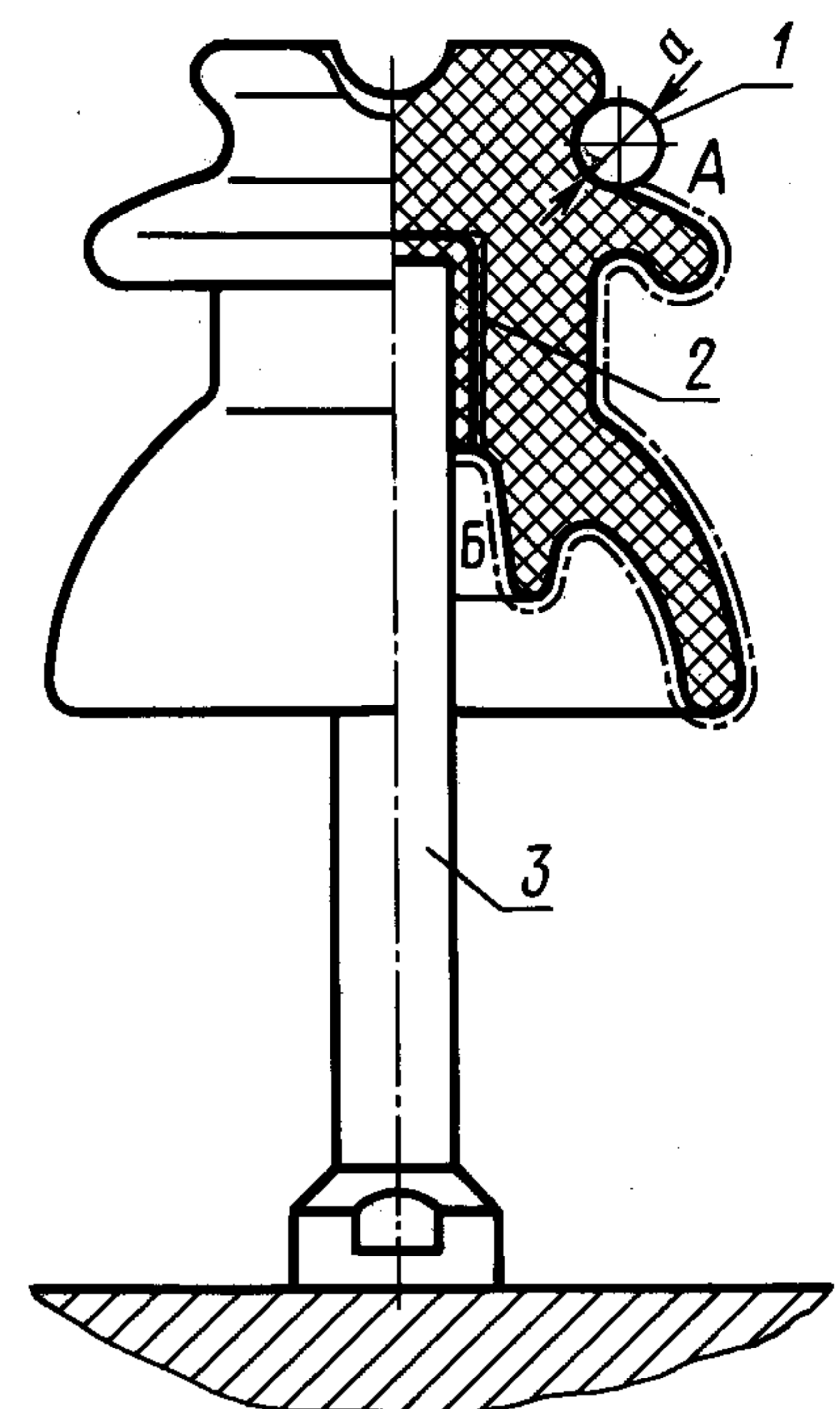
1 — провод; 2 — уплотнитель; 3 — штырь
