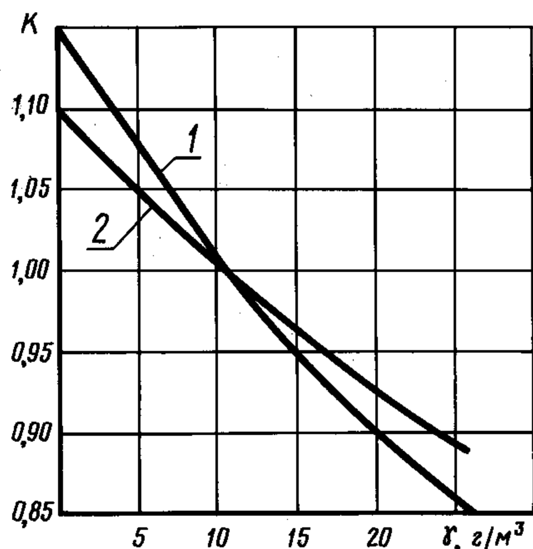
Изменение коэффициента K в зависимости от абсолютной влажности воздуха
