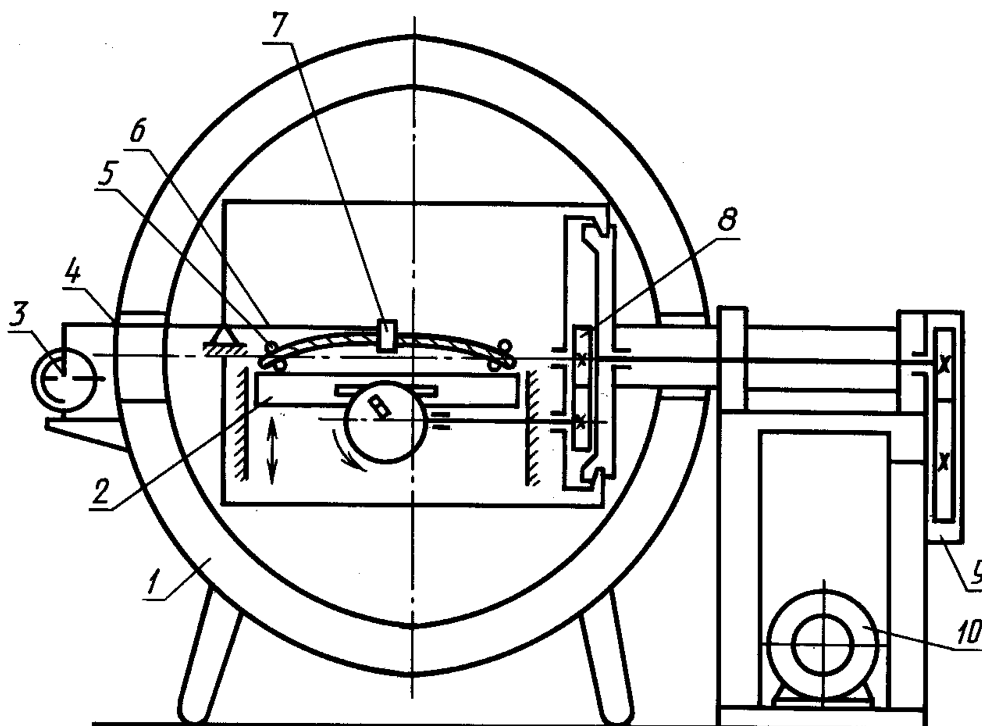
Схема стенда для определения усилия изгиба кабеля
