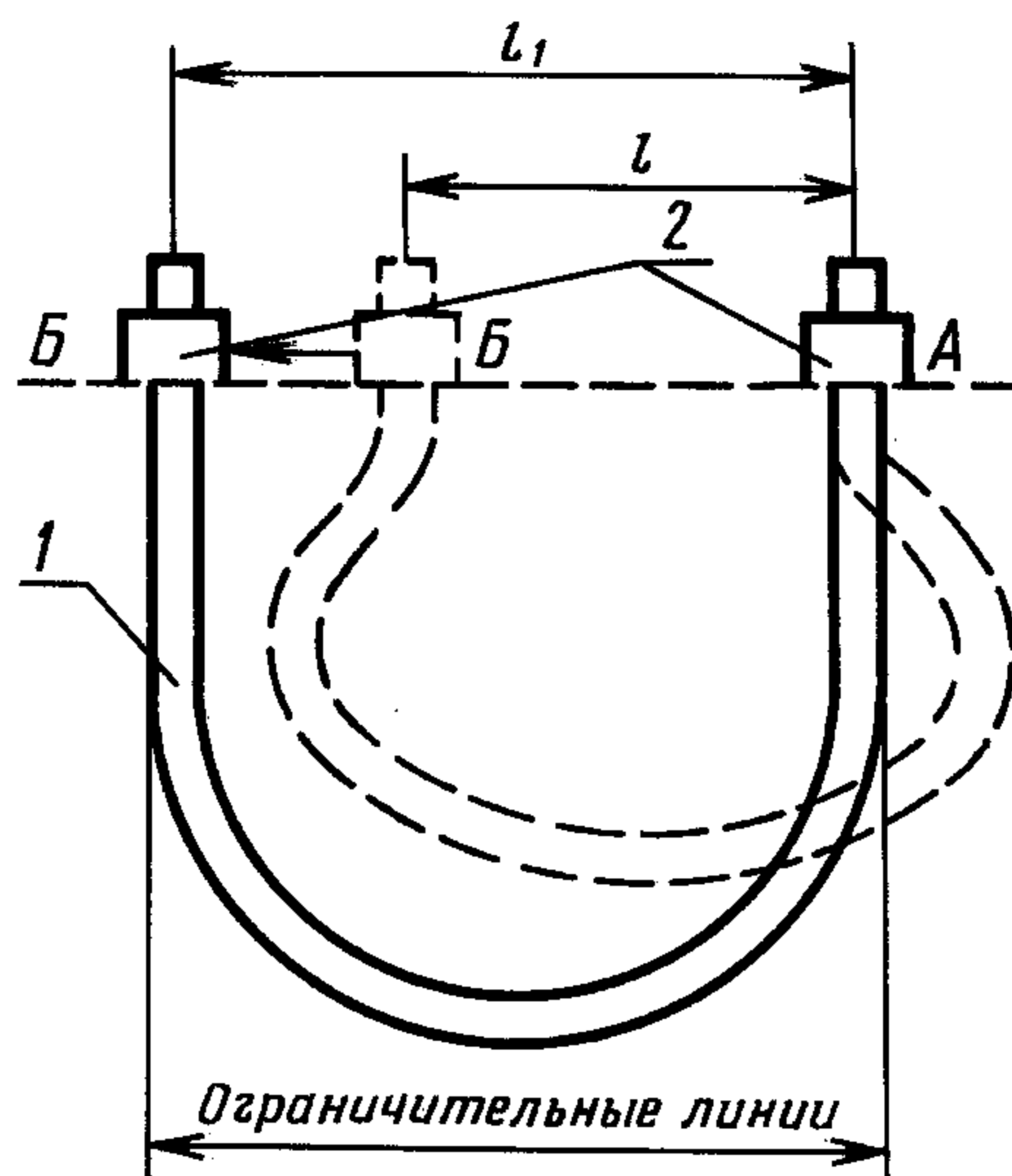
1 — испытуемый образец; 2 — зажимы
