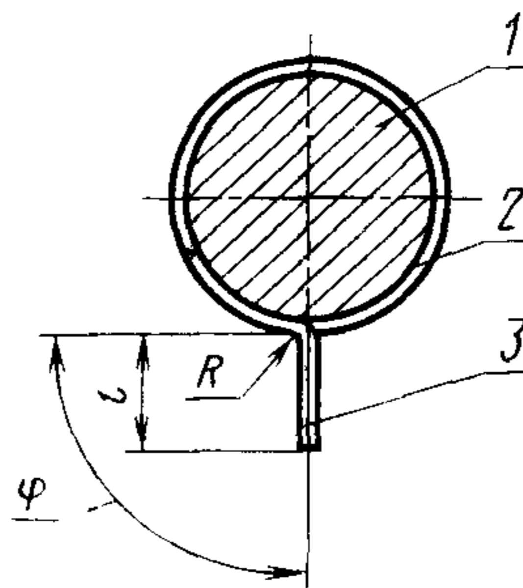
1—оправка, 2—провод; 3—стрелка
