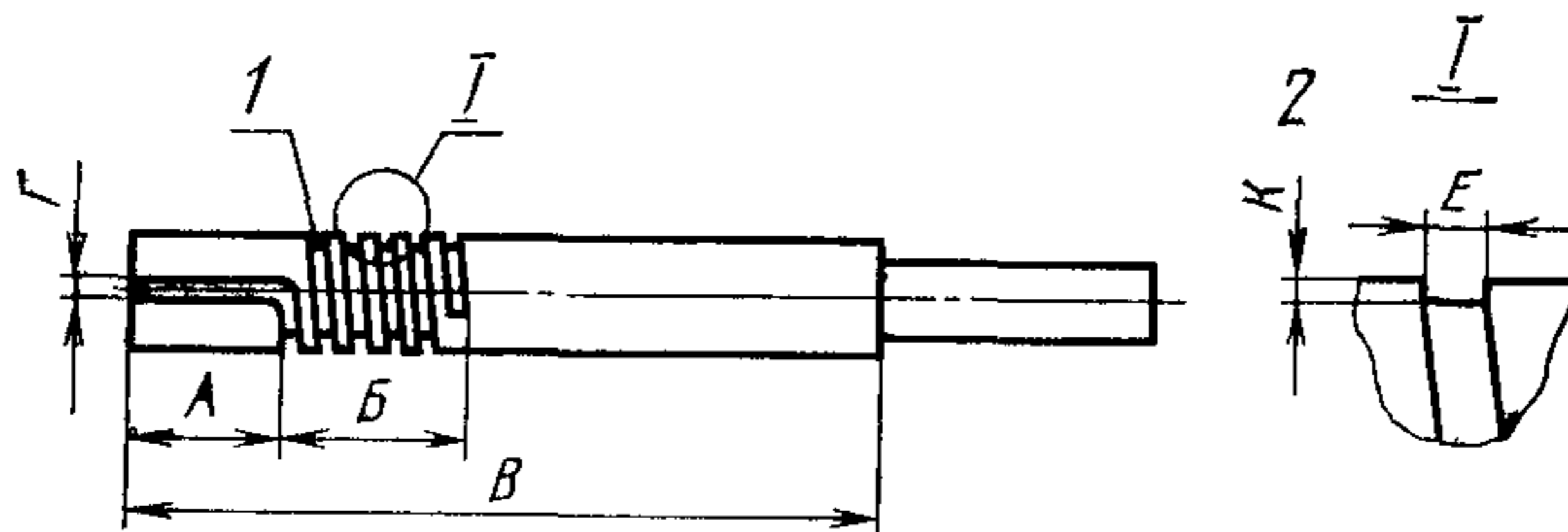
1—винтовая канавка; 2—канавка в увеличенном виде
