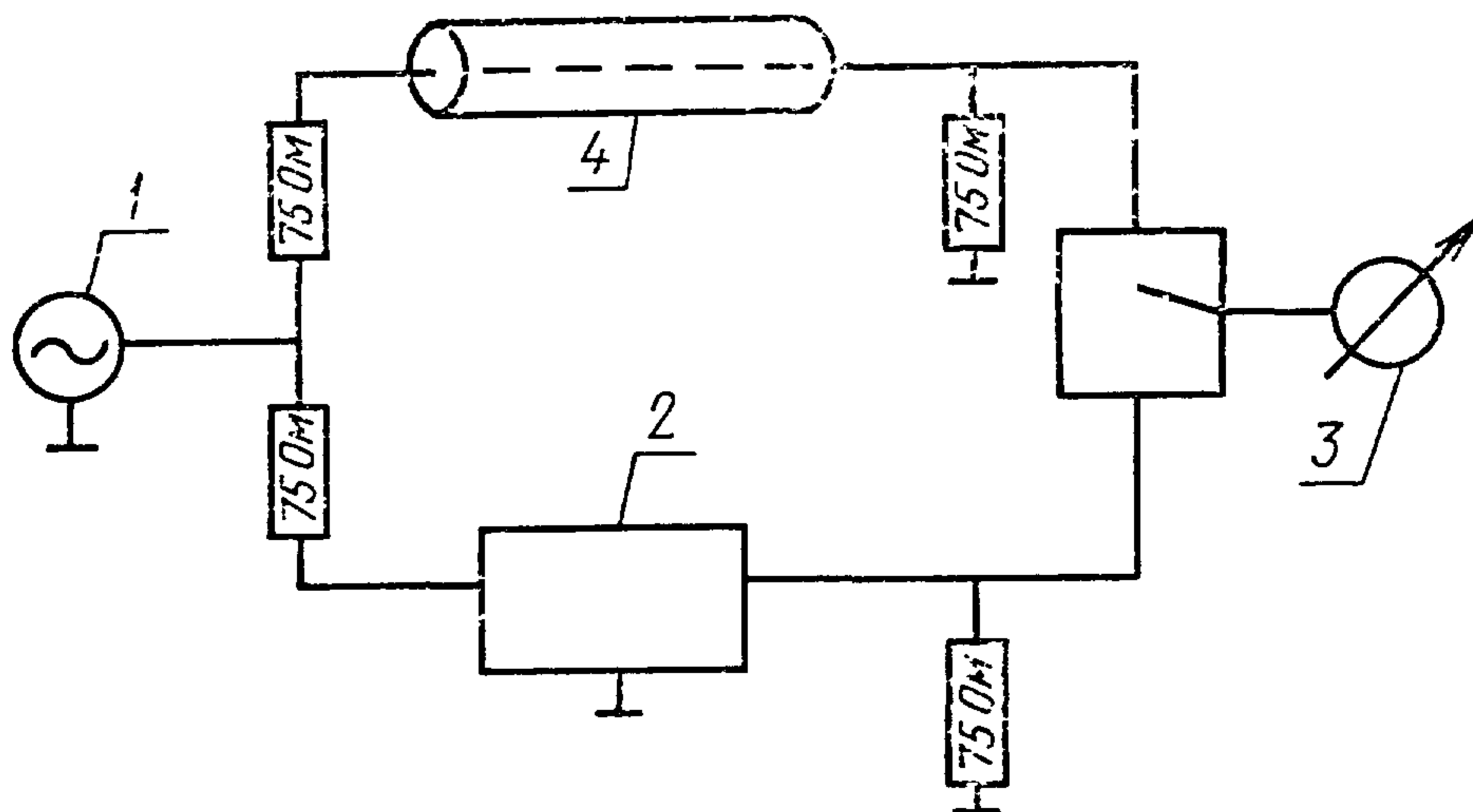
1—генератор; 2—магазин затухания; 3—индикатор; 4—измеряемая коаксиальная линия
