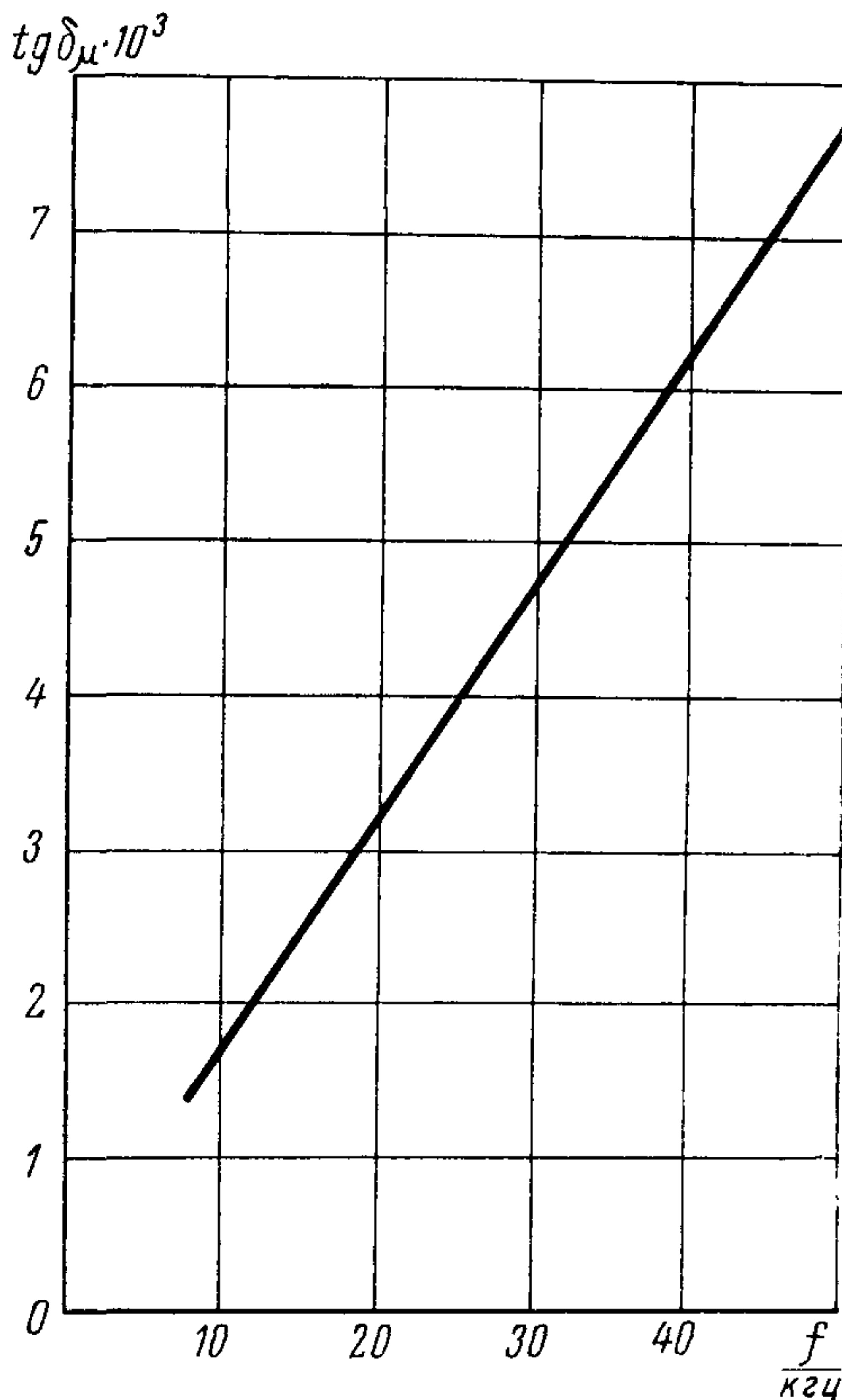
График зависимости тангенса угла потерь материала от частоты
