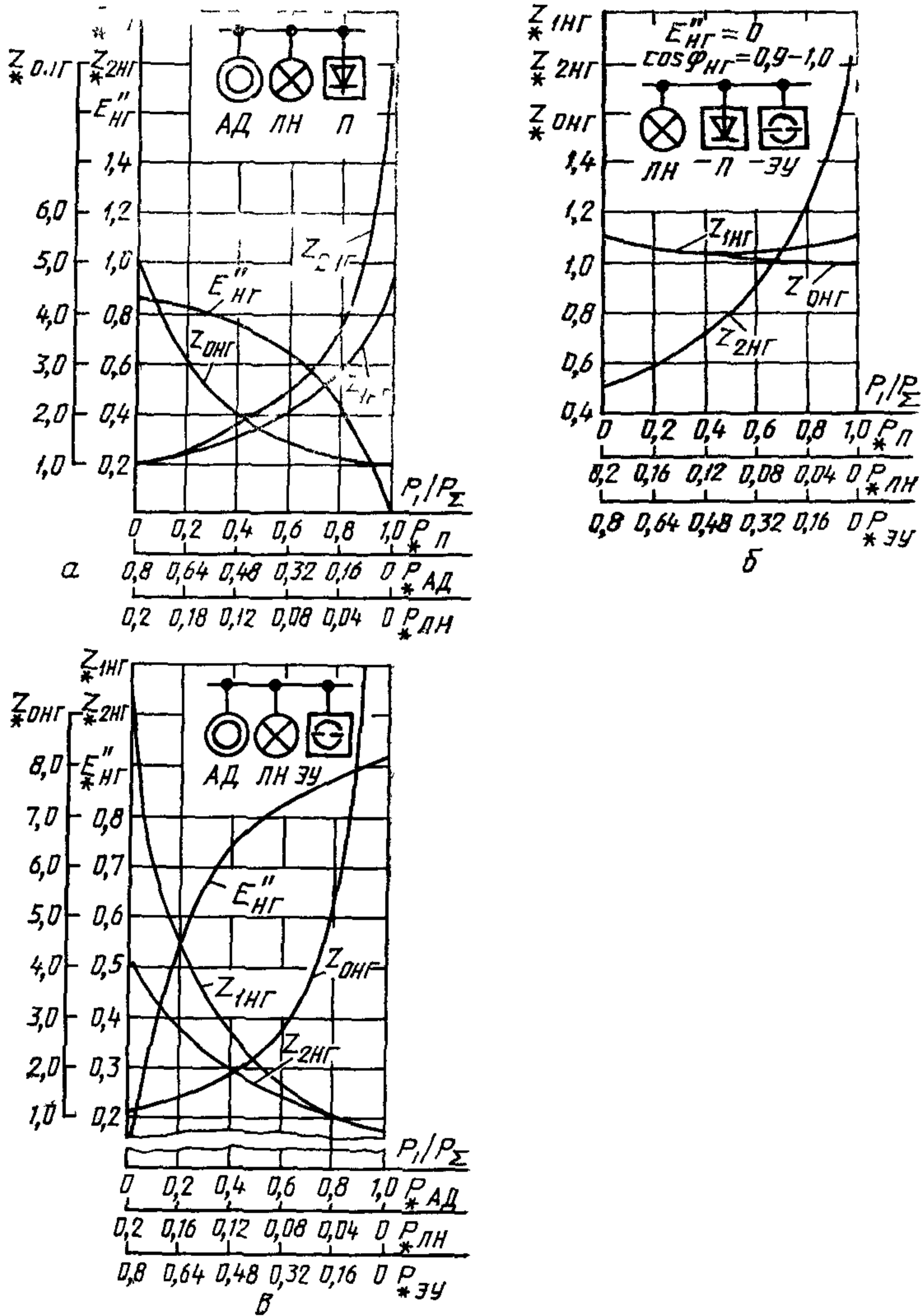
Зависимость параметров комплексной нагрузки Z_{1НГ} , Z_{2НГ} , Z_{0НГ} , E_{НГ}'' от ее состава
