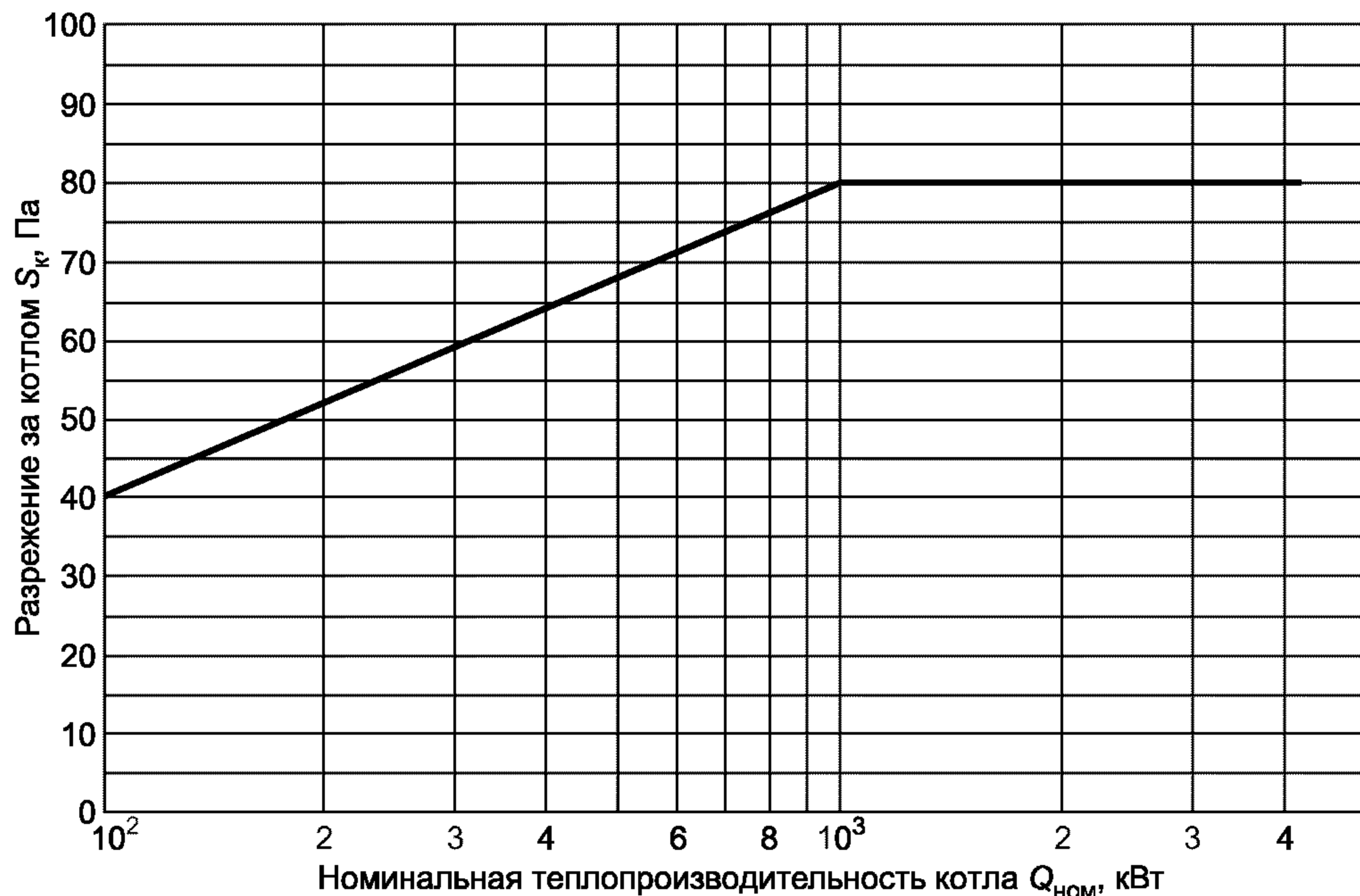
Рисунок 2 — Максимальное разрежение за котлом на естественной тяге
