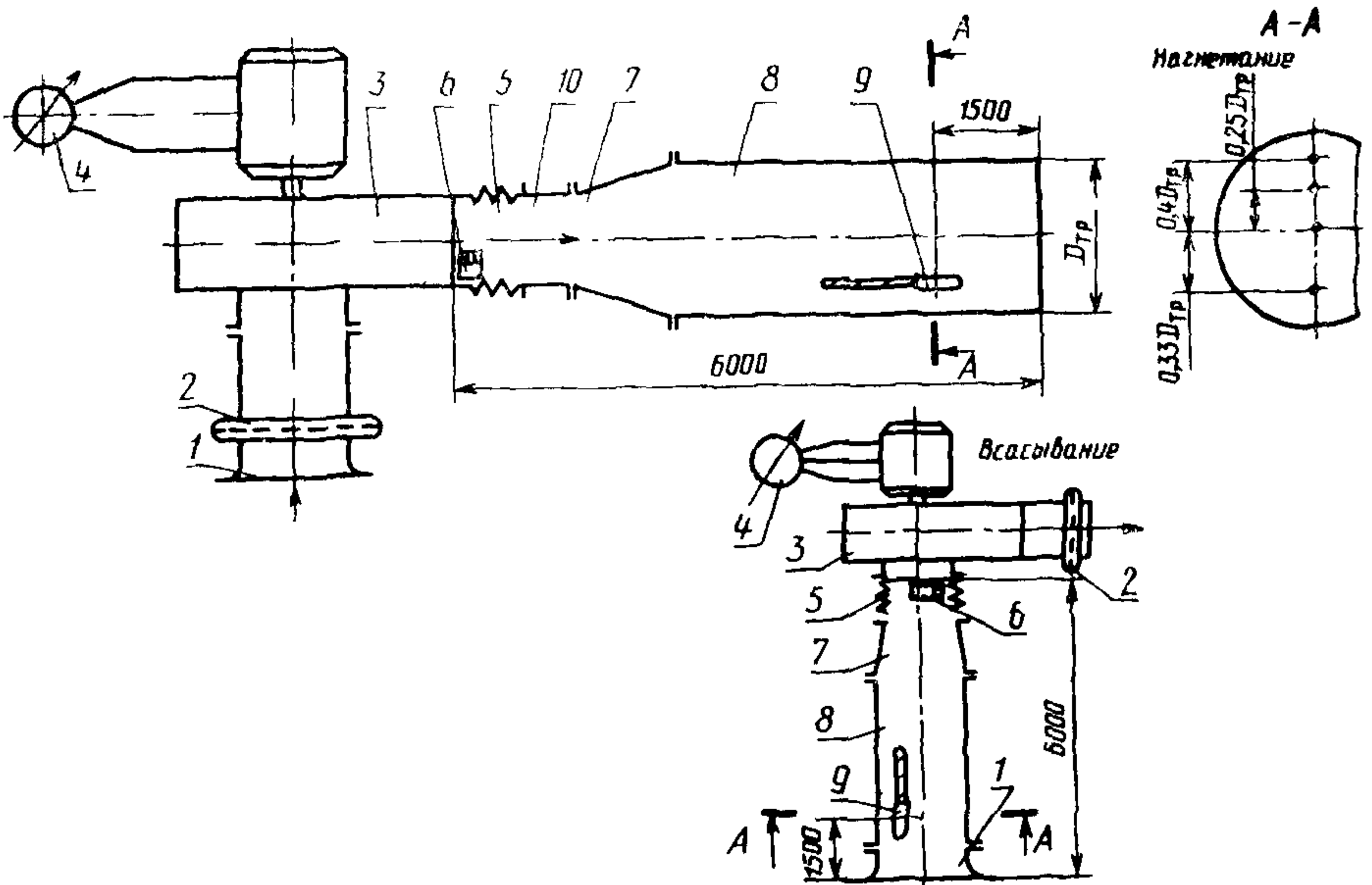
Схема стенда для определения акустических характеристик ТДМ по методу II. Центробежная машина
